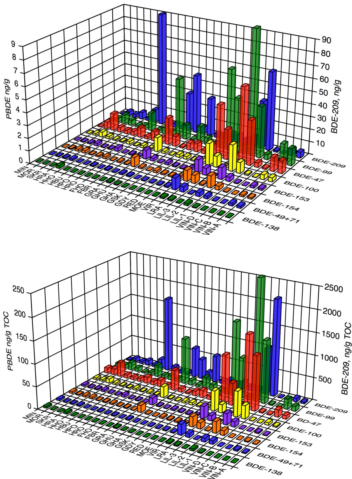
Figur 3. Konsentrasjoner av utvalgte PBDE-kongenerer i overflatesjikt ved de enkelte stasjoner. Konsentrasjoner under deteksjonsgrensen er satt lik halve denne. Øvre figur viser konsentrasjonene på tørrvektsbasis, nedre figur viser dem justert for innholdet av organisk karbon (ng/g TOC). Merk: ulik skala for BDE-209 (høyre verdiakse) og de øvrige kongenerer (venstre verdiakse). De enkelte stasjonene er identifisert ved stasjonskoden.
