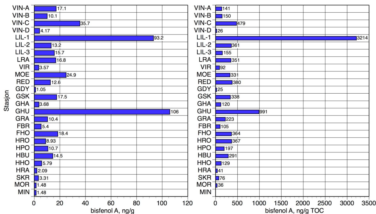
Figur 8. Konsentrasjoner av bisfenol A i overflatesjikt ved ulike stasjoner. Venstre figur viser konsentrasjonen på tørrvektsbasis (ng/g), høyre figur viser konsentrasjonen normalisert mot prøvens innhold av totalt organisk karbon (ng/g TOC). Konsentrasjoner under deteksjonsgrensen er satt lik halve denne. De enkelte stasjonene er identifisert ved stasjonskoden.
