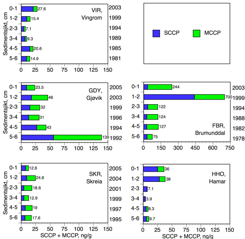
Figur 13. Konsentrasjoner av klorerte parafiner (kortkjedede: SCCP, mellomkjedede: MCCP) i ulike sedimentsjikt ved fem stasjoner. Årstall for dateringen av sedimentsjiktet er gitt langs høyre akse (beregnet for midtpunkt for sjiktet). De enkelte stasjonene er identifisert ved stasjonskoden.
