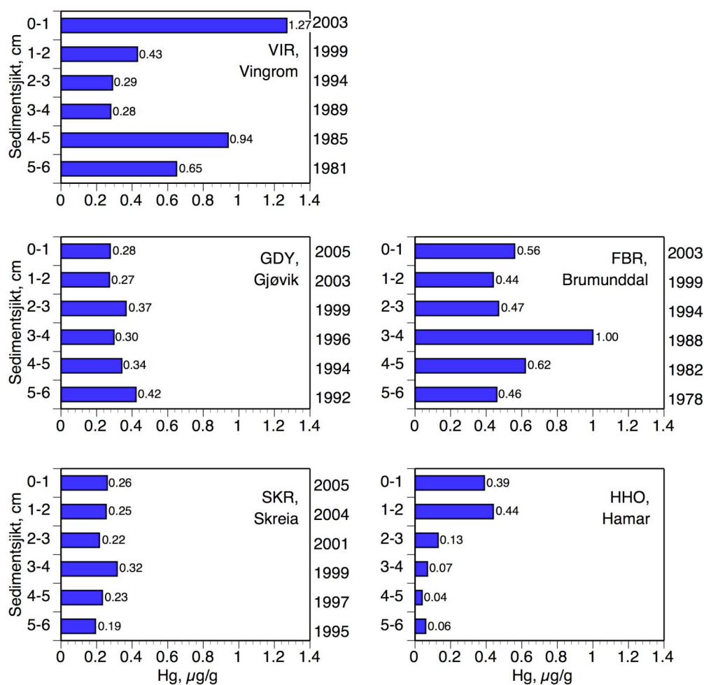
Figur 17. Konsentrasjoner av kvikksølv (Hg) i ulike sedimentsjikt ved fem stasjoner. Årstall for datering av sedimentsjiktet er gitt langs høyre akse (beregnet for midtpunkt av sjiktet). De enkelte stasjonene er identifisert ved stasjonskoden.
