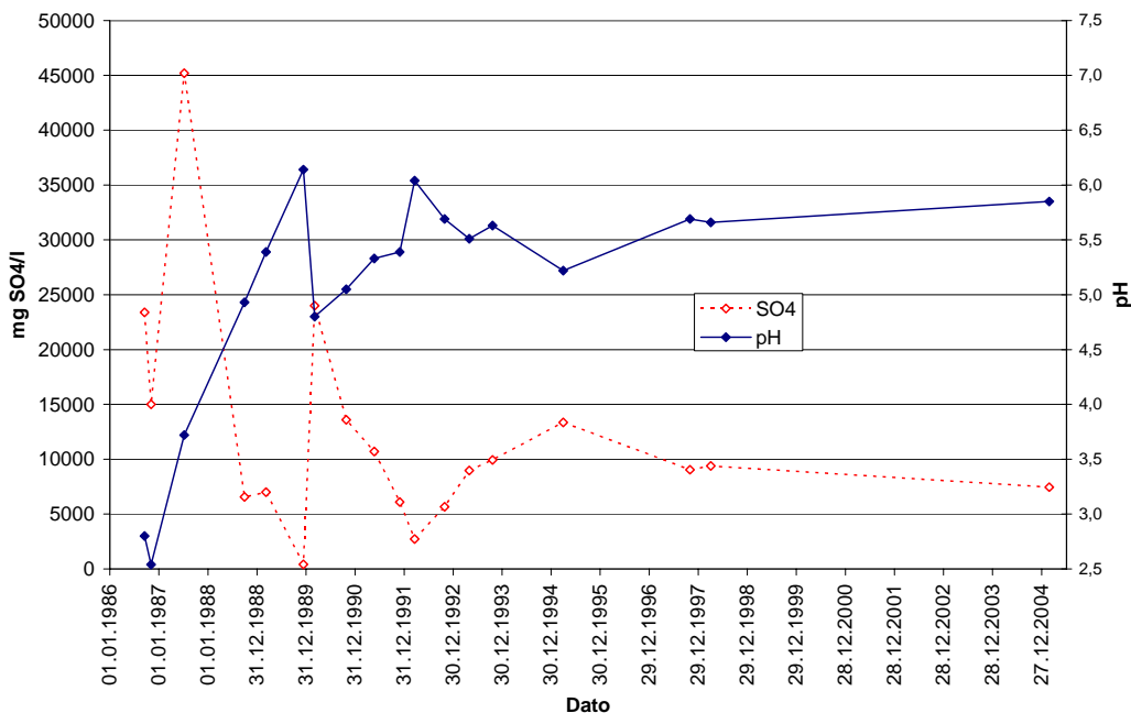
Figur 20. pH- og sulfatobservasjoner ved nivå 380 i perioden 1992-2005.
