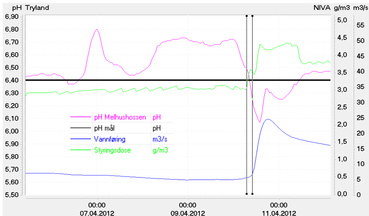
Figur 6. Vannføring og styringsdose ved Tryland doseringsanlegg sammen med pH ved Melhushossen og pH-mål for elva i april 2012. Høyere dosering ble iverksatt kun 3 timer før flommen satte i gang, (markert med to vertikale linjer).
