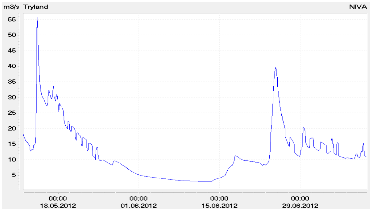
Figur 3. Vannføringen ved Tryland doseringsanlegg fra midt i mai og ut juni 2012. Det ble registrert unøyaktig vannføring. Årsaken er ikke klarlagt.
