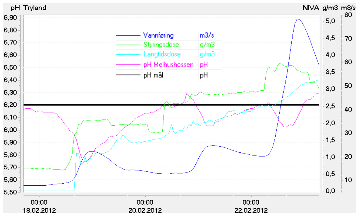
Figur 5. Vannføring, styringsdose og langtidsdose ved Tryland doseringsanlegg sammen med pH ved Melhushossen og pH-mål for elva i februar 2012. Dosene som ble tilført elva i tre fortløpende flommer ble lavere enn styringssignalet skulle tilsi.. Resultatet ble for surt vann i elva.
