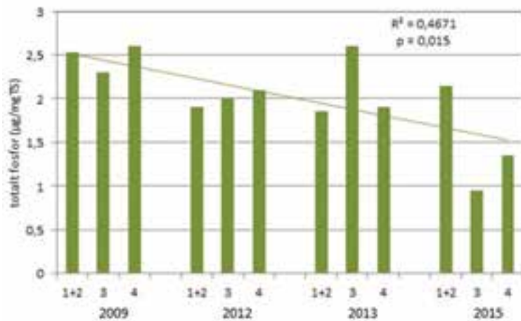
Figur 11. Endringer i fosfor i sedimentet i perioden 2009-2015. Data fra 2009 er hentet fra Molversmyr (2010), mens data fra 2011-2013 er fra Johnsen (2014).
