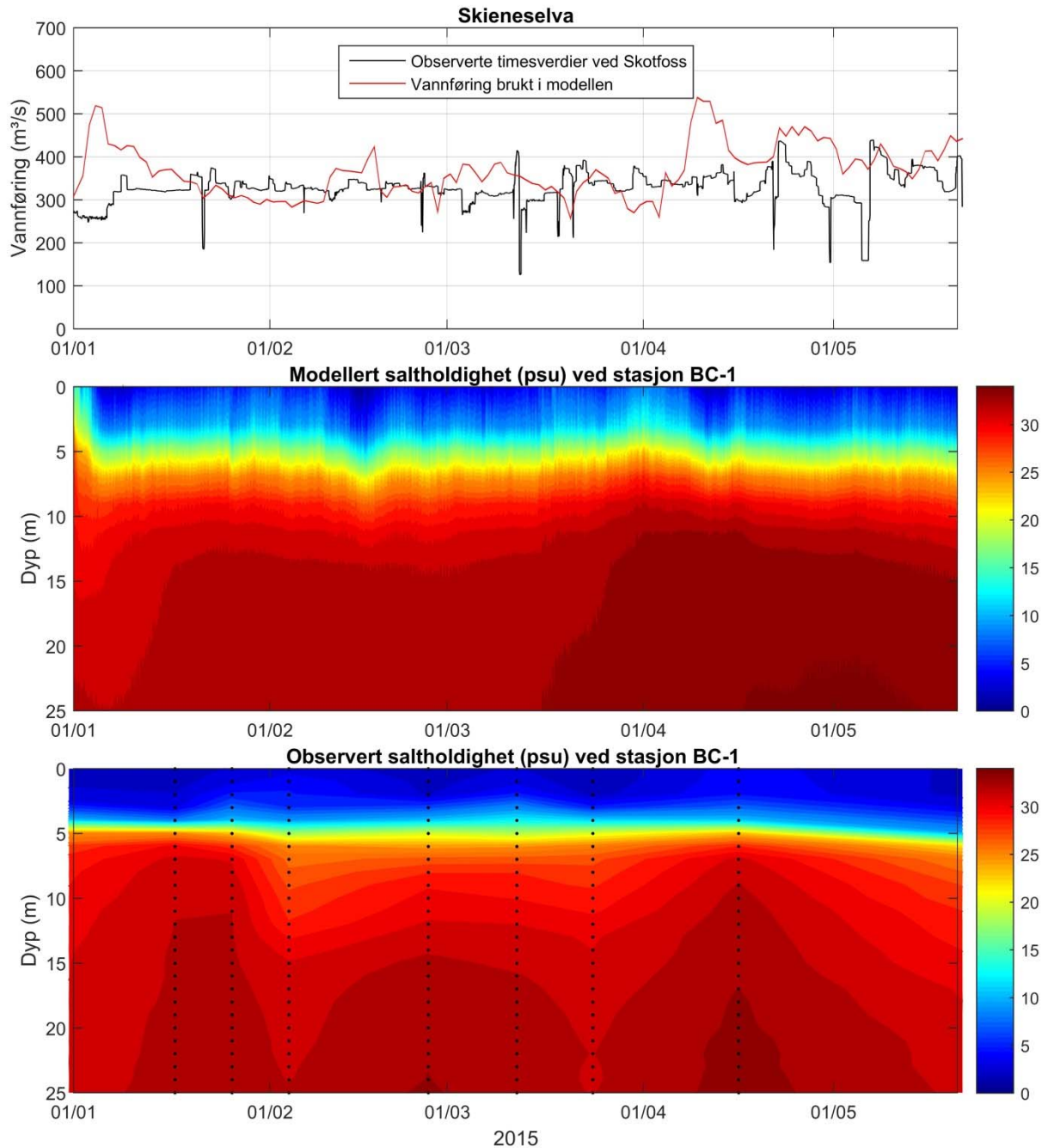
Figur 6. Vannføring i Skieneselva og saltholdighet i de øverste 25 meterne ved stasjon BC-1 midt i Friertfjorden. Øverst vises vannføring målt ved Skotfoss i Skieneselva og den vannføringen som er brukt i modellen. I midten vises modellert saltholdighet og nederst vises observert saltholdighet. De svarte prikkene i den nederste figuren viser hvor det er observasjoner.
