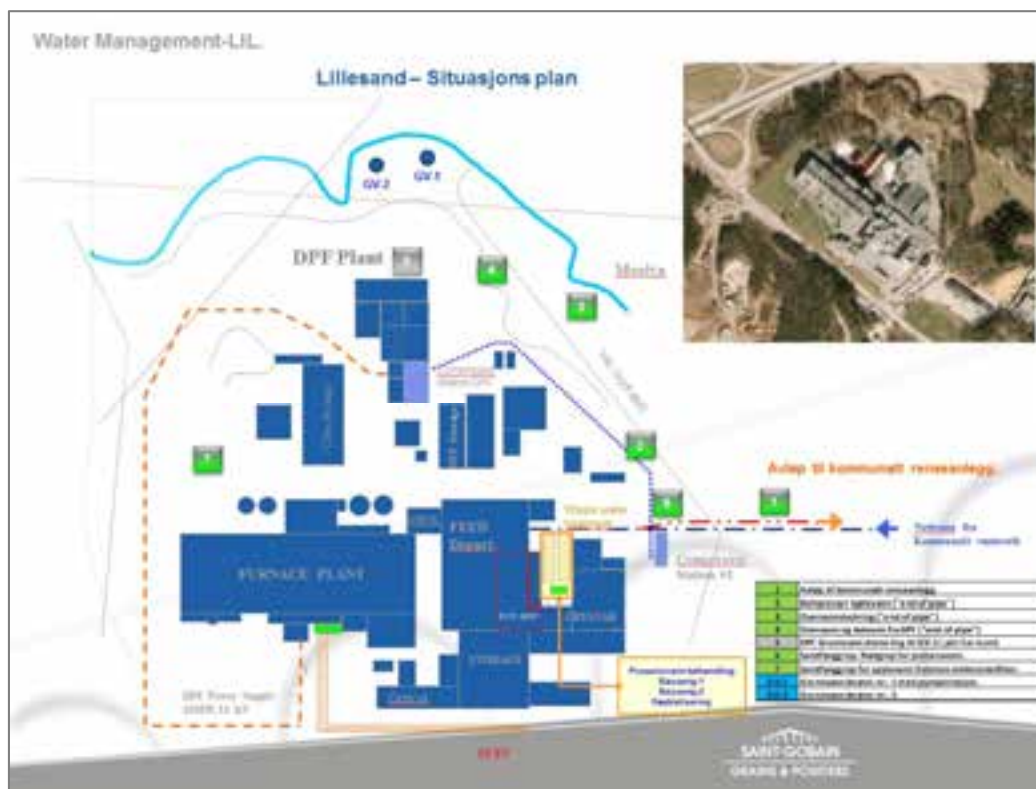
Figur 2. Oversikt over vannflyt i SG Lillesand. Punkt 1 viser avløp til kommunalt nett, via internt rensanlegg (basseng 1 og 2) og med nødgrøp (sandfang; pkt 6). GV-1 og GV-2 er grunnvannsbrønner, mens punkt 7 er den sandfanggroppa som inntil mai 2015 ble brukt for spylevann fra mange av ovnhuspipenes elektrostatfiltere. Pkt 3 er utslipp til Moelva og pkt 4 er utslipp til grunnen av oppsamlet overvann fra faste flater og takvann.
