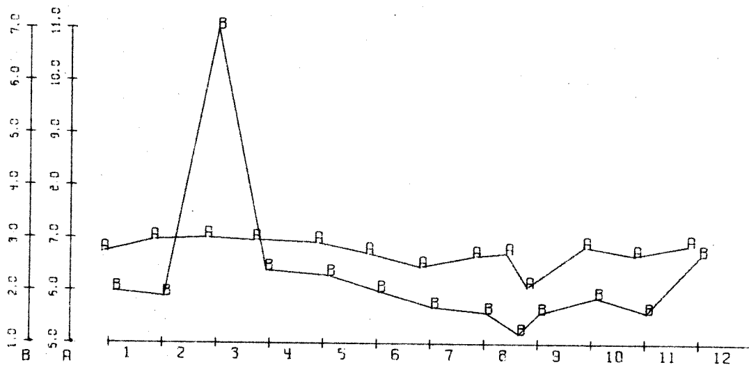
Fig. 28. Stasjon El. Grafisk fremstilling av analyseresultater 1977. pH og sulfat.
