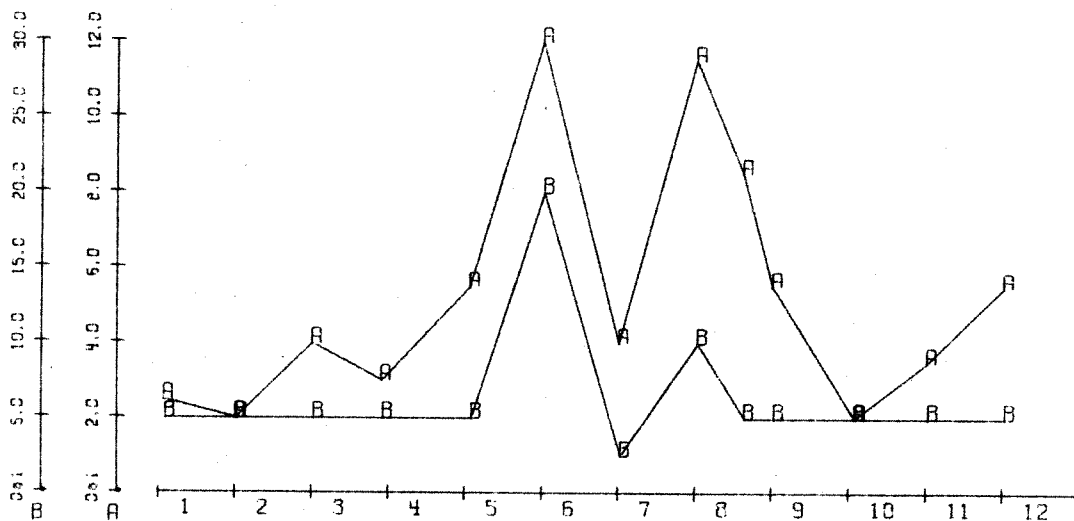
Fig. 29. Stasjon El. Grafisk fremstilling av analyseresultater 1977: Kobber og sink.
