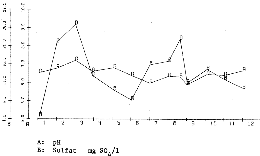
Fig. 25. Stasjon B10. Grafisk fremstilling av analyseresultater 1977: pH og sulfat.
