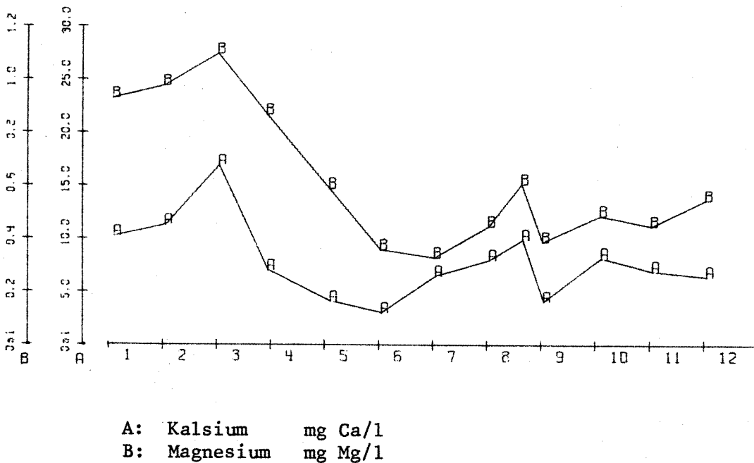
Fig. 26. Stasjon B10. Grafisk fremstilling av analyseresultater 1977: Kalsium og magnesium.
