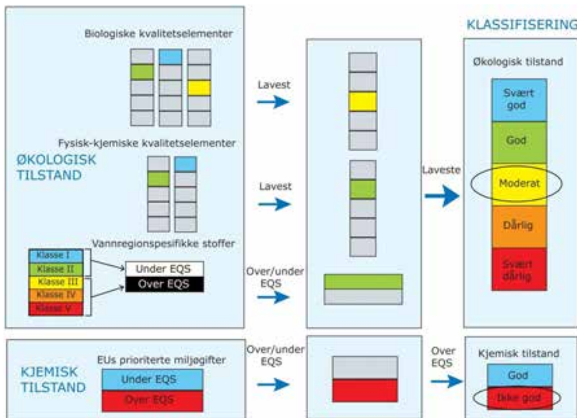
Figur 5. Prinsippskisse som viser klassifisering av miljøtilstand i en vannforekomst. De ulike kvalitetselementer som inngår i vurdering av økologisk og kjemisk tilstandsvurdering er vist. EQS-verdier (Environmental Quality Standards) angir miljøkvalitetsstandarder, også kalt grenseverdier. Piler påtegnet
