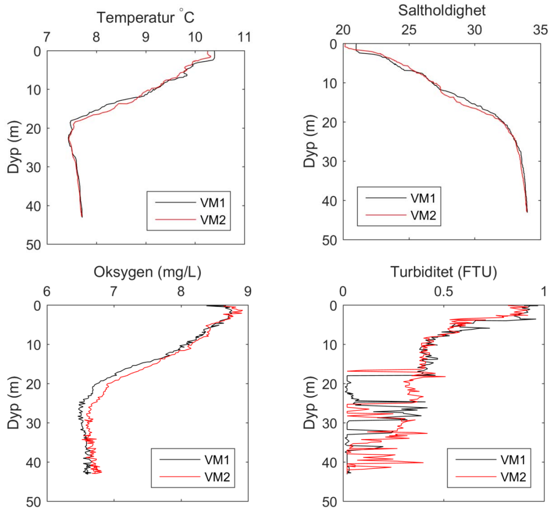
Figur 13. Temperatur saltholdighet, oksygen og turbiditet på stasjonene VM1 og VM2 i Beitstadfjorden. Målt med sonde ned til drøyt 40m dyp 15. juni 2015.
