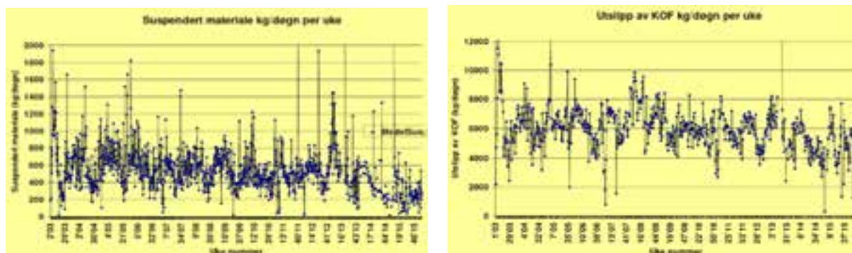
Figur 2. Utslippstall for perioden 2003 til og med 2015 gitt som kg/døgn per uke for STS og KOF M (Kilde Hellefoss Paper AS).
