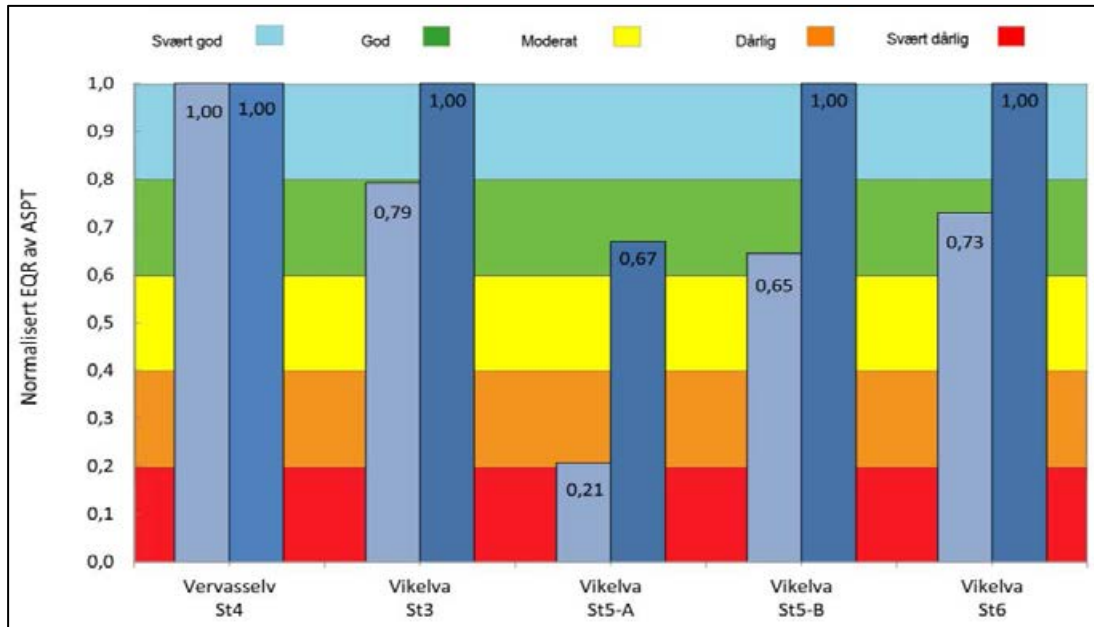
Figur 18. Miljøtilstand mht. organisk belastning og eutrofiering den 7. april og 28. august 2016 basert på bunndyrsmfunnets sammensetning og normaliserte indeksverdier for ASPT.
