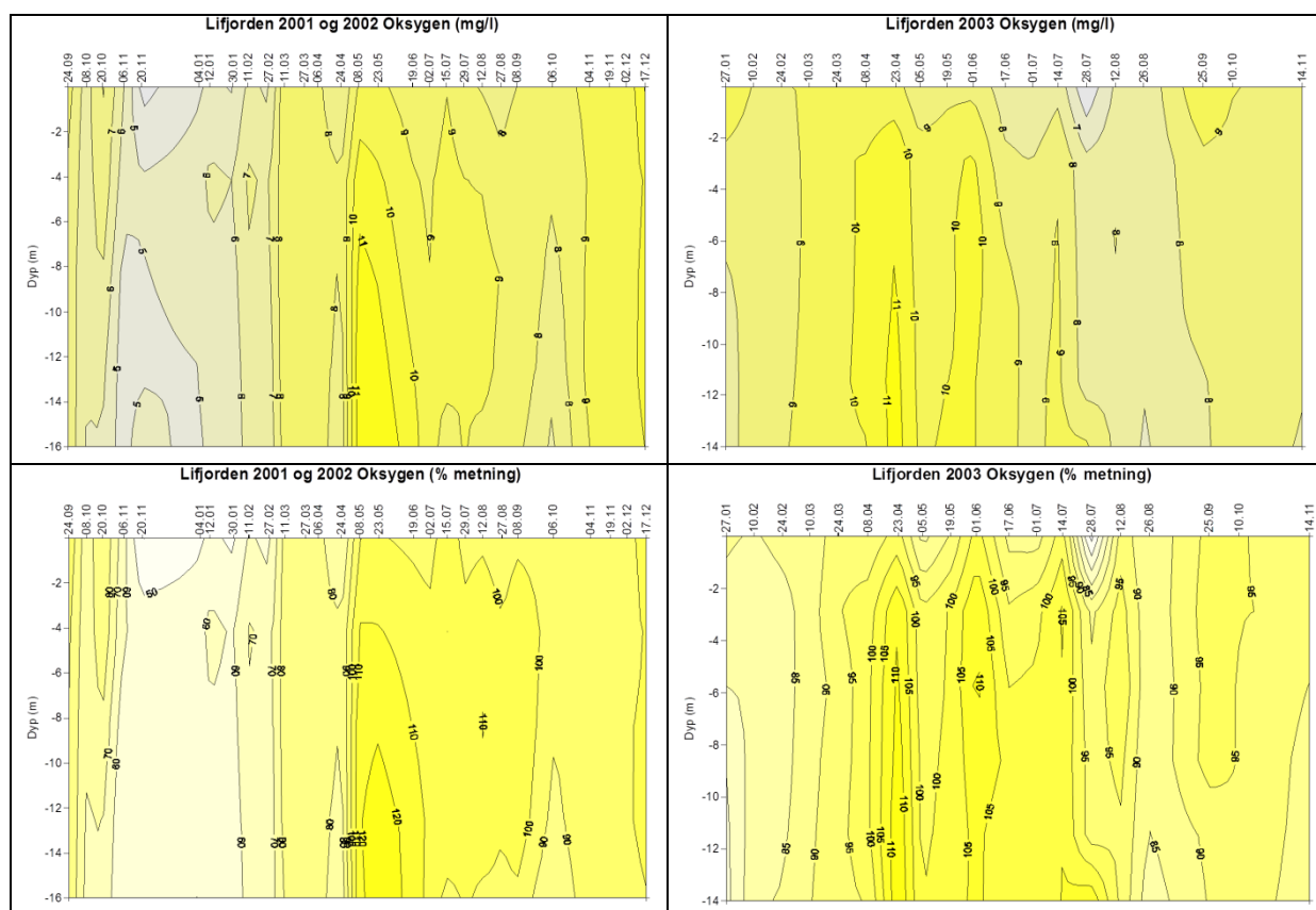
Figur 52. Oksygenkonsentrasjoner og oksygenmetning på lokaliteten Hyllestad i Liffjorden i perioden 2001-2003.
