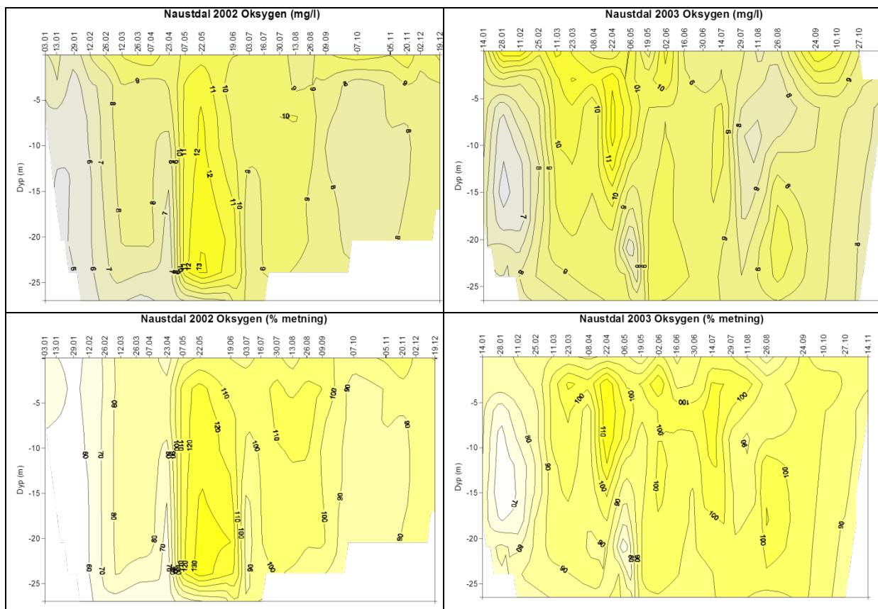
Figur 40. Oksygenkonsentrasjoner og oksygenmetning på lokaliteten Naustdal i Førdefjorden i perioden 2002-2003.
