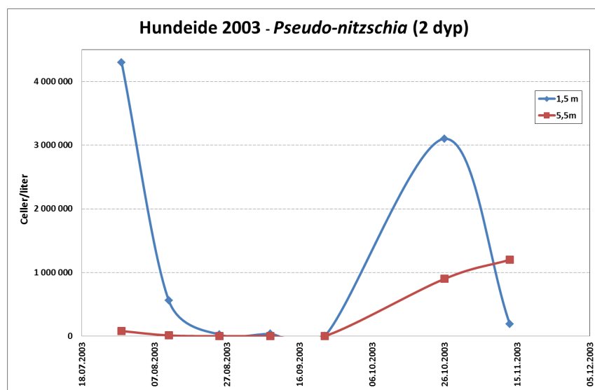
Figur 24. Utviklingen av Pseudo-nitzschia delicatissima -typen i perioden 29. juli-13. november 2003 på 1,5 og 5,5 m dyp på lokaliteten Hundeide i Eid.
