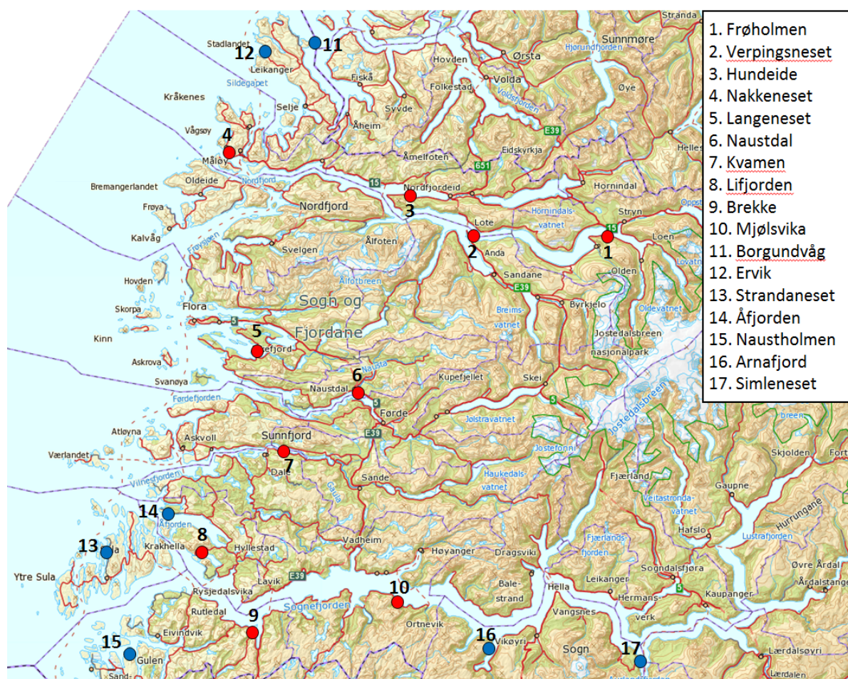
Figur 1. Kart med markering av testlokalitetene. De røde punktene angir lokalitetene som er omtalt i denne rapporten, mens de blå punktene angir lokaliteter hvor det ikke er gjennomført hydrografiske målinger og som ikke inngår i rapporten.
