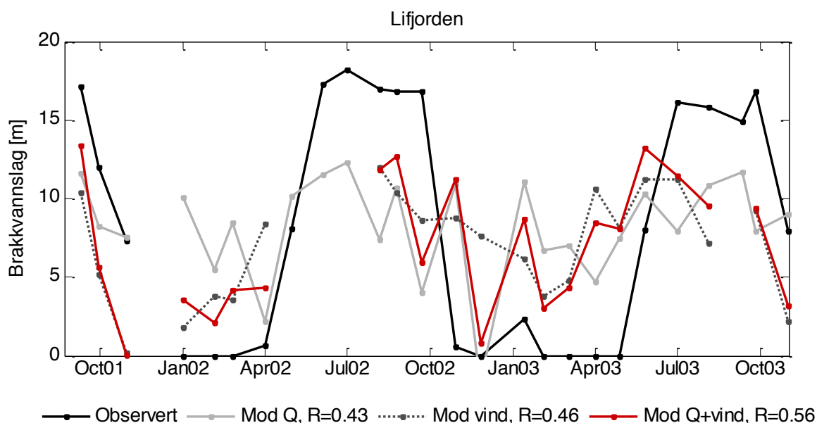
Figur 51. Observerte månedsmiddel av brakkvannslagets tykkelse (svart heltrukken linje) og resultat fra brakkvannsmoellene (lys grå = kun elv, grå stiplet = kun vind, rød = elv+vind).
