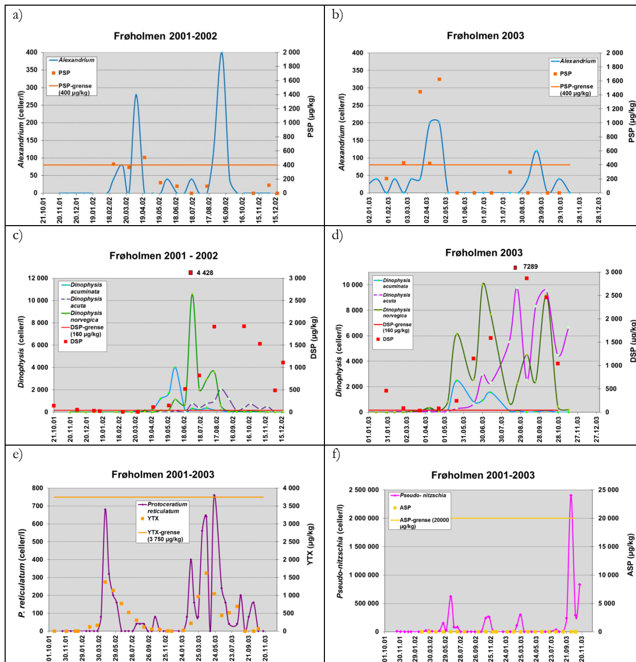
Figur 8. Forekomster av Alexandrium tamarense i a) 2001-2002 og b) 2003, Dinophysis i c) 2001-2002 og d) 2003, e) Protoceratium reticulatum i 2001-2003 og f) Pseudo-nitzschia i 2001-2003 på lokaliteten Frøholmen i Stryn.
