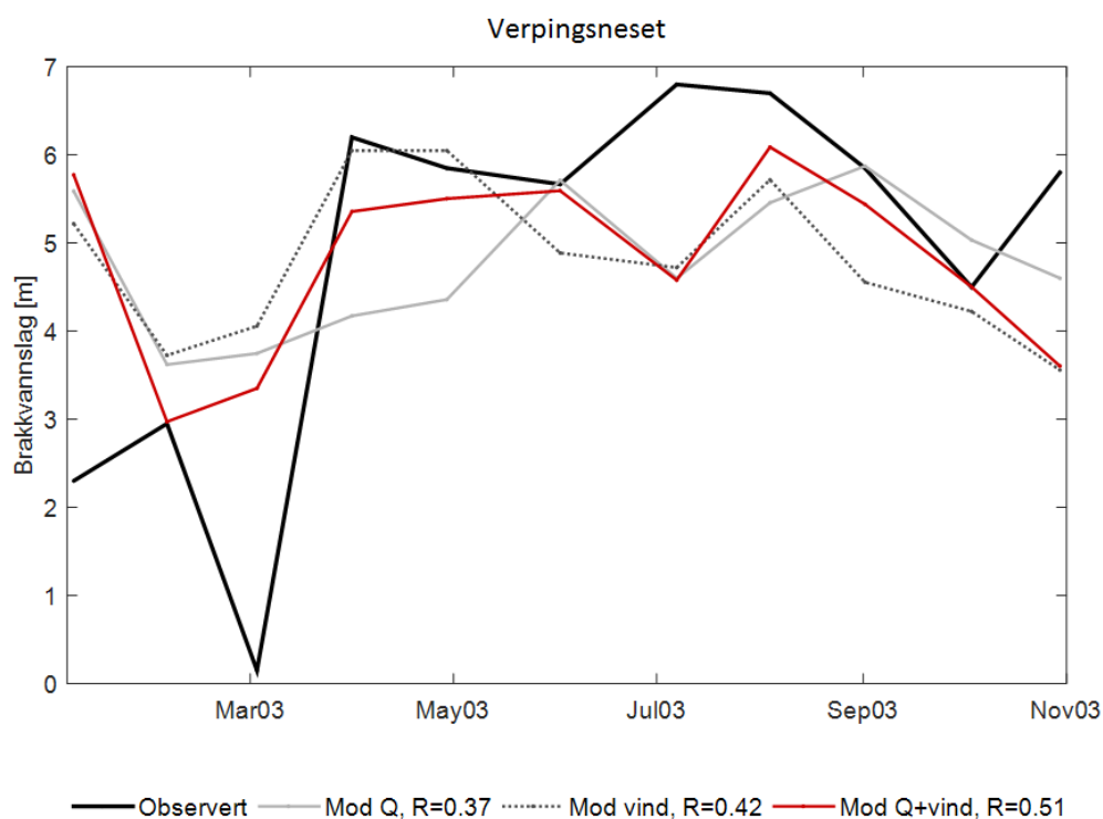
Figur 12. Observerte månedsmiddel av brakkvannslagets tykkelse (svart heltrukket linje) og resultat fra brakkvannsmoellene (lys grå = kun elv, grå stiplet = kun vind, rød = elv+vind).
