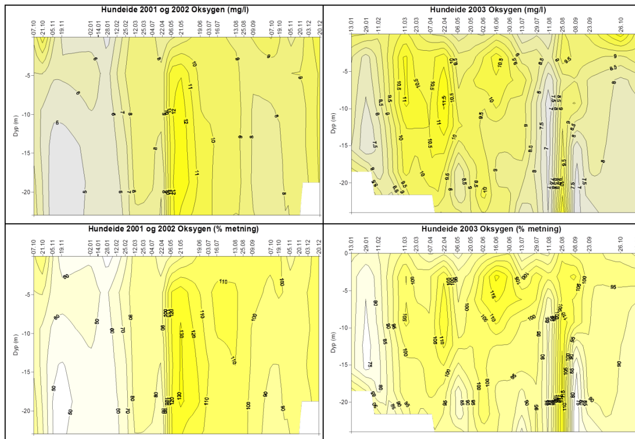
Figur 20. Oksygenkonsentrasjoner og oksygenmetning på lokaliteten Hundedeide i Eid i perioden 2001-2003.
