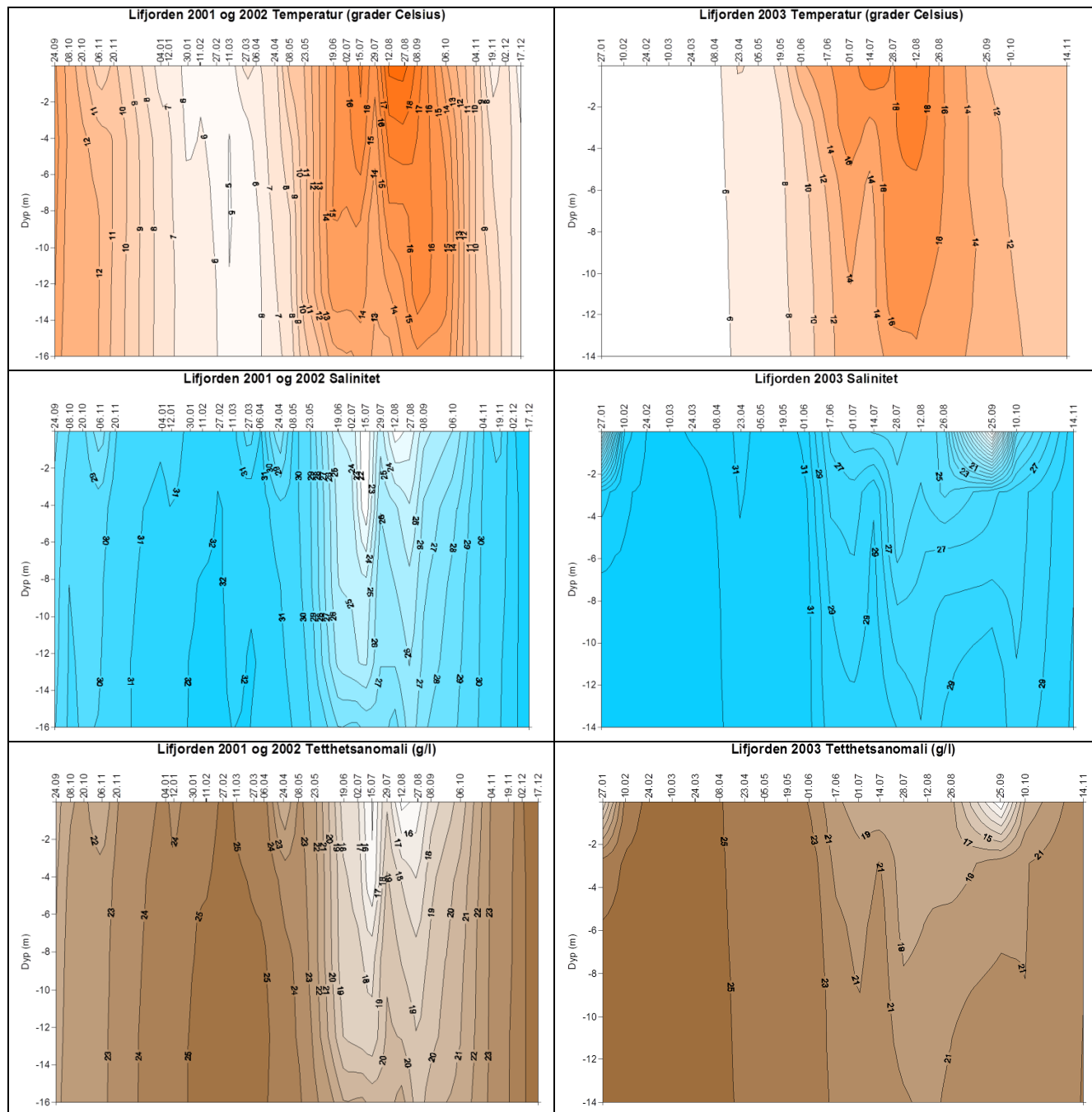
Figur 49. Temperatur, salinitet og tetthetsanomalier på lokaliteten Hyllestad i Lifjorden i perioden 2001-2003.
