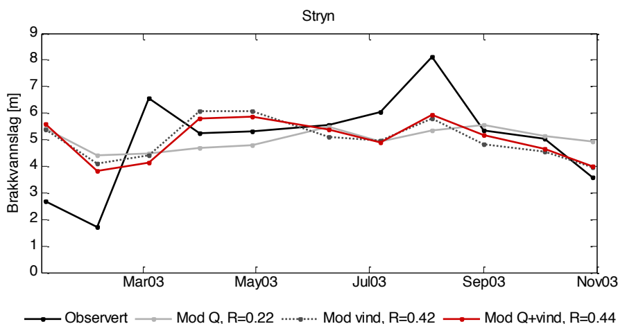
Figur 5. Observerte månedsmiddel av brakkvannslagets tykkelse (svart heltrukken linje) og resultat fra brakkvannsmodellene (lys grå = kun elv, grå stiplet = kun vind, rød = elv+vind).
