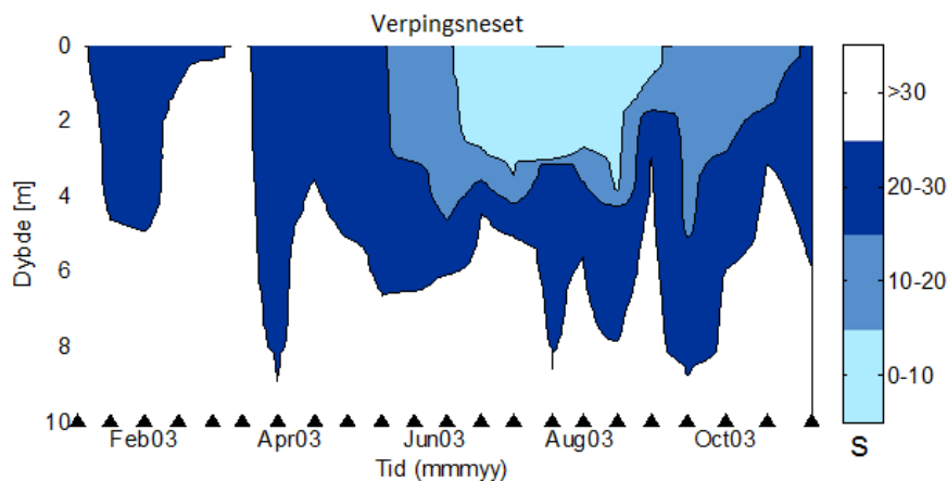
Figur 11. Utvikling av brakkvannslagets dybde ved Verpingsneset. De svarte trekantene angir måletidspunkt. Brakkvannet er farget blått med inndeling etter salinitet.
