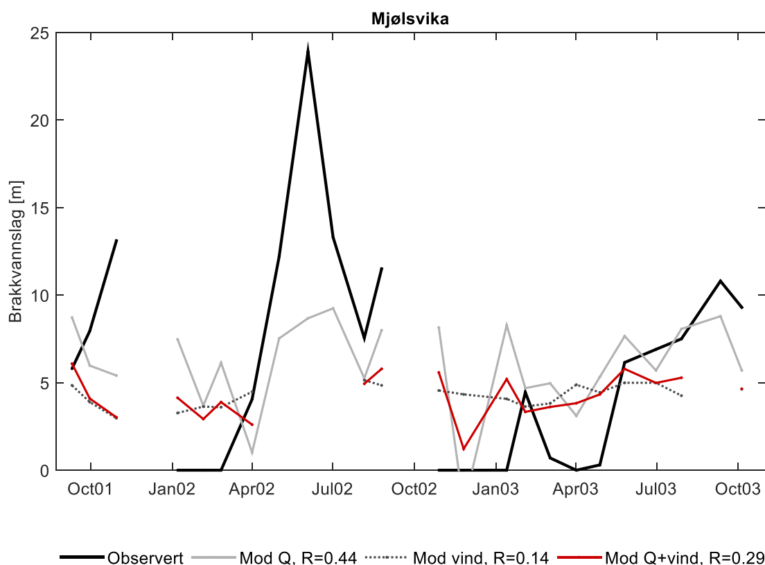
Figur 62. Observerte månedsmiddel av brakkvannslagets tykkelse (svart heltrukken linje) og resultat fra brakkvannmodellene (lys grå = kun elv, grå stiplet = kun vind, rød = elv+vind).
