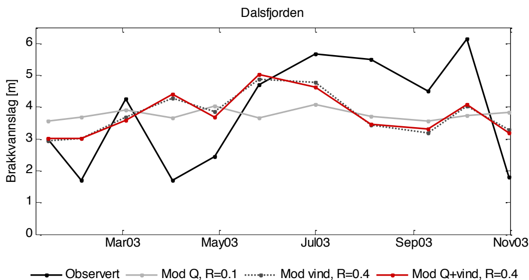
Figur 45. Observerte månedsmiddel av brakkvannslagets tykkelse (svart heltrukken linje) og resultat fra brakkvannsmoedellene (lys grå = kun elv, grå stiplet = kun vind, rød = elv+vind).
