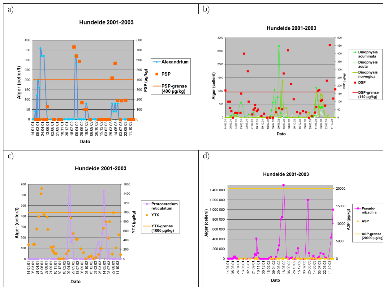
Figur 22. Forekomster i 2001-2003 av a) Alexandrium tamarense , b) Dinophysis , c) Protoceratium reticulatum og d) Pseudo-nitzschia på lokaliteten Hundefide i Eid.
