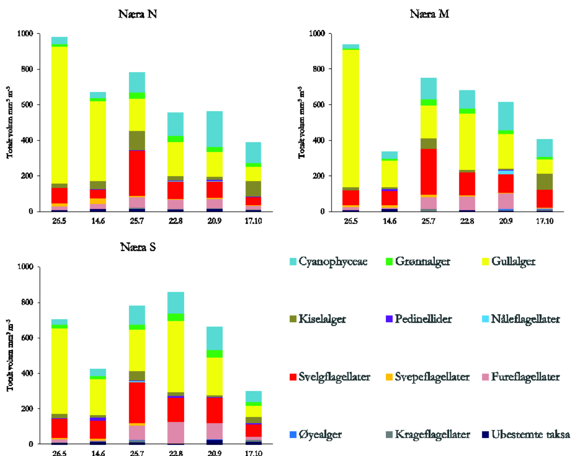
Figur 7. Totalmengde og sammensetting av planteplankton i Næra 2016.
