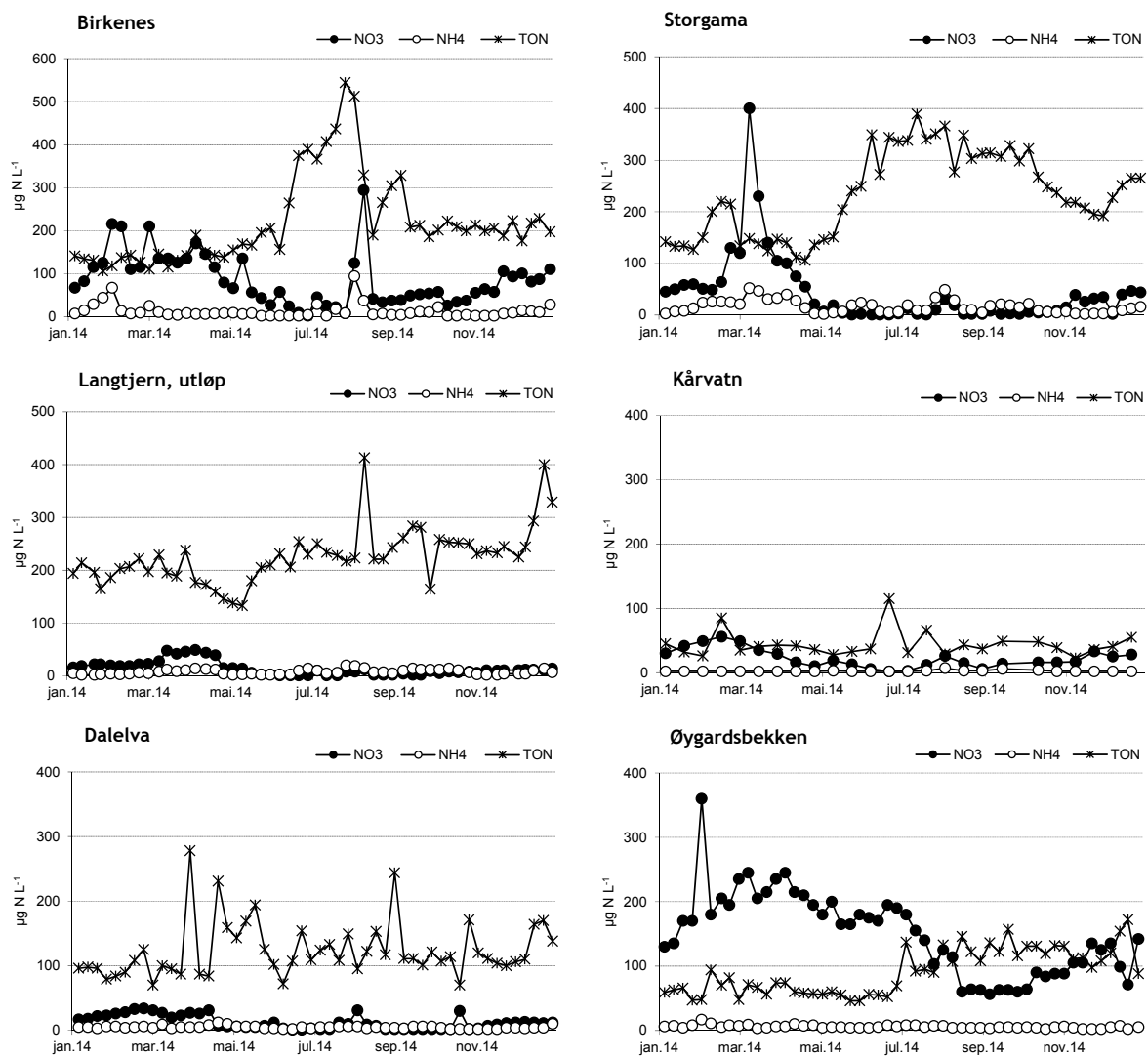
Figur 19. Sesongmessig fordeling av nitrat (NO 3 ), ammonium (NH 4 ) og totalt organisk nitrogen (TON) på feltforskningsstasjonene i 2014. TON = total nitrogen - NO 3 - NH 4 . NB! Uluk skala på y-aksene. Enhet: µg N L -1 .
