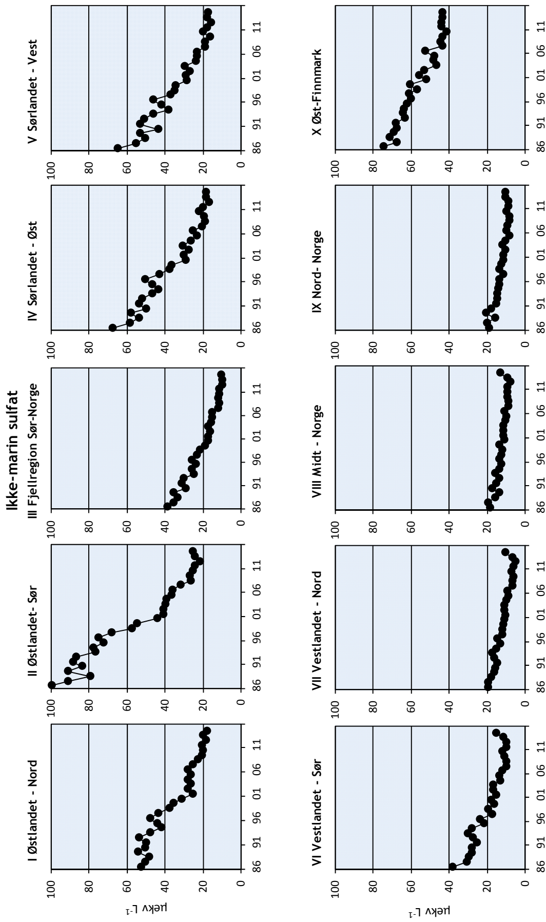
Figur 4. Trender for ikke-marin sulfat ( SO_4^{2-} ) for innsjøer i de 10 regionene for perioden 1986-2014.
