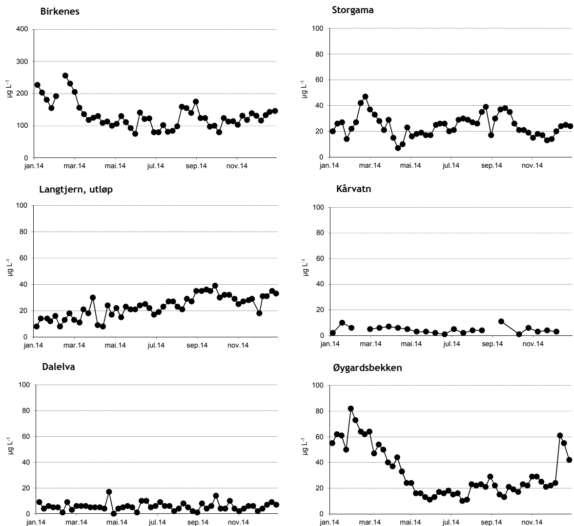
Figur 15. Sesongmessig fordeling av labilt uorganisk (bundet) aluminium (LAI) på feltforskningsstasjonene i 2014. NB! Ulitk skala på y-aksene. Enhet: \mu\text{g L}^{-1} .
