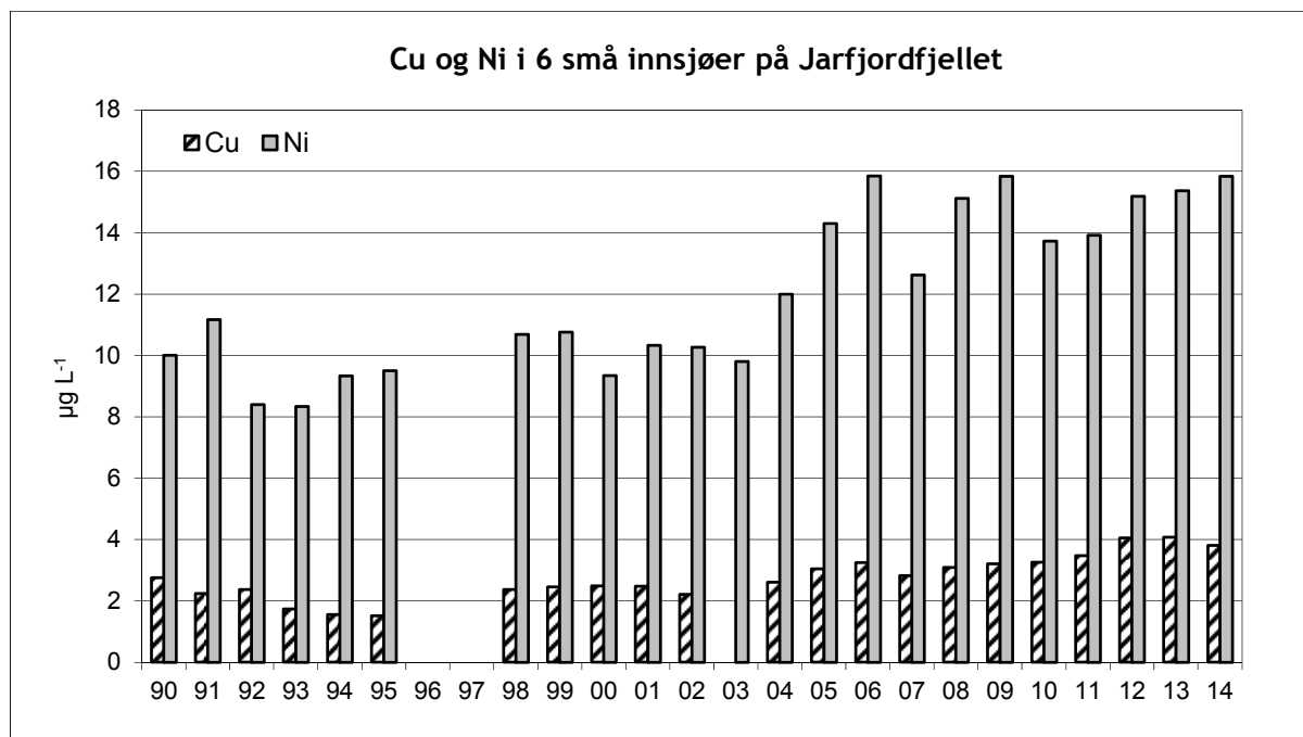
Figur 12. Årlige middelverdier for kobber og nikkel i seks små innsjøer på Jarfjordfjellet for perioden 1990-2014.
