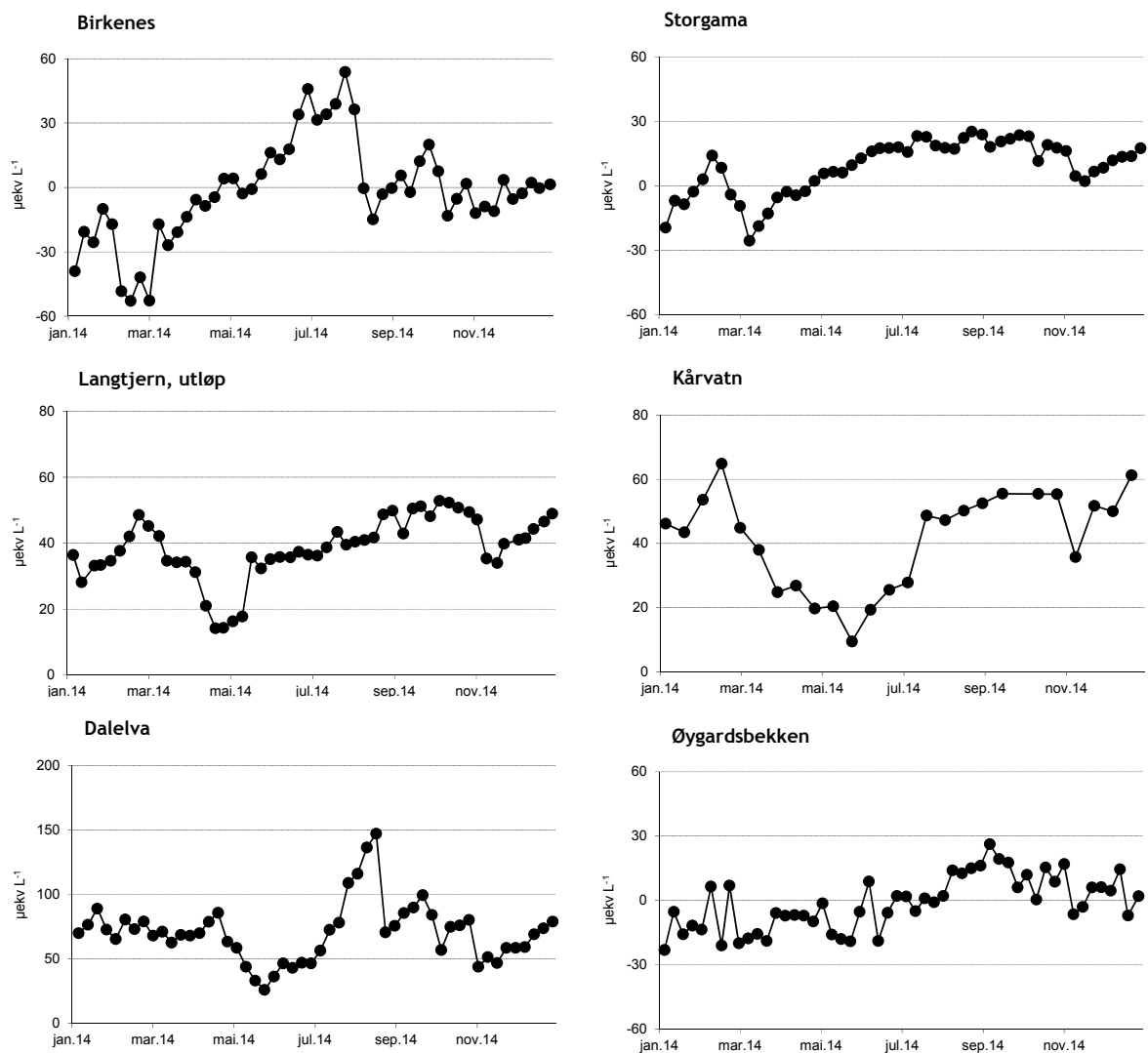
Figur 17. Sesongmessig fordeling av syrenøytraliserende kapasitet (ANC) på feltforskningsstasjonene i 2014. NB! Ulik skala på y-aksene. Enhhet: \mu\text{ekv L}^{-1} .
