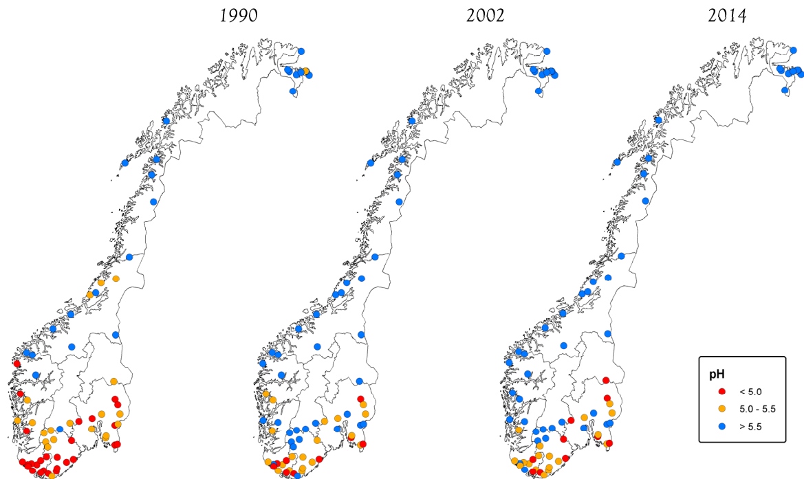
Figur 2. pH i overvåkingsinnsjøene i 1990, 2002 og 2014. Figuren illustrerer tydelig forbedringen i forurensingssituasjonen, ved at sjøene blir mindre sure (får høyere pH). Enkelte sjøer på Østlandet er fortsatt røde, og dette er forårsaket av høyt humusinnhold som gir naturlig lav pH.
