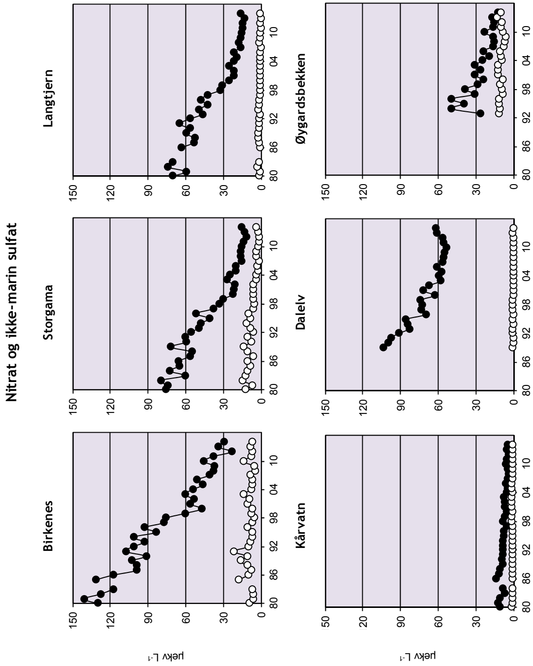
Figur 20. Trender for volumveid konsentrasjon av nitrat og ikke-marin sulfat for feltforskningsstasjonene for perioden 1980-2014. Ikke-marin sulfat ● og nitrat ○. Enhet: µekv L -1 .
