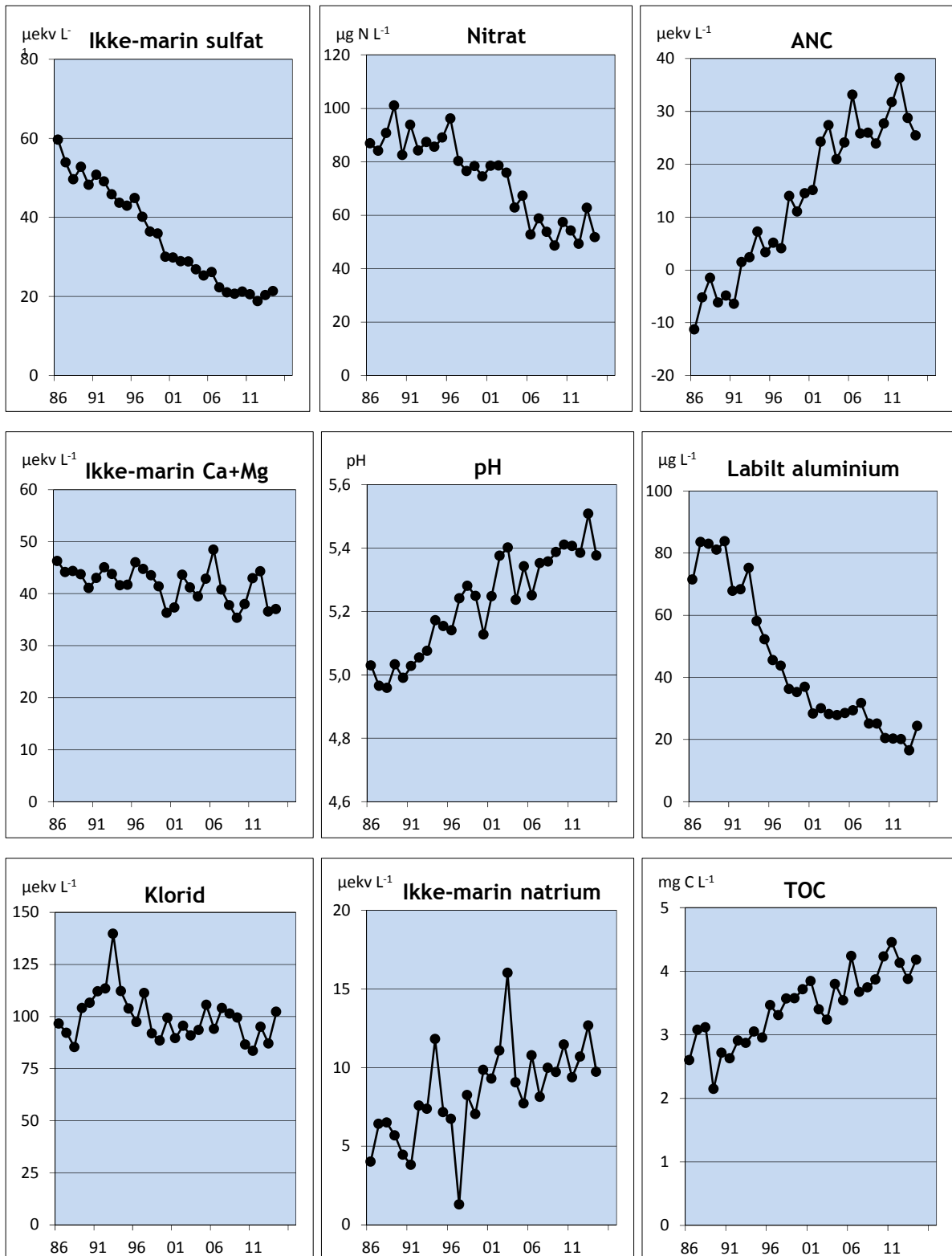
Figur 3. Endring i gjennomsnittlige konsentrasjoner for et utvalg av komponenter i 78 innsjøer fordelt over hele landet, for perioden 1986-2014.
