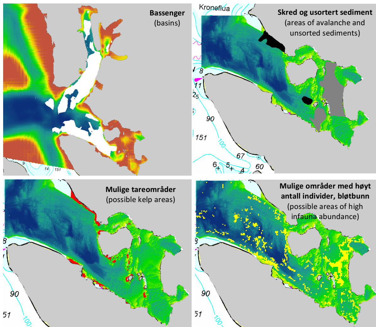
Figur 6. Fjordbassenger (hvite områder) modellert av NIVA basert på Havforskningsinstituttets dybdemodell med 160 m romlig oppløsning for Kongsfjorden, Krossfjord-, Møllerfjord, Lilliehøekfjord-systemet og området utenfor. Figuren viser også Kartverkets skredområder (svart) og områder med usorterte bunnsedimenter (grå), NIVAs modellerte mulige områder for tare (rødt) og mulige områder med over gjennomsnittlig høyt antall sedimentlevende dyr (infauna, gult).
