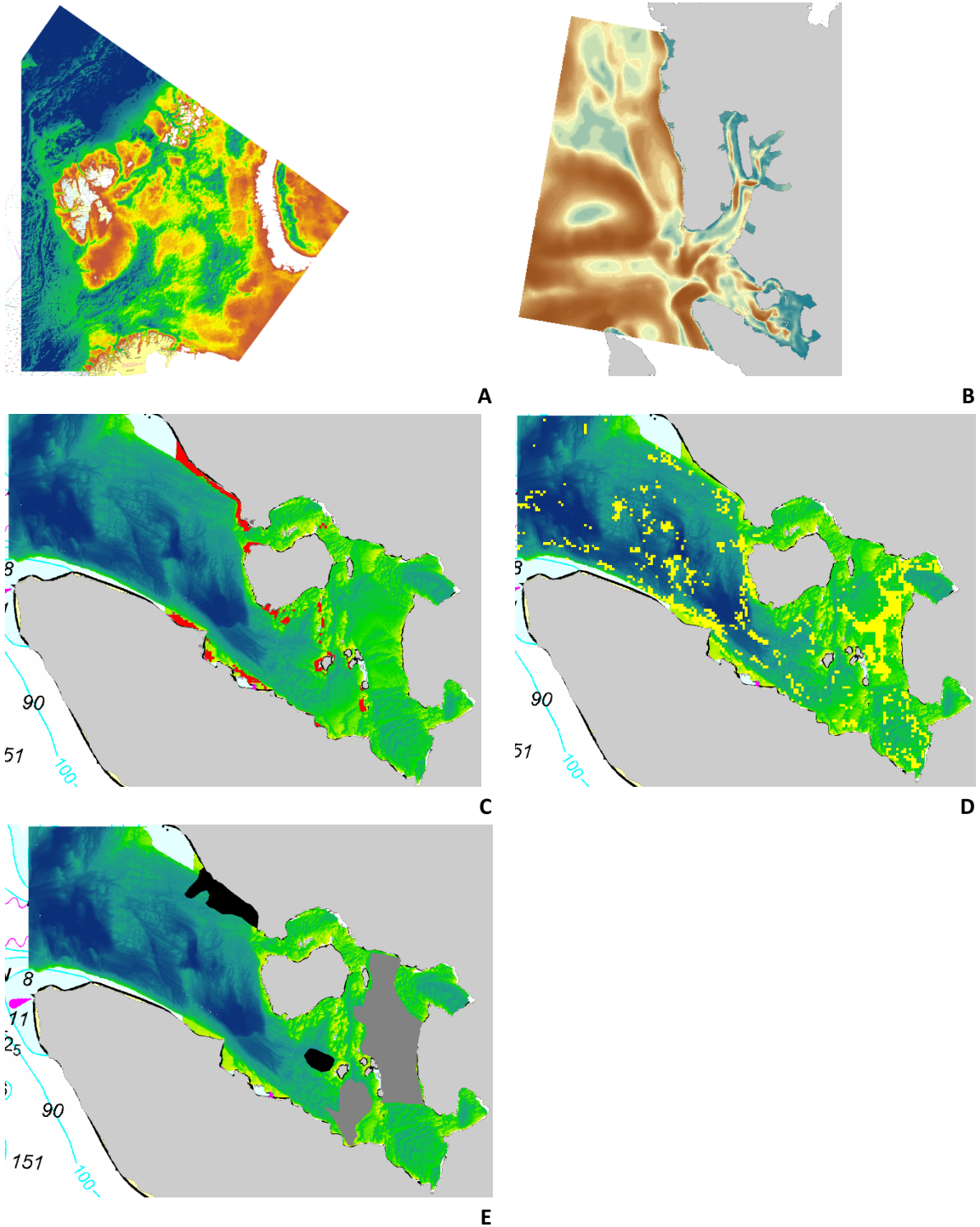
Figurene viser et utvalg av de modellene gjort tilgjengelig fra dette prosjektet. A: Dyp, modellert med 500 m romlig oppløsning, for hele Svalbard; B: Strømstyrke, modellert med 160 m oppløsning for Kongsfjorden, Krossfjord-, Møllerfjord og Lilliehöökfjordsystemet og området utenfor; C: Mulige tareområder (rødt), modellert for Kongsfjorden ved bruk av marine grunnkart med 5 m og 160 m oppløsning; D: Mulige bløtbunnsområder med høyt antall dyr (infauna, gult), modellert for Kongsfjorden ved bruk av marine grunnkart med 5 m og 160 m oppløsning; E: Områder med skred (sort) og usorterte sedimenter (grå) avgrenset for Kongsfjorden fra modell med 5 m romlig oppløsning.
