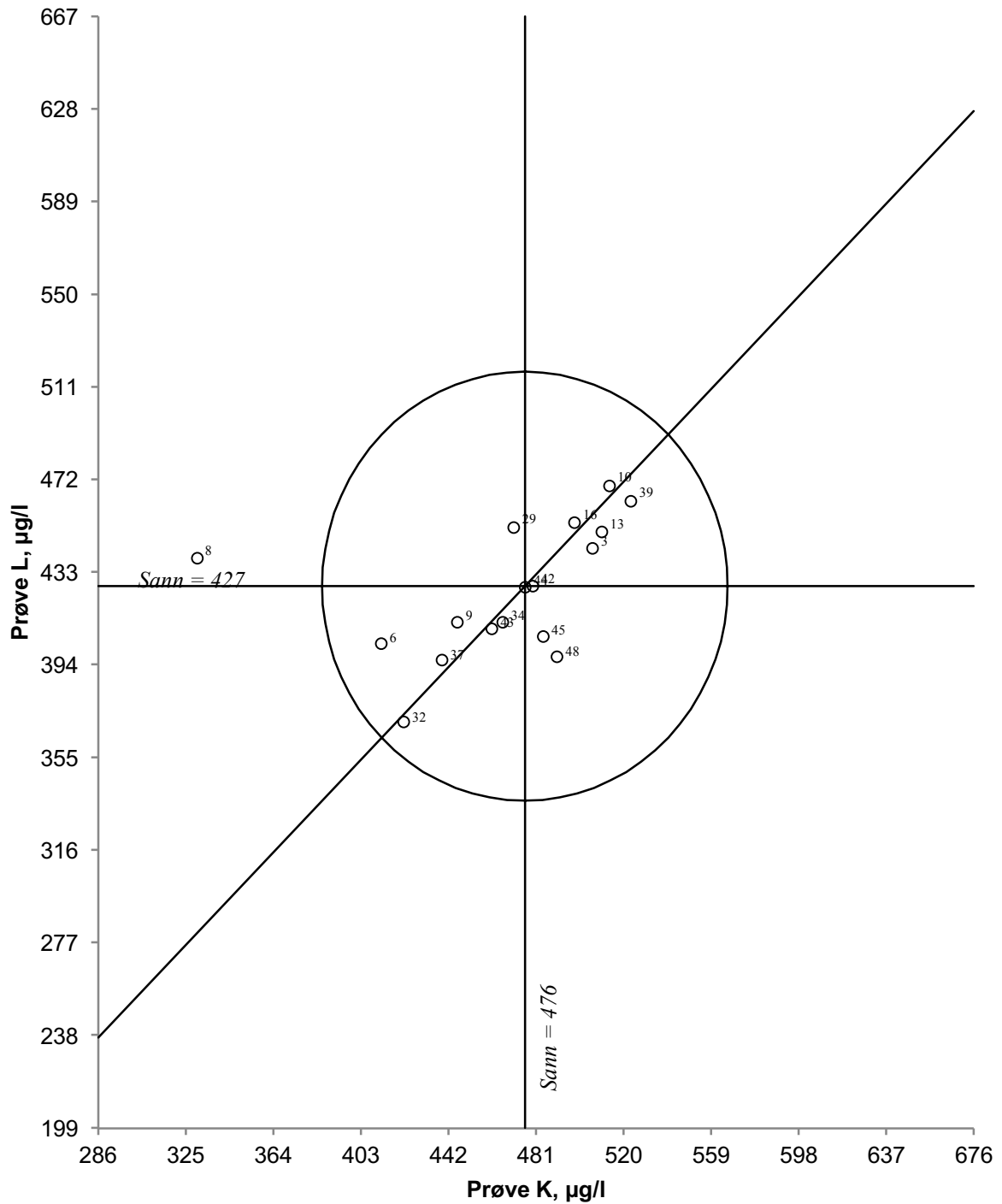
Figur 43. Youndendiagram for aluminium, prøvepar KL Akseptansegrensen, angitt med en sirkel, er 20 %
