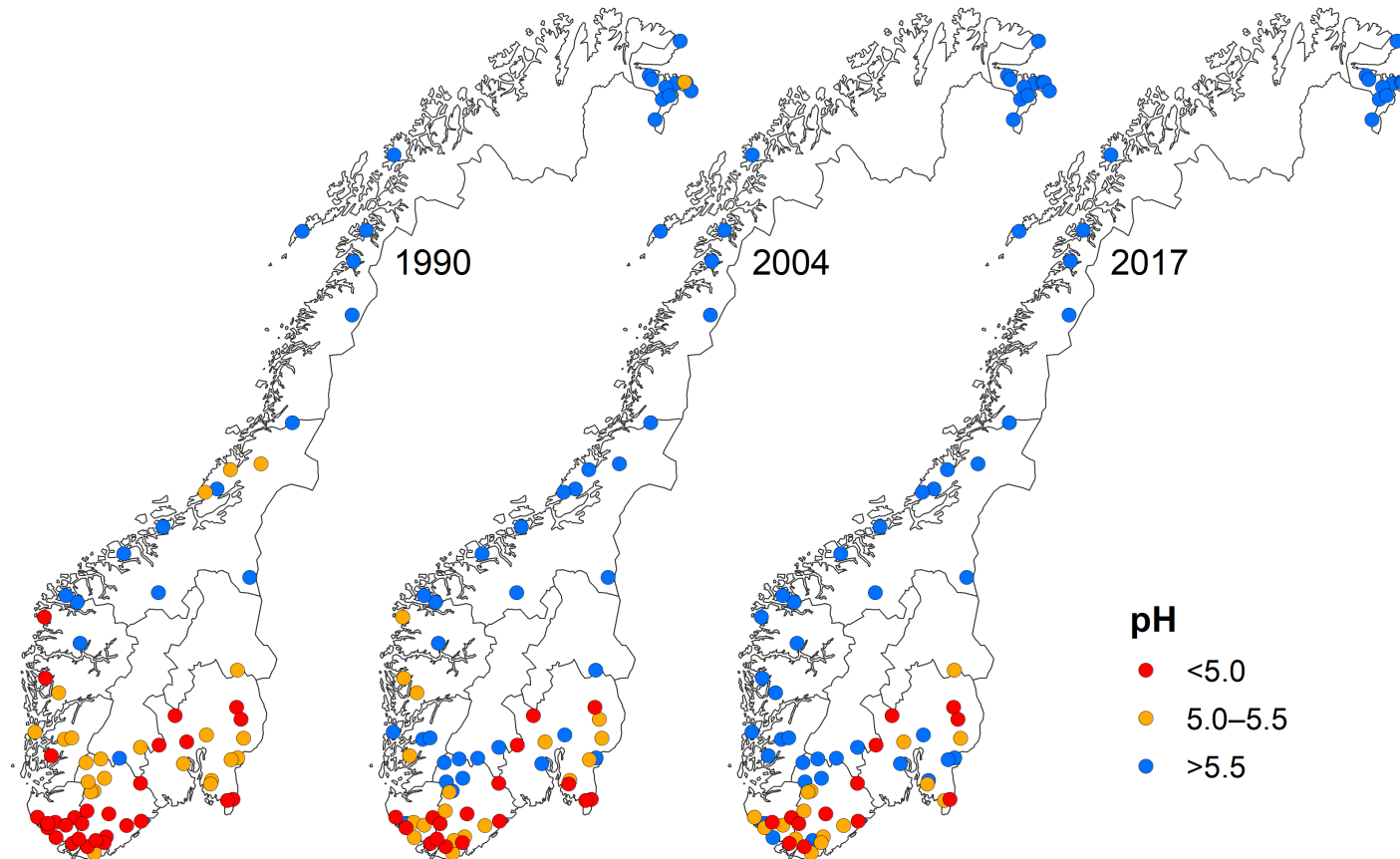
Figur 2. pH i overvåkingsinnsjøene i 1990, 2004 og 2017. Figuren illustrerer tydelig forbedringen i forsuringssituasjonen, ved at sjøene blir mindre sure (får høyere pH). Enkelte sjøer på Østlandet er fortsatt røde, og dette er forårsaket av høyt humusinnhold som gir naturlig lav pH.
