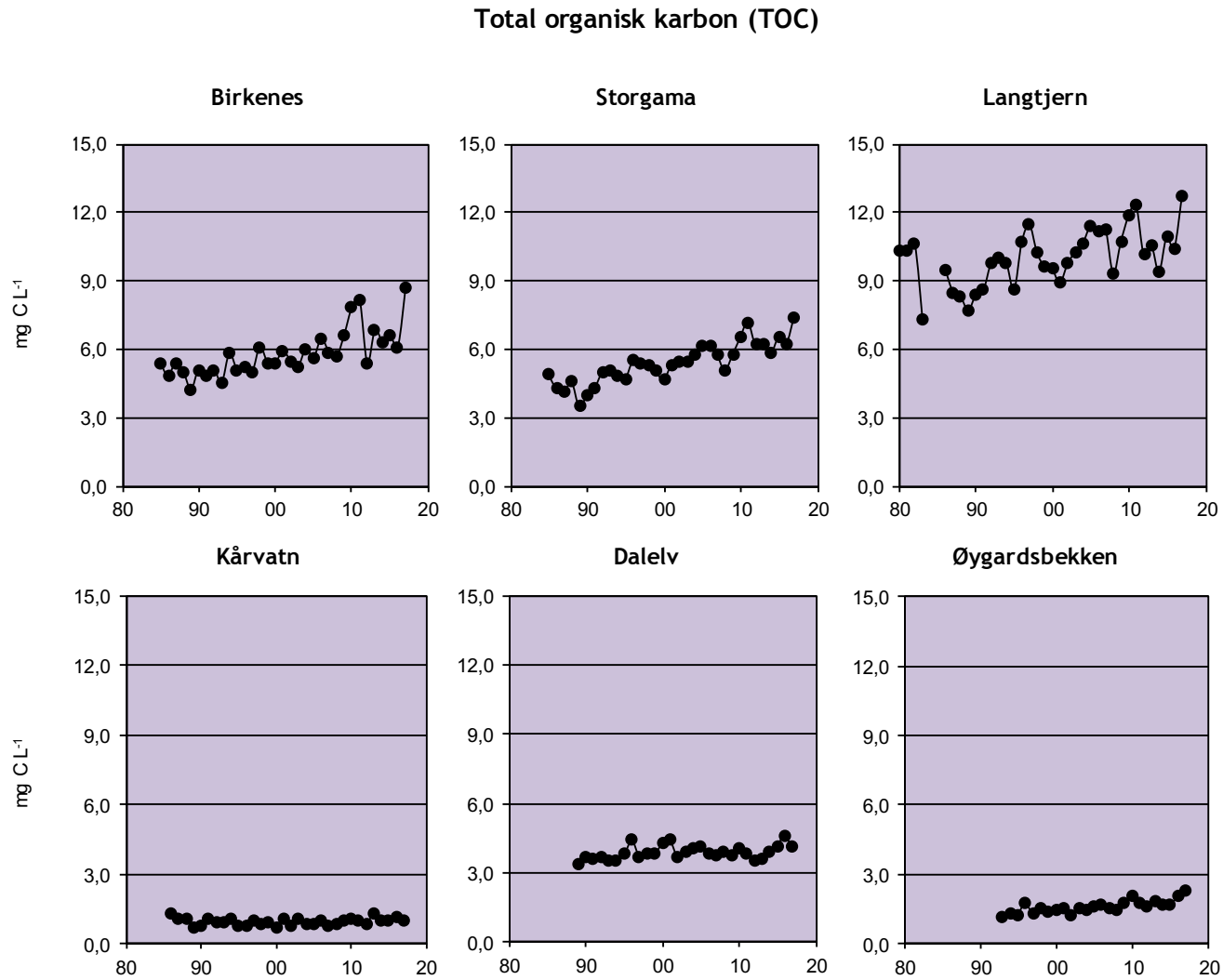
Figur 24. Trender for volumveid konsentrasjon TOC (totalt organisk karbon) for feltforskningsstasjonene for perioden 1980-2017. Enhet: mg C L -1 .
