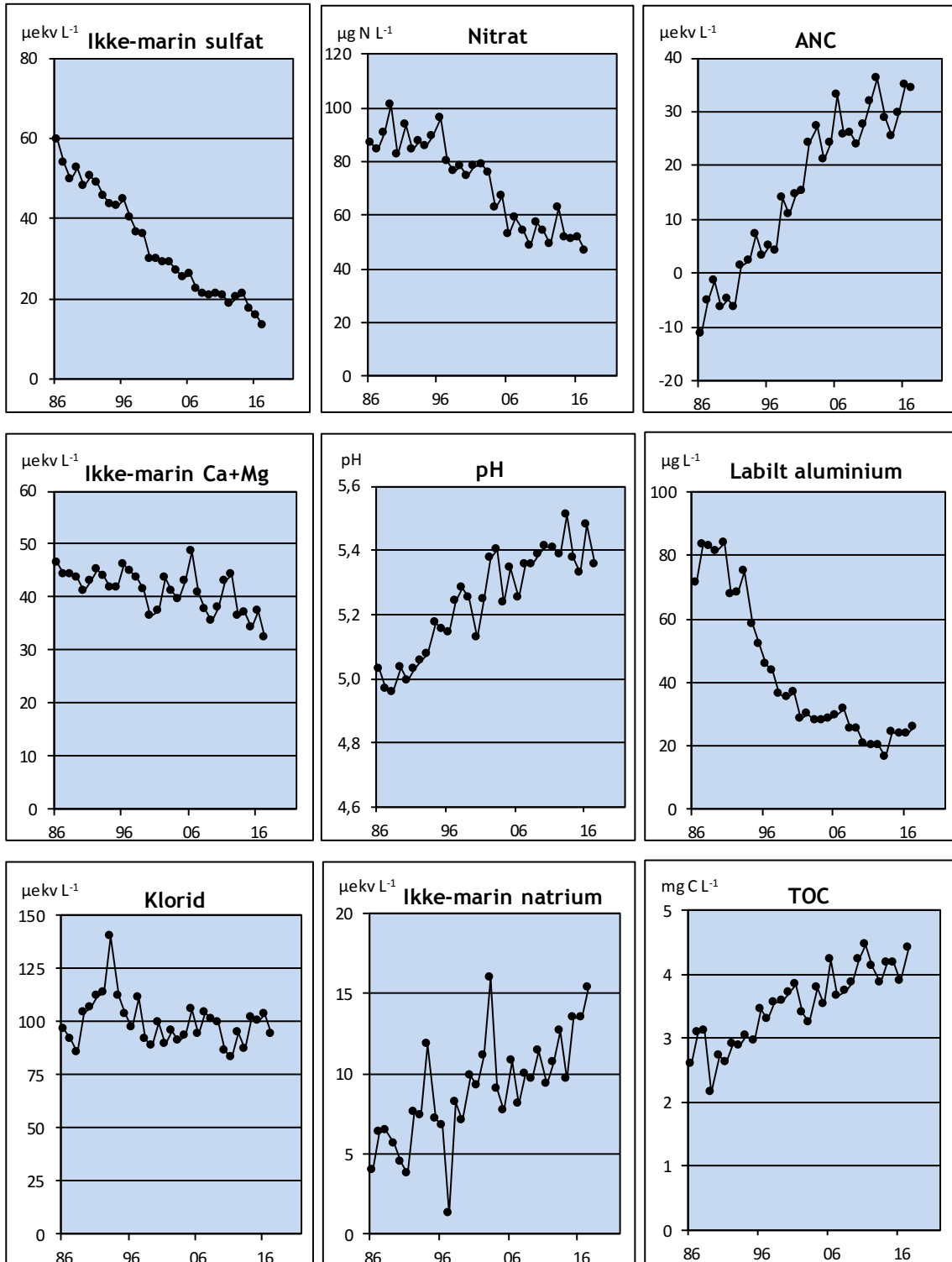
Figur 3. Endring i gjennomsnittlige konsentrasjoner for et utvalg av komponenter i 78 innsjøer fordelt over hele landet, for perioden 1986-2017.
