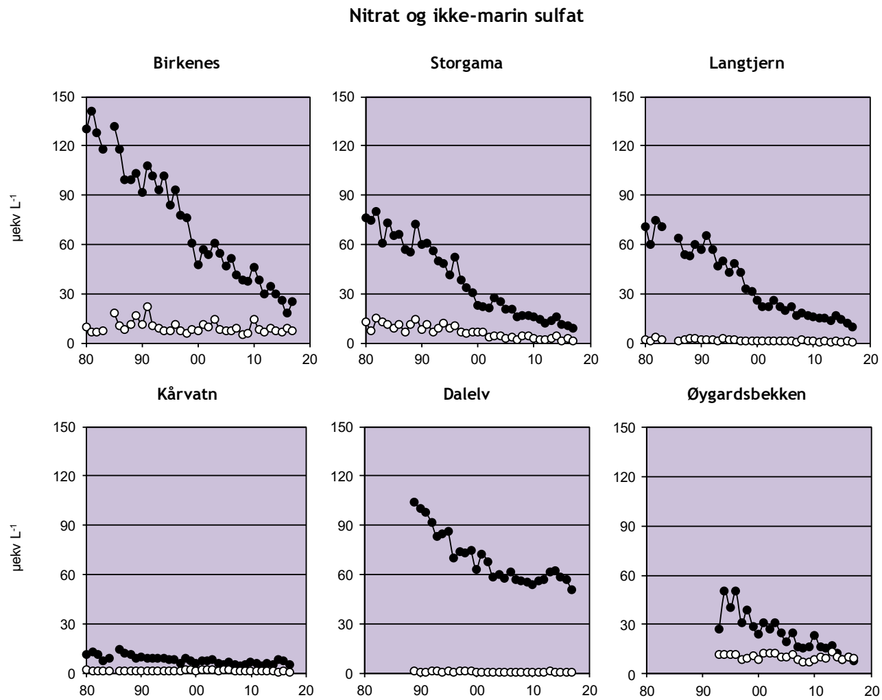
Figur 20. Trender for volumveid konsentrasjon av nitrat og ikke-marin sulfat for feltforskningsstasjonene for perioden 1980-2017. Ikke-marin sulfat ● og nitrat ○. Enhet: \mu\text{ekv L}^{-1} .
