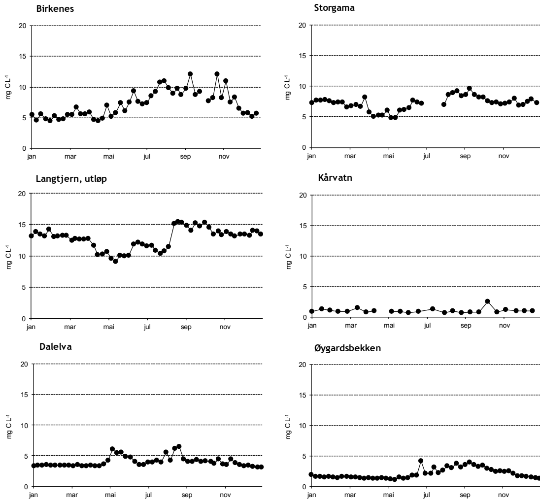
Figur 18. Sesongmessig fordeling av total organisk karbon (TOC) på feltforskningsstasjonene i 2017. Enhet: \text{mg C L}^{-1}
