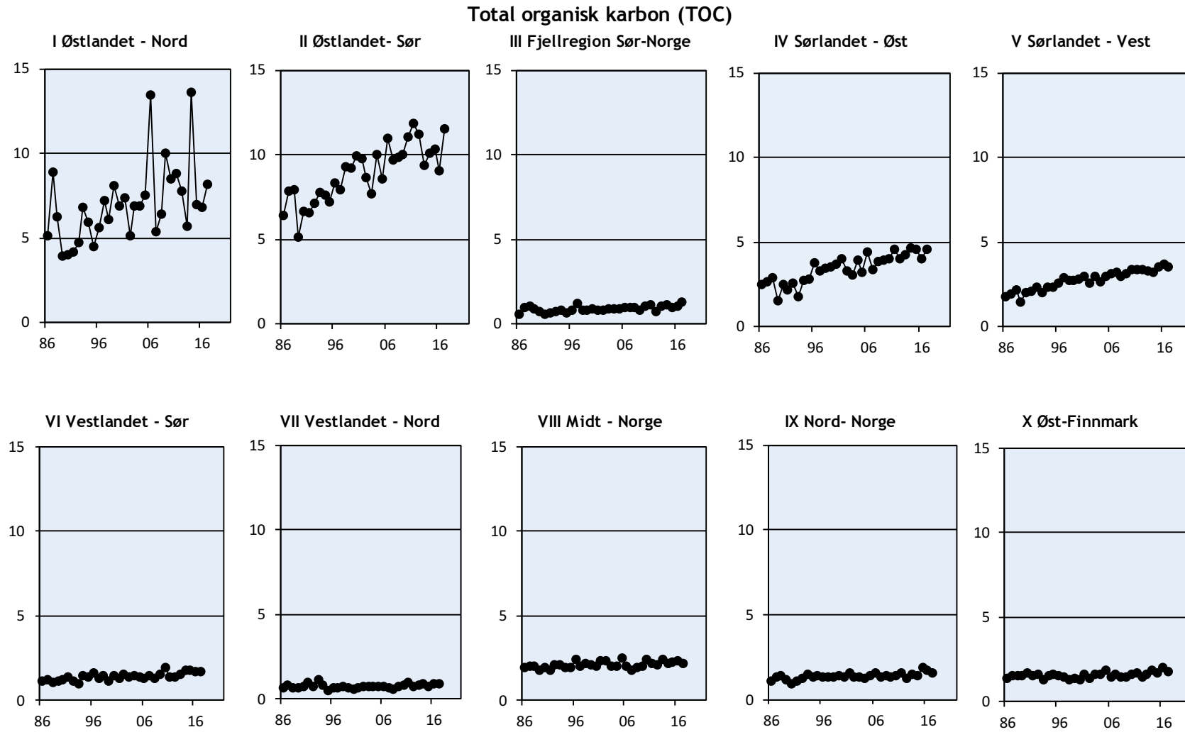
Figur 10. Trender for total organisk karbon (TOC) for innsjøer i de 10 regionene for perioden 1986-2017. Enhet: \text{mg C L}^{-1} .
