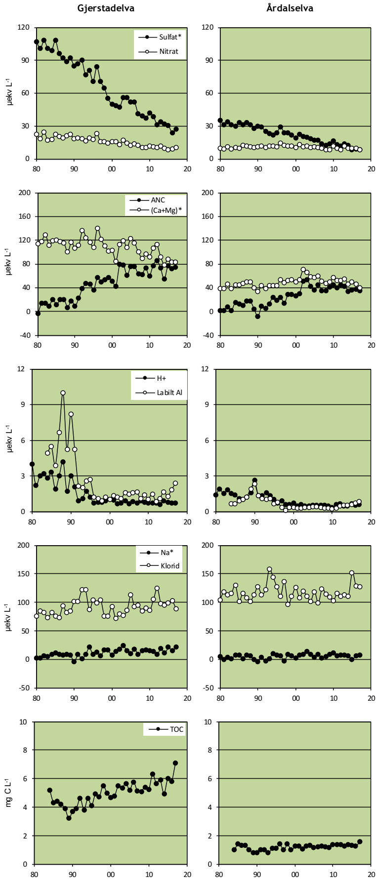
Figur 25. Årsmiddelverdier av utvalgte parametere for Gjerstadelva og Årdalselva for perioden 1980-2017.
