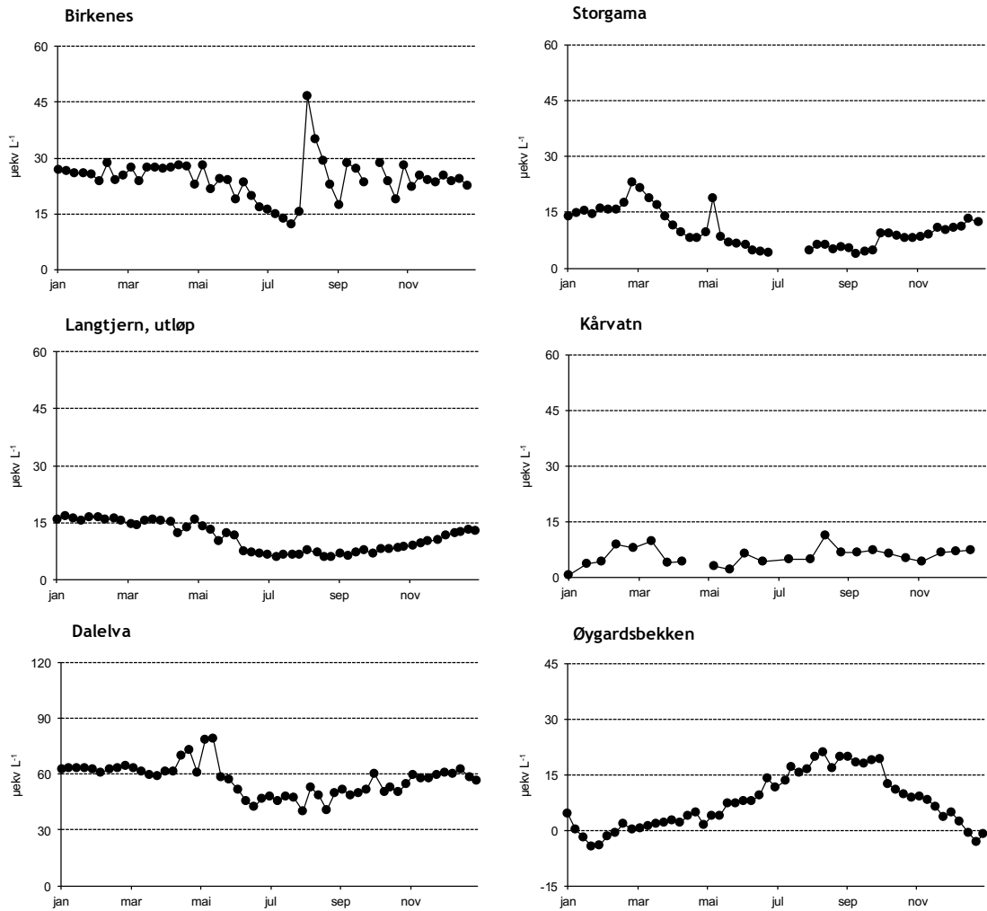
Figur 13. Sesongmessig fordeling av ikke-marin sulfat på feltforskningsstasjonene i 2017. NB! Ulik skala på y-aksene. Enhet: µekv L -1 .
