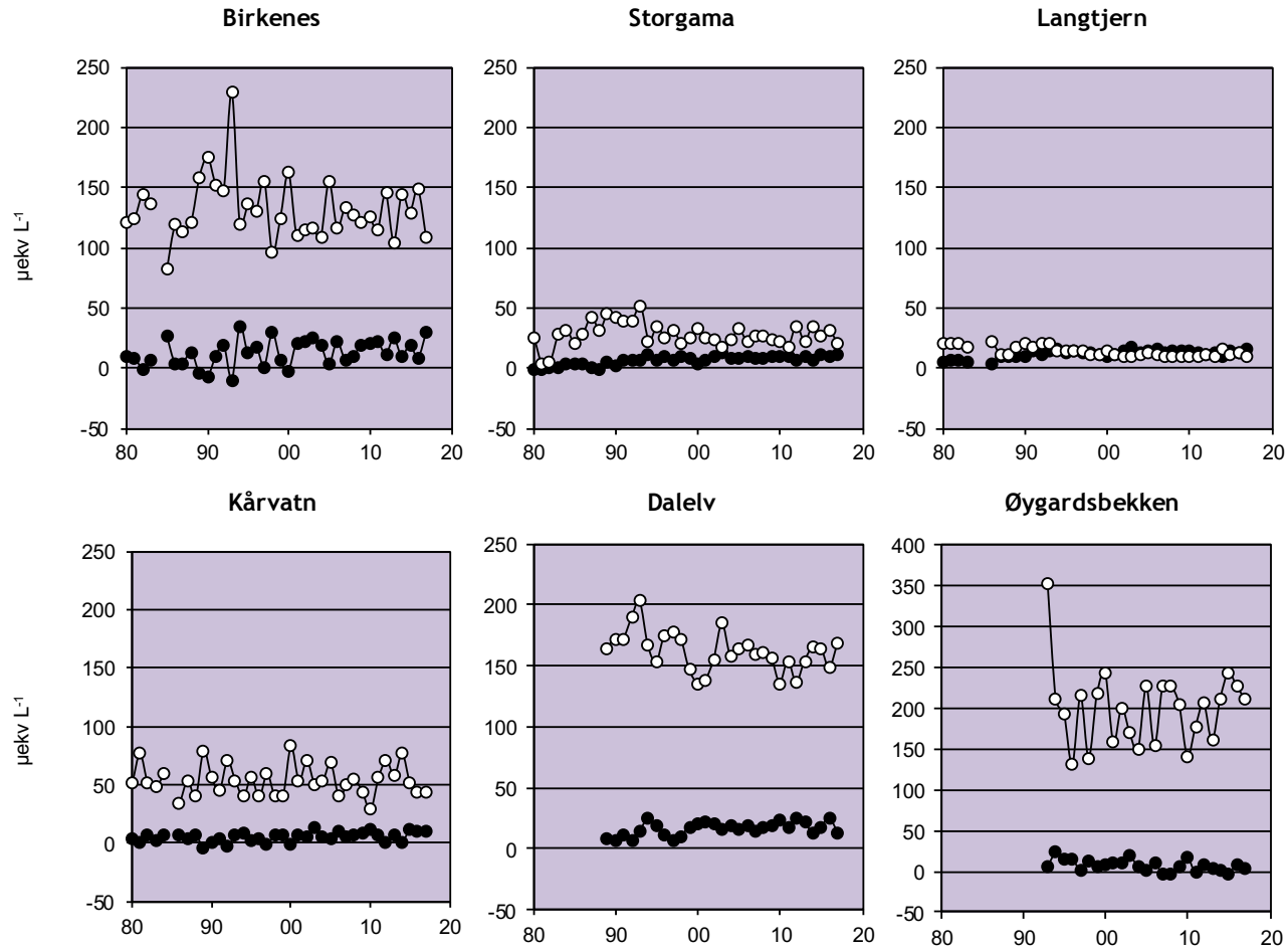
Figur 23. Trender for volumveid konsentrasjon klorid og ikke-marin natrium for feltforskningsstasjonene for perioden 1980-2017. Ikke-marin natrium ● og klorid ○. Enhet: \mu\text{ekv L}^{-1} . NB! Skala Øygardsbekken
