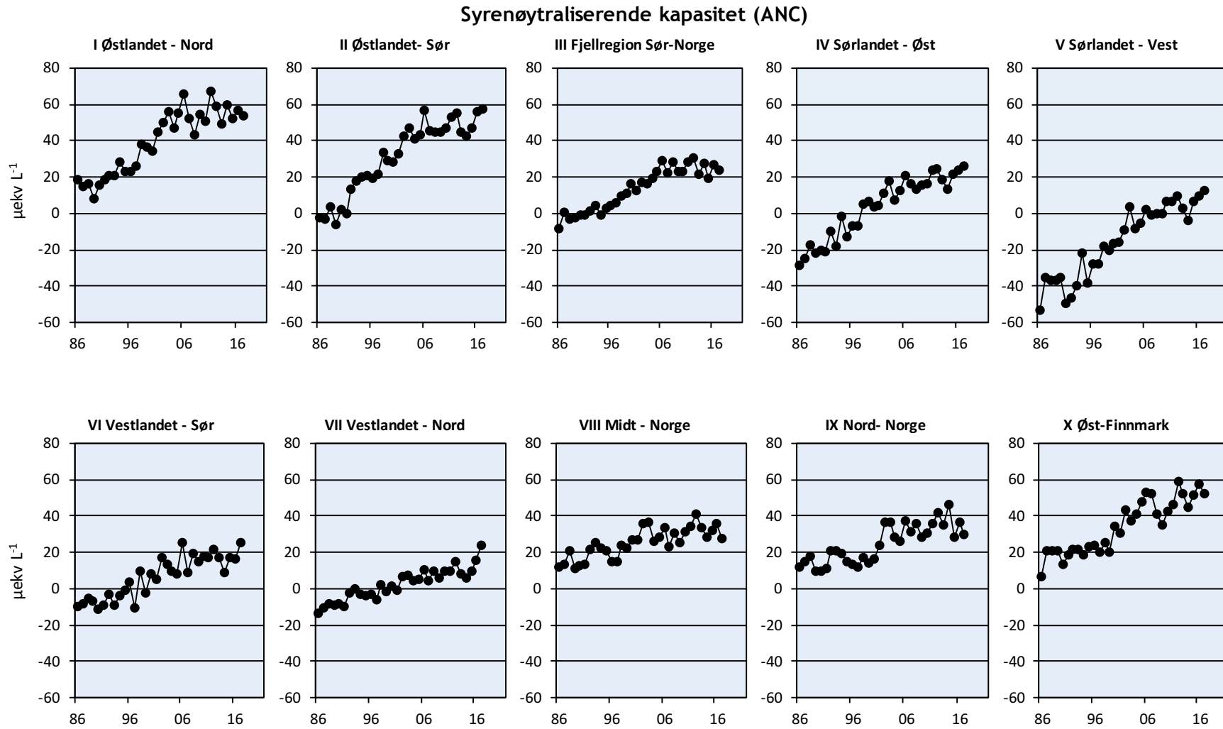
Figur 6. Trender for syrenøytraliserende kapasitet (ANC) for innsjøer i de 10 regionene for perioden 1986-2017. Enhet: \mu\text{ekv L}^{-1} .
