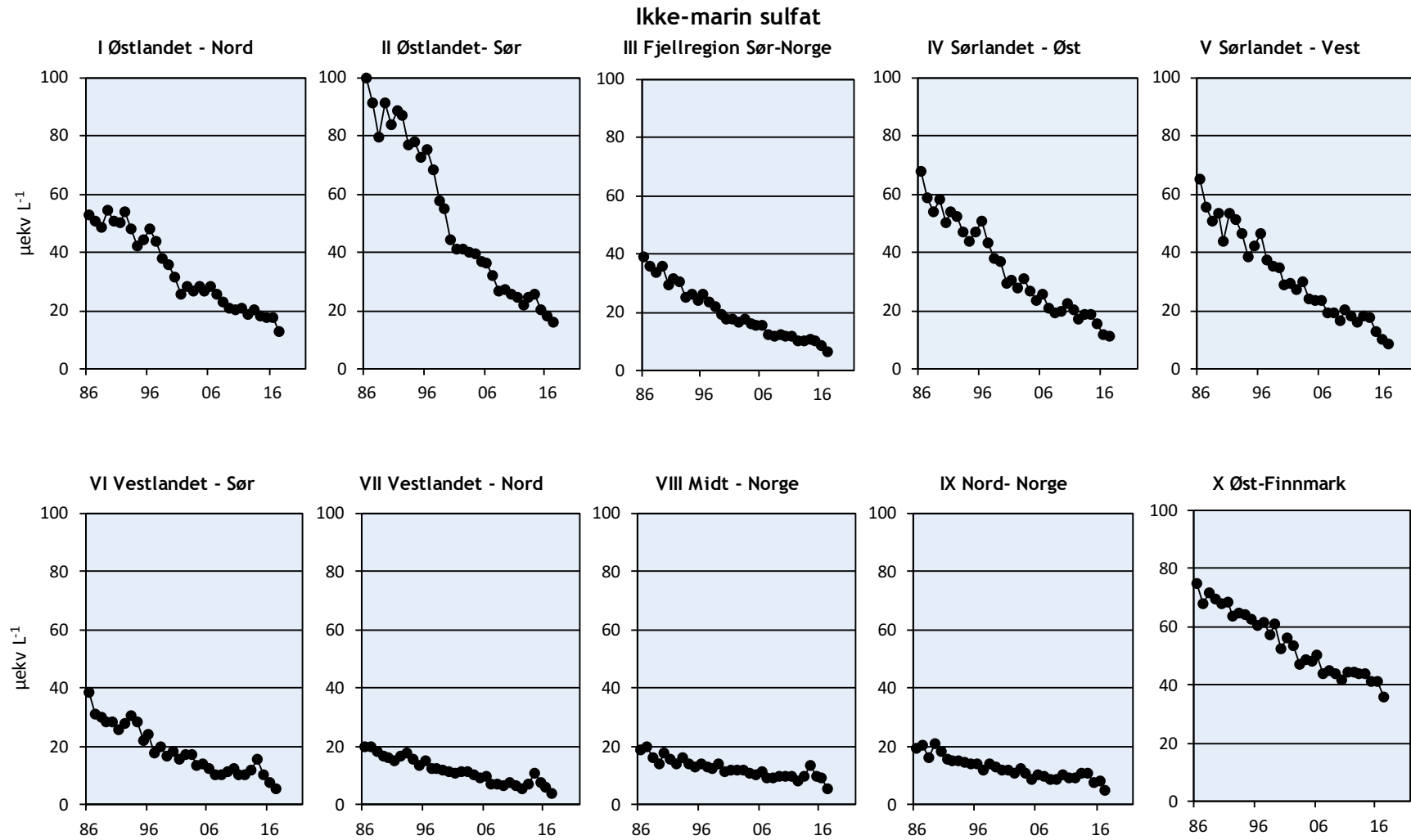
Figur 4. Trender for ikke-marin sulfat ( \text{SO}_4^* ) for innsjøer i de 10 regionene for perioden 1986-2017. Enhet: \mu\text{ekv L}^{-1} .
