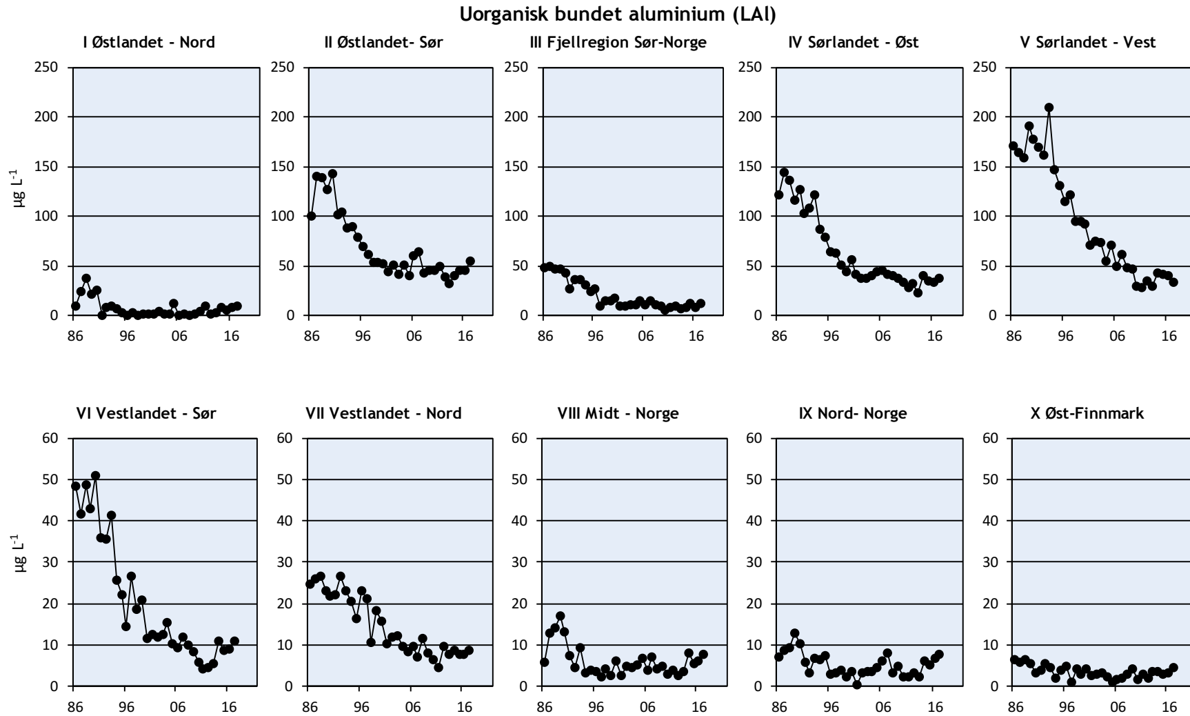
Figur 9. Trender for labilt uorganisk (bundet) aluminium (LAI) for innsjøer i de 10 regionene for perioden 1986-2017. NB! Ulik inndeling på y-aksene. Enhet: \mu\text{g L}^{-1} .
