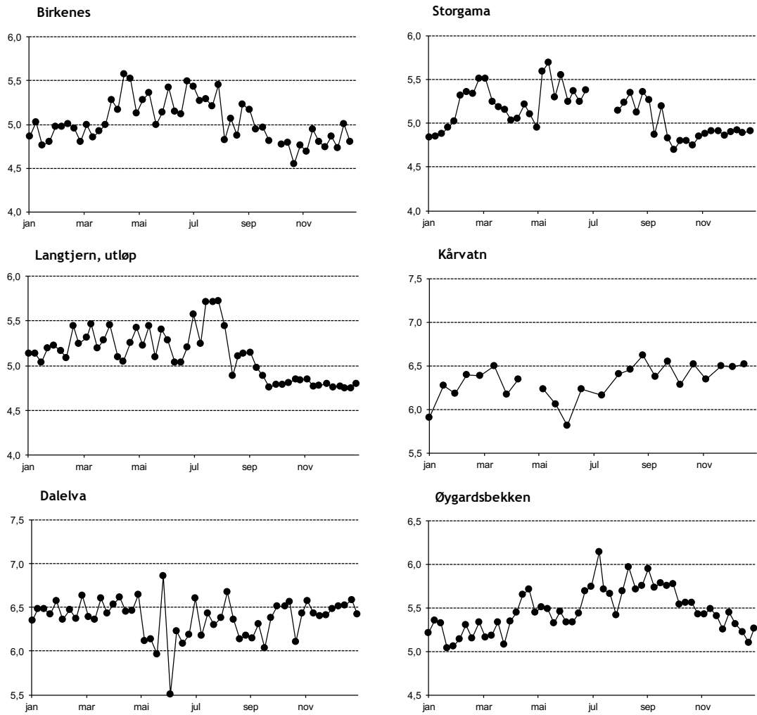
Figur 14. Sesongmessig fordeling av pH på feltforskningsstasjonene i 2017. NB! Ulik skala på y-aksene.
