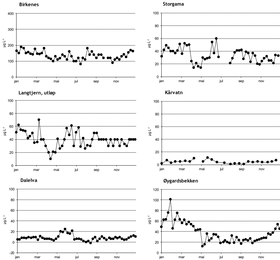
Figur 15. Sesongmessig fordeling av labilt uorganisk (bundet) aluminium (LAI) på feltforskningsstasjonene i 2017. NB! Ulik skala på y-aksene. Enhet: \mu\text{g L}^{-1} .
