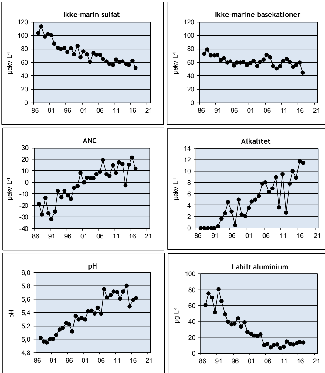
Figur 11. Forsuringsparametere for seks små vann på Jarfjordfjellet for perioden 1987-2017. Middelerverdier for ikke-marin sulfat ( SO_4^* ), ikke-marine basekationer ( Ca+Mg^* ), syrenøytraliserende kapasitet (ANC), alkalitet, pH og labilt aluminium.
