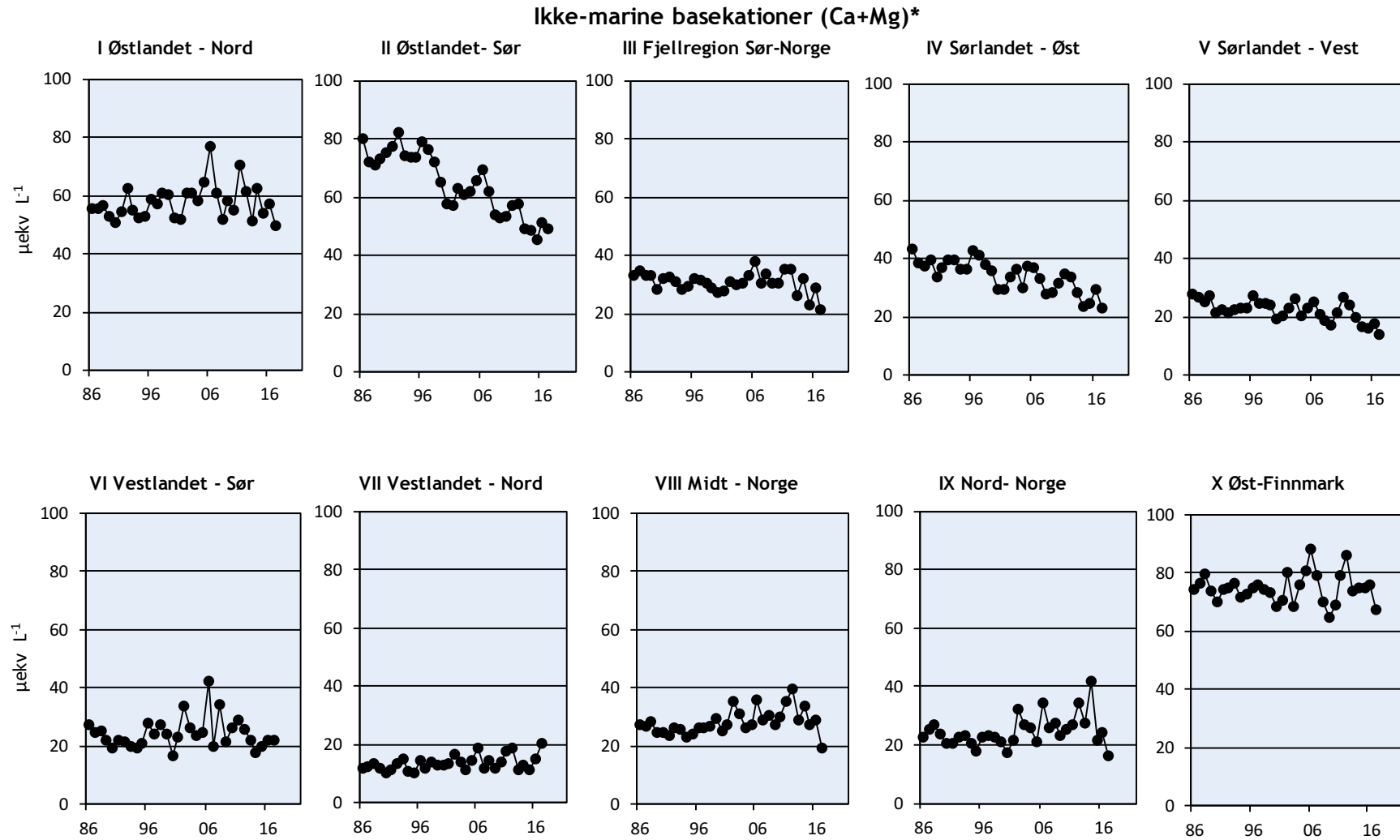
Figur 7. Trender for ikke-marine basekationer (Ca+Mg)* for innsjøer i de 10 regionene for perioden 1986-2017. Enhet: \mu\text{ekv L}^{-1} .
