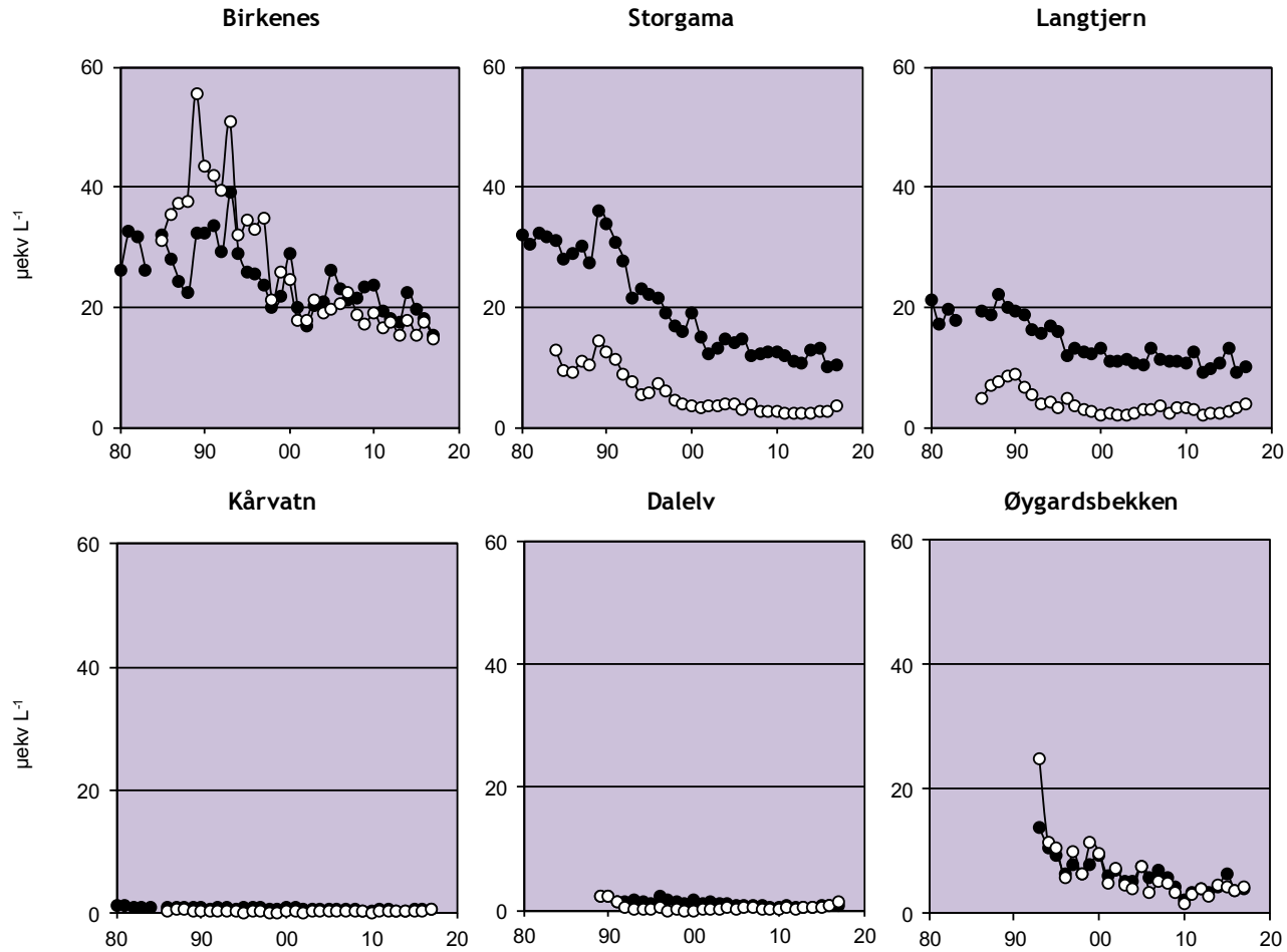
Figur 22. Trender for volumveid H + og labilt uorganisk (bundet) aluminium (LAI) for feltforskningsstasjonene for perioden 1980-2017. H + ● og labilt Al ○. Enhet: µekv L -1 .
