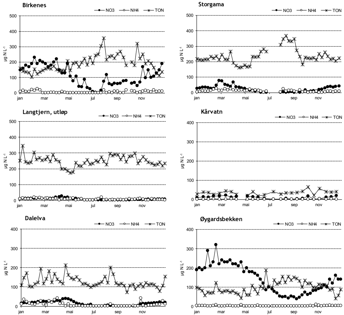
Figur 19. Sesongmessig fordeling av nitrat (NO 3 ), ammonium (NH 4 ) og totalt organisk nitrogen (TON) på feltforskningsstasjonene i 2017. TON = total nitrogen - NO 3 - NH 4 . NB! Ulik skala på y-aksene. Enhet: µg N L -1 .
