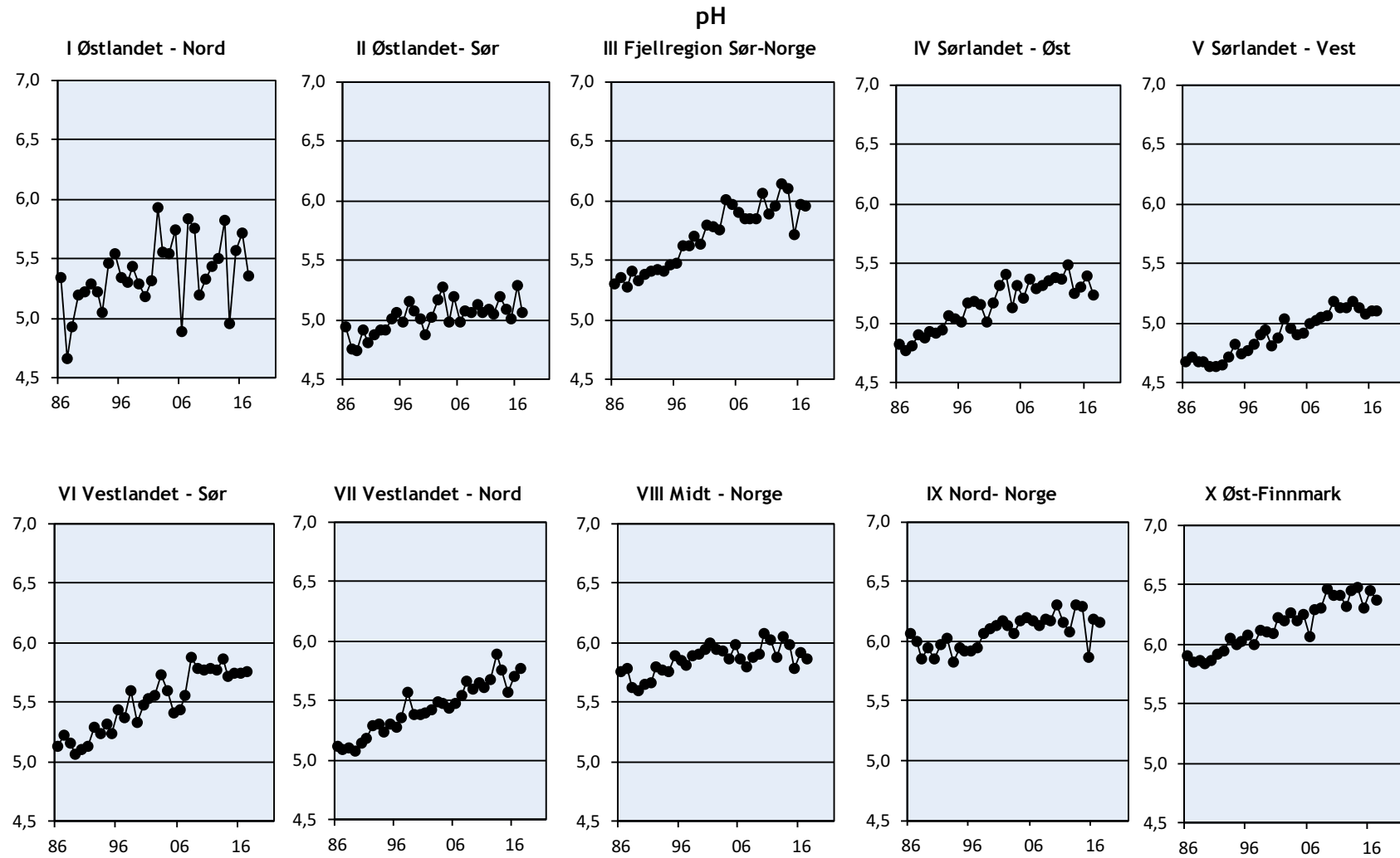
Figur 8. Trender for pH for innsjøer i de 10 regionene for perioden 1986-2017.
