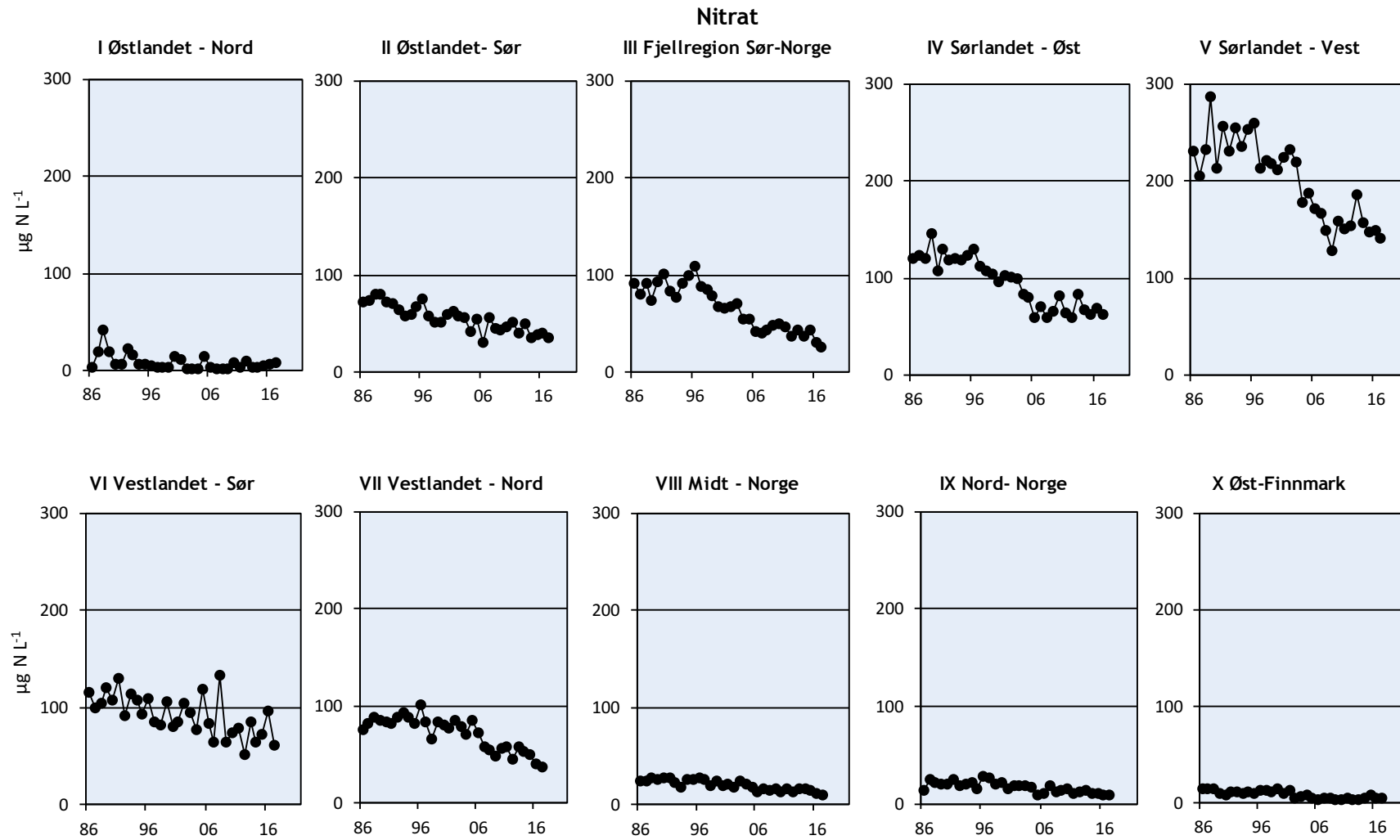
Figur 5. Trender for nitrat for innsjøer i de 10 regionene for perioden 1986-2017. Enhet: \mu\text{g N L}^{-1} .
