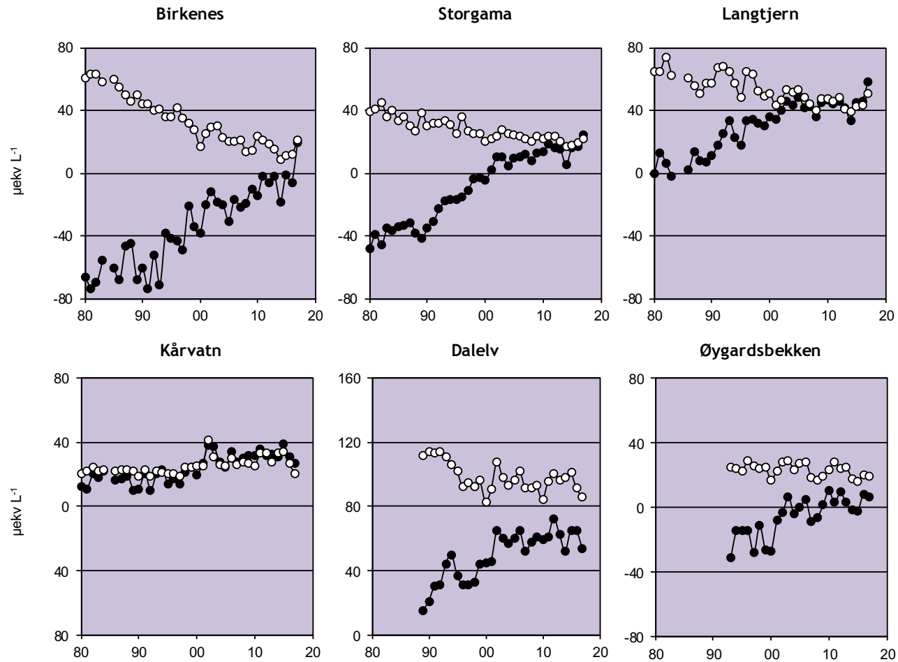
Figur 21. Trender for volumveid syrenøytraliserende kapasitet (ANC) og ikke-marine basekationer (Ca+Mg)* for feltforskningsstasjonene for perioden 1980-2017. ANC ● og ikke-marine basekationer (Ca+Mg)* ○. Enhet: \mu\text{ekv L}^{-1} . NB! Skala Dalelv.
