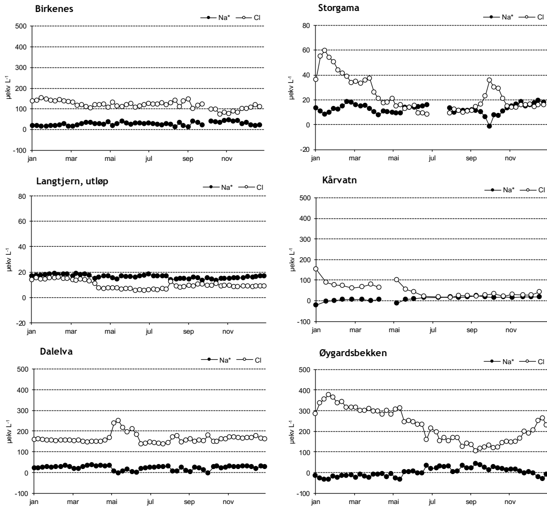
Figur 16. Sesongmessig fordeling av klorid og beregnet ikke-marin natrium på feltforskningsstasjonene i 2017. Ikke-marin natrium ● og klorid ○. NB! Uluk skala på y-aksene. Enhet: \mu\text{ekv L}^{-1} . Negativ ikke-marin natrium tolkes som at natrium holdes tilbake i nedbørfeltet og erstattes av andre ioner i avrenningen.
