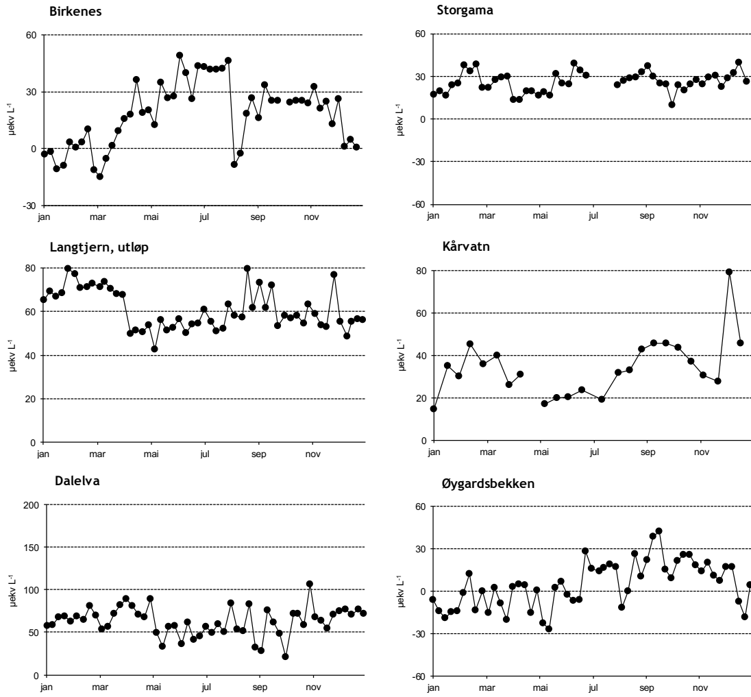
Figur 17. Sesongmessig fordeling av syrenøytraliserende kapasitet (ANC) på feltforskningsstasjonene i 2017. NB! Ulik skala på y-aksene. Enhet: \mu\text{ekv L}^{-1} .
