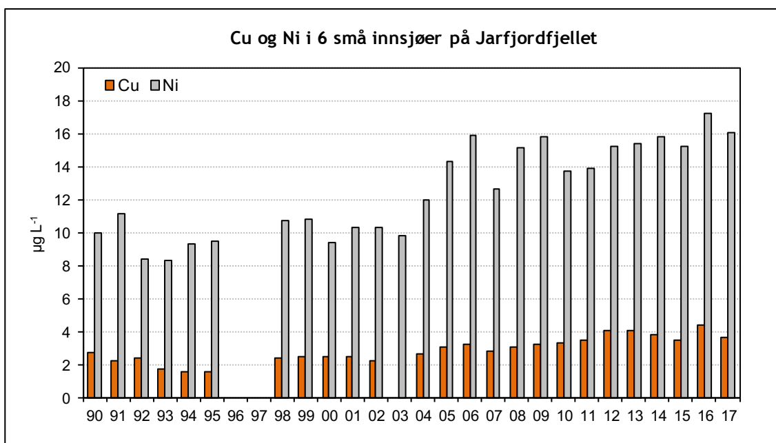
Figur 12. Årlige middelverdier for kobber og nikkel i seks små innsjøer på Jarfjordfjellet for perioden 1990-2017.
