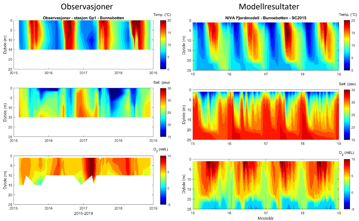
Figur 23. Temperatur, saltholdighet og oksygen i Bunneboten. Til venstre vises målinger fra stasjon Gp1, og til høyre vises modellresultater fra NFM, scenarier SC2015.
