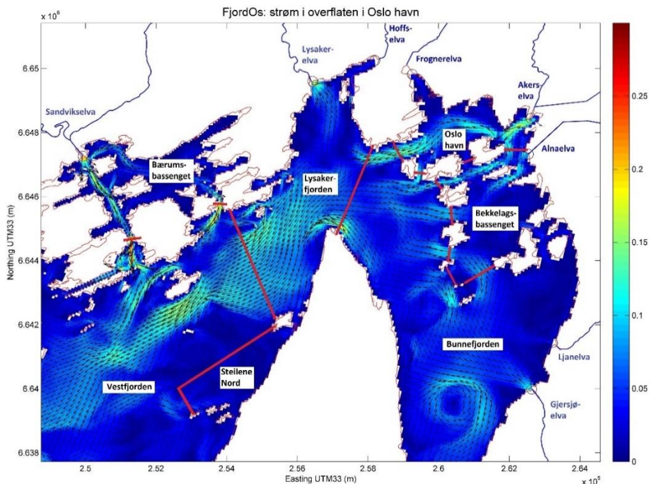
Figur 3. Et øyeblikksbilde som viser strømsituasjonen i overflaten i Oslofjorden, hvor strømmen er beregnet med 3D-modellen FjordOs. Fargeskalaen angir strømstyrken i m/s, og pilene viser strømretningen. De røde strekkene viser hvilke bassenger som boks-modellen NFM bruker for å beskrive denne delen av fjorden.
