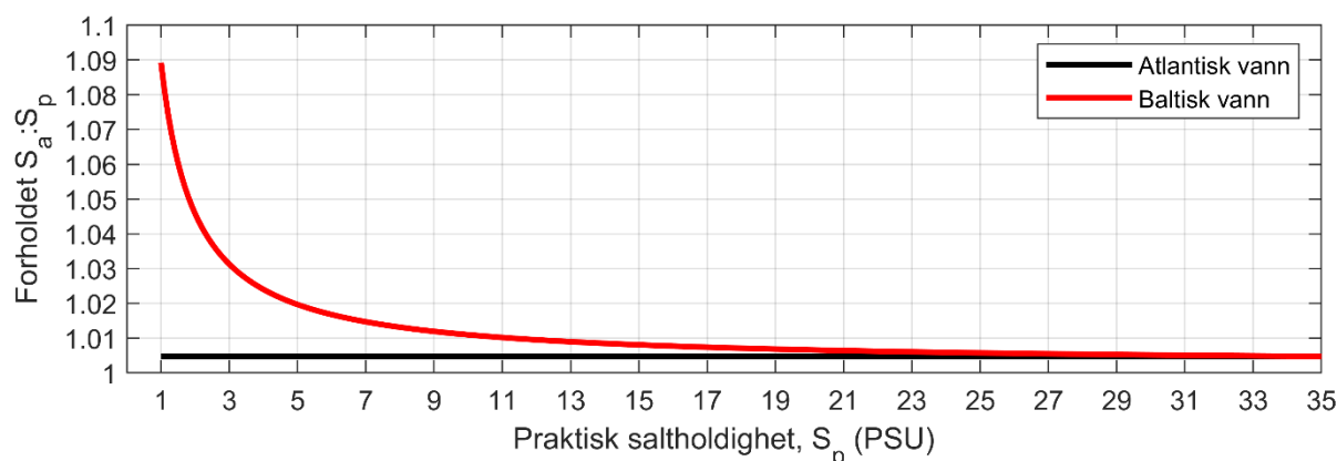
Figur 2. Forholdet mellom absolutt saltholdighet målt i tusendeler ( \text{g/kg} ) og praktisk saltholdighet målt i PSU. Grafen gjelder for Indre Oslofjord.
