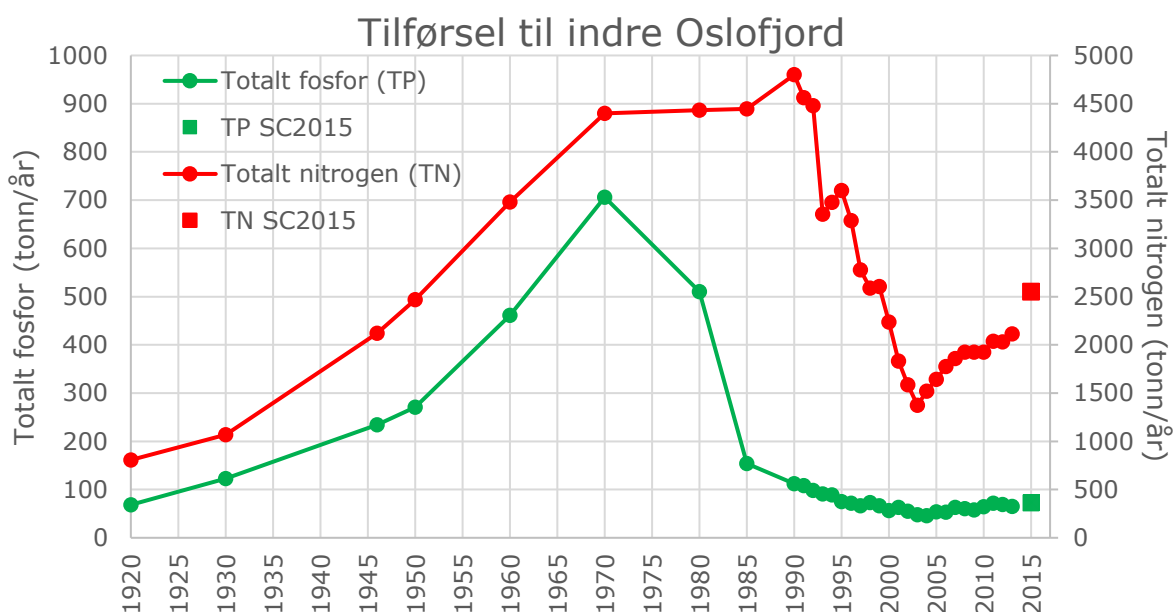
Figur 1. Tilførsel til Indre Oslofjord. Data fra 1985 og 1990 til 2013 er hentet fra Berge et al. (2015). Data fra 1920-1980 er hentet fra Bergestøl et al. (1981). Verdiene som er lagt inn i modellen i scenariet SC2015 er markert med grønn og rød firkant.
