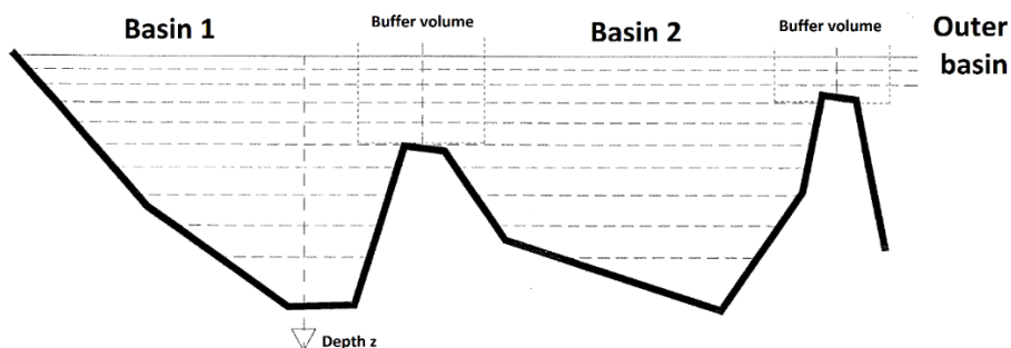
Figur 4. En skjematisk illustrasjon av hvordan en boks-modell kan beskrive en fjord som har to bassenger som står i forbindelse med et ytre basseng, hvor bassengene er adskilt av terskler. Boks-modellen må beregne hvordan vannet utveksles mellom disse bassengene.
