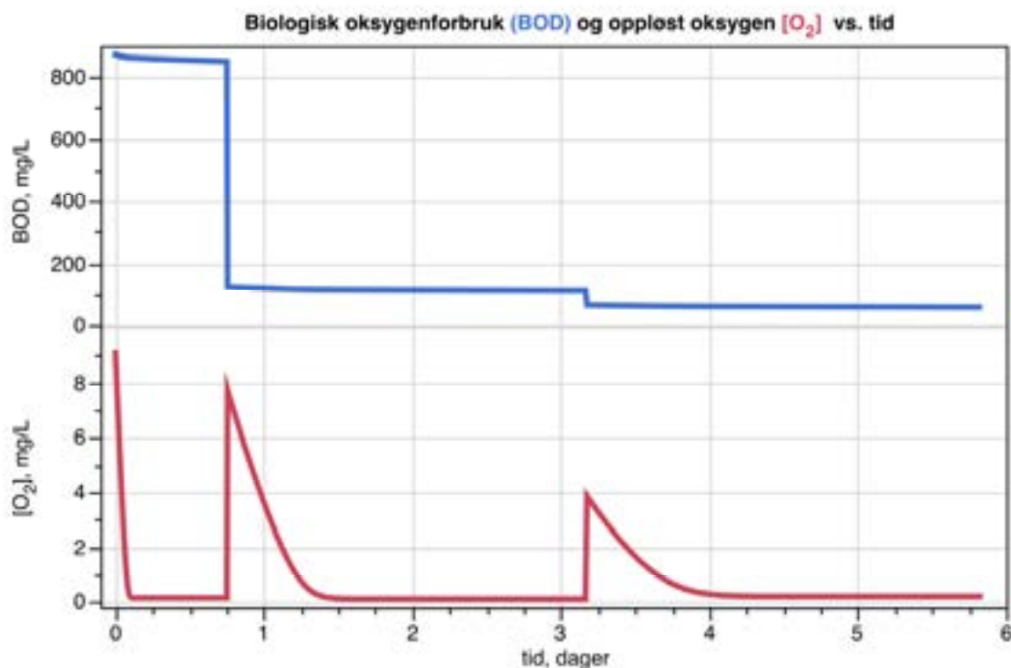
Figur 9. Konsentrasjonen oppløst oksygen [O_2] og organisk materiale målt som biologisk oksygenforbruk i vann (BOD, mg O_2/l ) i Aulivassdraget etter tilførsel av brannskum fra slukkingen ved Revac AS. Konsentrasjonene er modellert for et avgrenset vannvolum som renner nedover vassdraget. Vassdraget er inndelt i tre ulike elveavsnitt, og tilførselen av uforurenset vann fra sidevassdragene Storelva og Merkedamselva fører til lokale bedringer i oksygenforholdene og fortynning av forurensingene (reduisert BOD).
