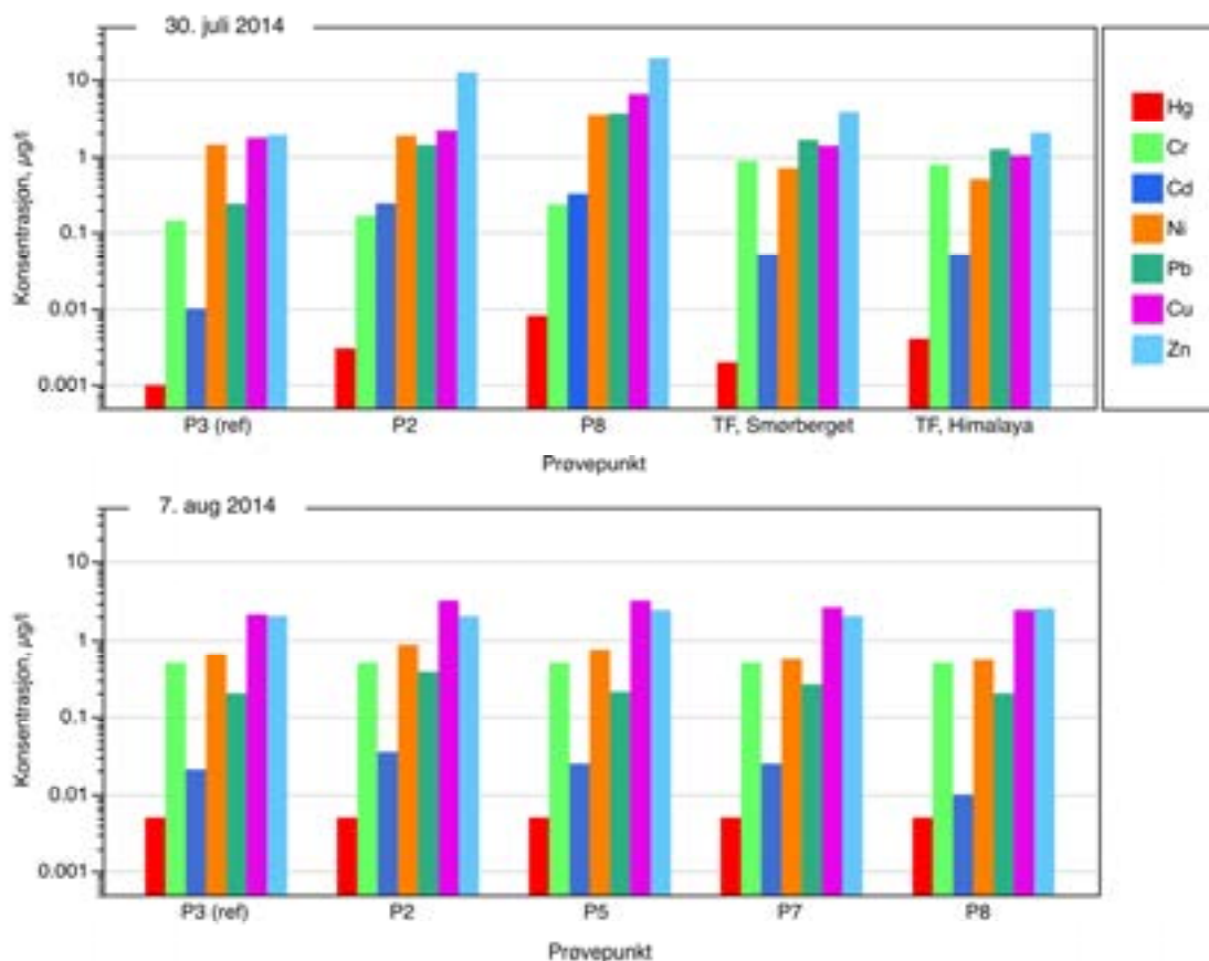
Figur 6. Konsentrasjoner av tungmetaller i vannprøver tatt i Aulivassdraget og Tønsbergfjorden (prøvepunktene merket TF) 30. juli og 7. august av NIVA. Det analysert på henholdsvis ufiltrerte (30. juli) og filtrerte prøver (7. august). Ytterligere resultater fra syreoppløstede prøver (7. august) finnes i Tabell 2. Verdier under kvantifikasjonsgrensen satt like grensen. Prøvene fra Aulivassdraget er merket P2–P8 (Figur 3). Prøvene fra Tønsbergfjorden er merket TF (Smørberget: nær utløpet av vassdraget; Himalaya: ved Melsomvik).
