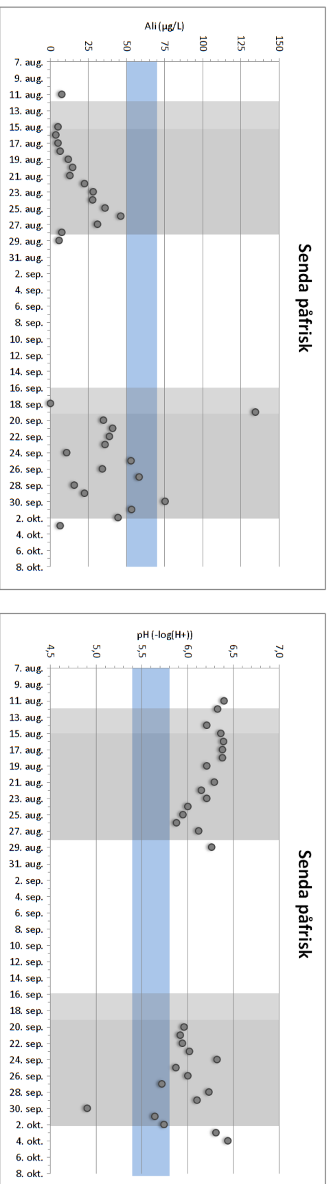
Figur A9. Konsentrasjon av labilt aluminium (Al i ) og pH i prøver fra Senda oppstrøms (referanse) og Senda påfrisk tatt i 2011. Behandlingsperiodene er markert med grått. Vannkjemiske målområder er markert med blått.
