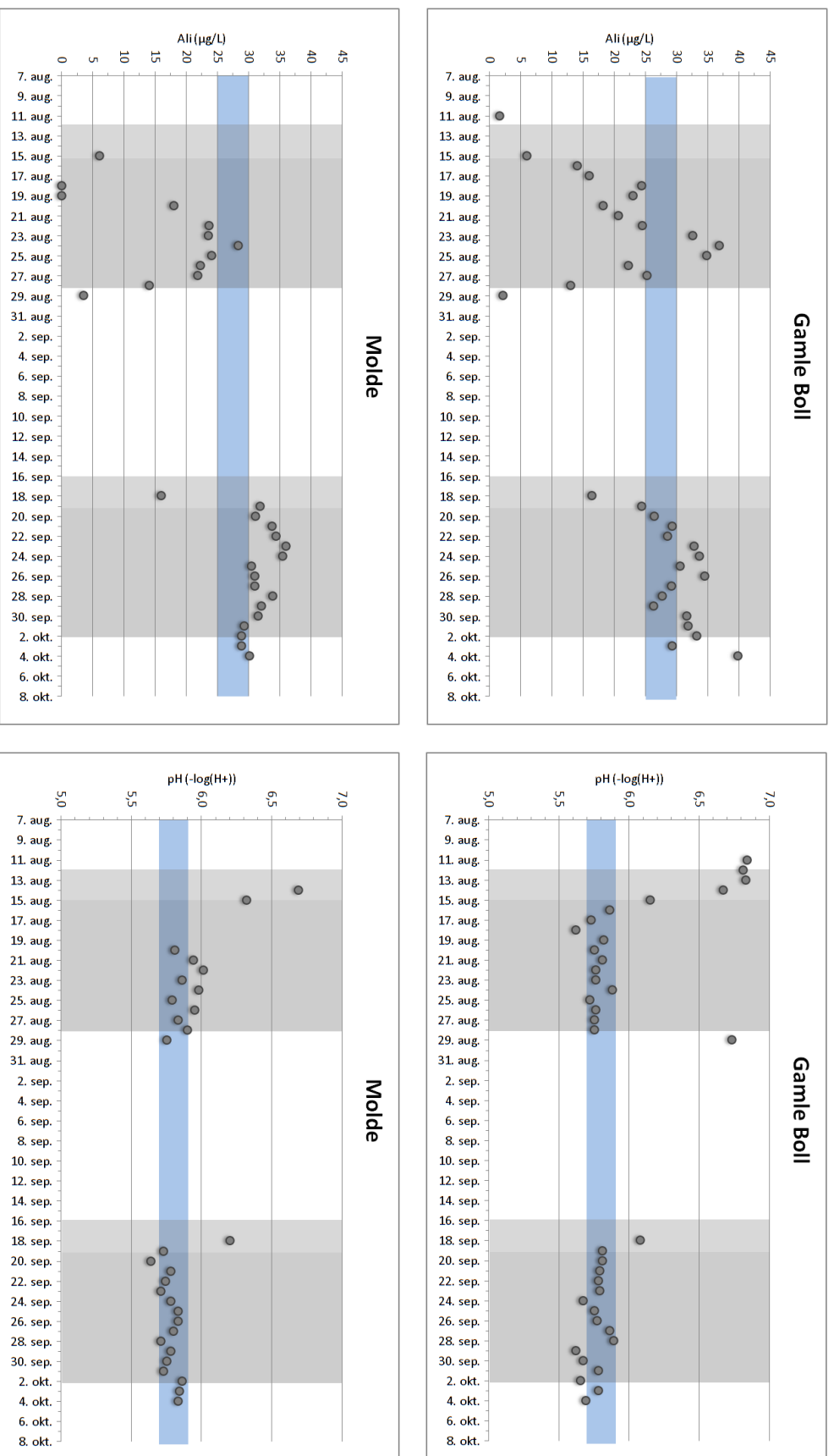
Figur A5. Konsentrasjon av labilt aluminium (Al i ) og pH i prøver fra Gamle Boll og Molde tatt i 2011. Behandlingsperiodene er markert med grått. Vannkjemiske målområder er markert med blått.
