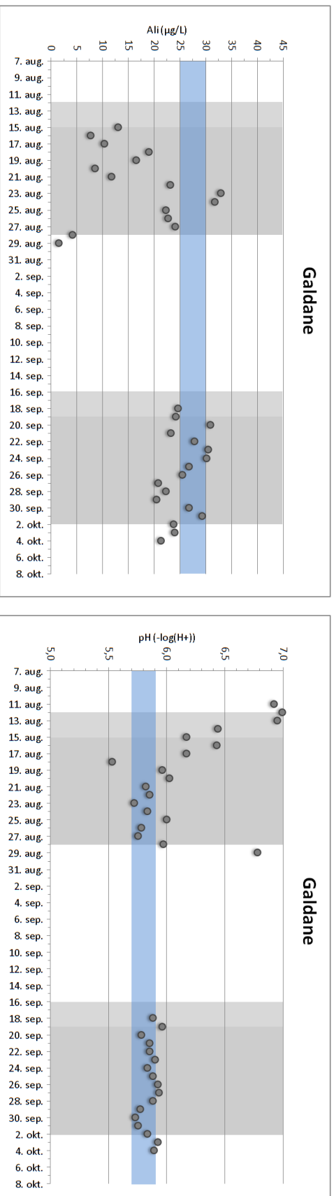
Figur A1. Konsentrasjon av labilt aluminium (Ali) og pH i prøver fra Sjurhaug oppstrøms (referanse) og Galdane tatt i 2011. Behandlingsperiodene er markert med grått. Vanntkjemiske målområder er markert med blått.
