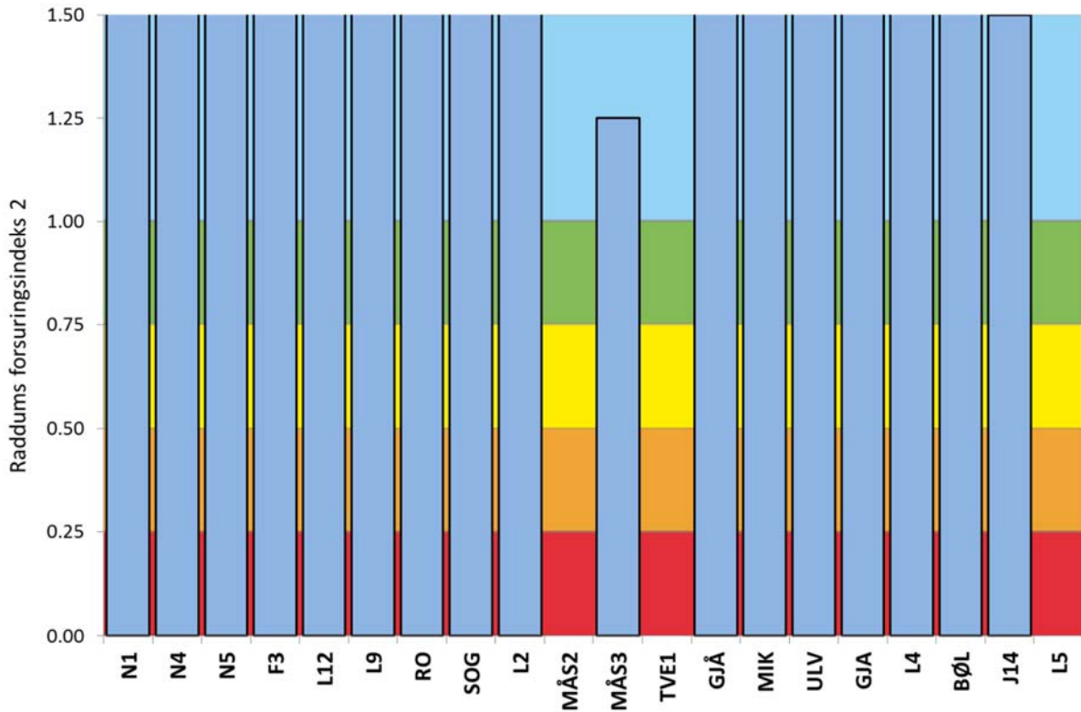
Figur 8. Forsuringsindeksen Raddum 2.
