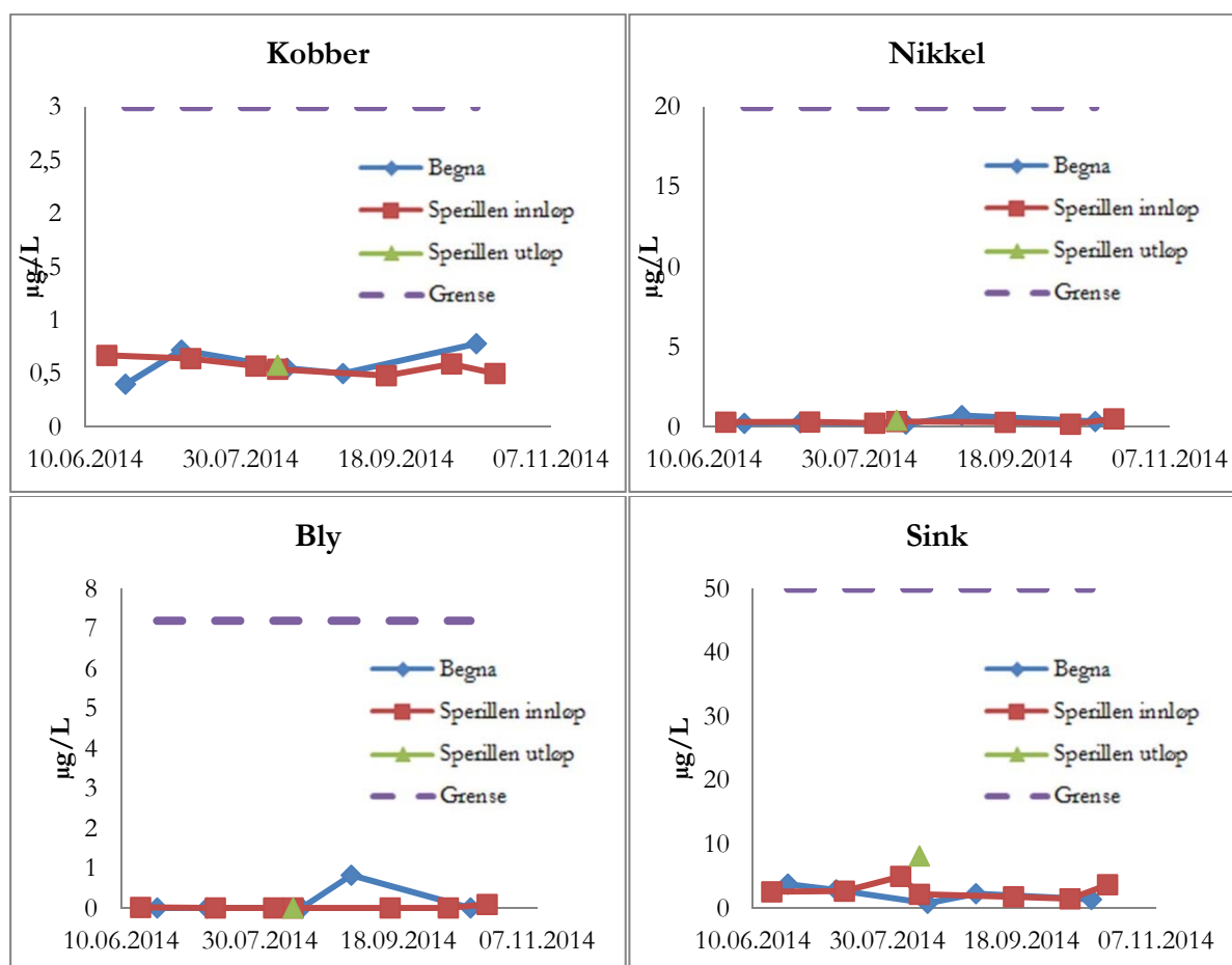
Figur 6. Metallkonsentrasjoner (µg/L) målt ved Begna nedstrøms Bagn, og innløp og utløp i Sperillen. Grenseverdien mellom god og dårlig tilstand er markert med stiplet linje.
