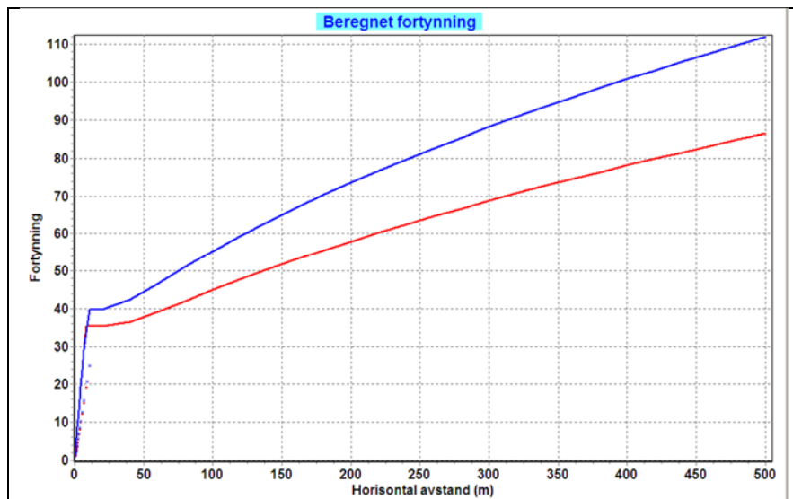
Figur 18. Beregning for en vertikalprofil målt 16.3.1984. Vannmengde 920 m 3 /h og temperaturøkning 15 °C. Rød kurve: utslipp gjennom diffusor med 15 hull. Blå kurve: utslipp gjennom diffusor med 9 hull.
