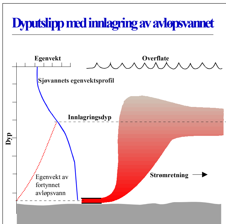
Figur 14. Prinsippskisse som viser hvordan et dyputslipp av avløpsvann fungerer i forhold til innlagring. En forutsetning for innlagring er at egenvekten for fjordvannet øker med dypet (vertikal stabil sjiktning).
