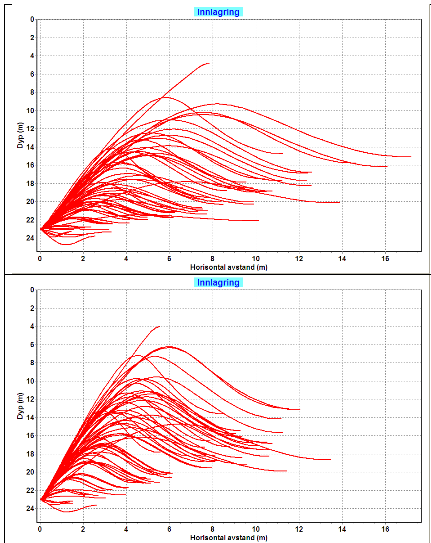
Figur 15. Beregningen av innlagringsdyp for avløpsvannet ved utslipp i 23 m dyp. Strømhastighet 3 cm/s. Øverst ved temperaturøkning 10 °C og nederst ved temperaturøkning 15 °C.
