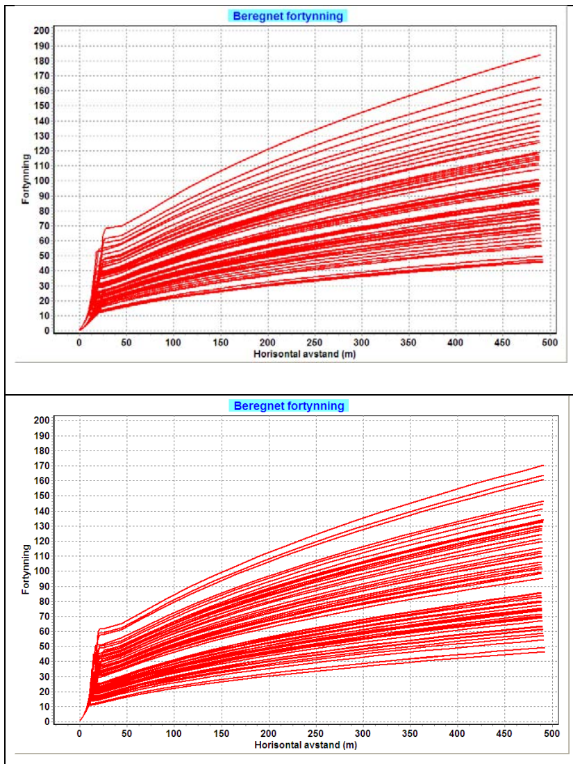
Figur 16. Beregnet fortynning av avløpsvannet for de 60 situasjonene og ved strømhastighet 3 cm/s. Øverst ved temperaturøkning 10 °C og nederst ved temperaturøkning 15 °C.
