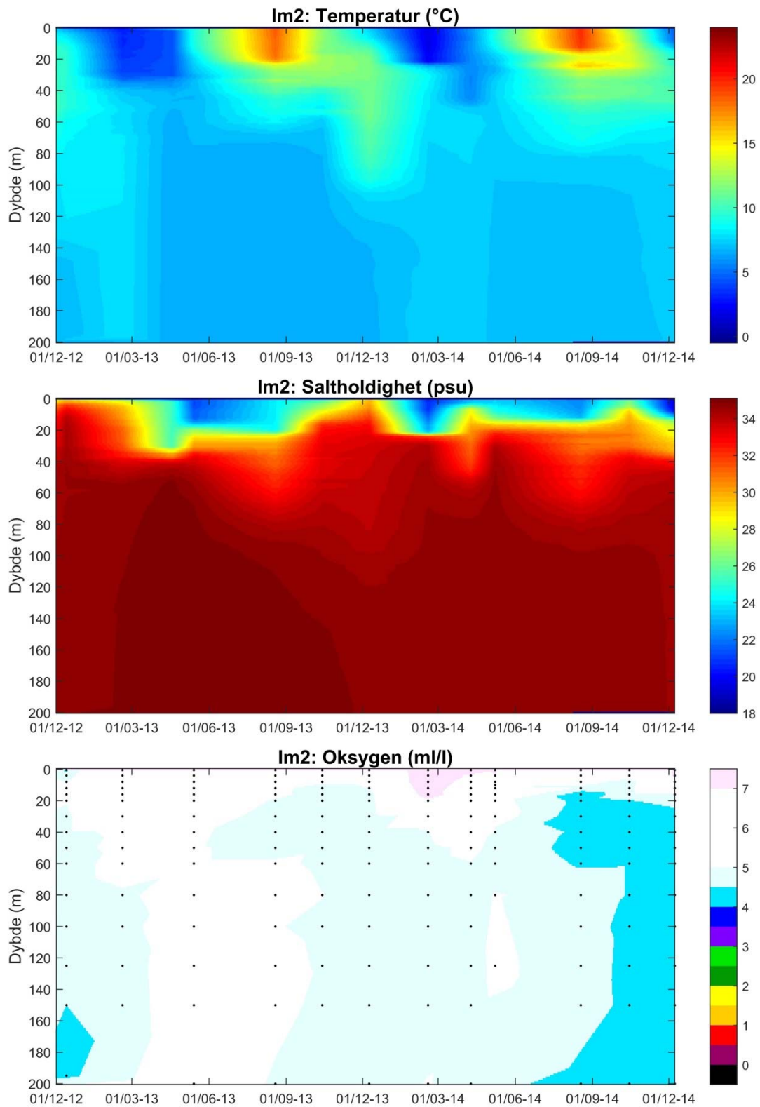
Figur 7. Hydrografisk utvikling i ulike dyp i Drøbaksundet utenfor Drøbakerskelen fra desember 2012 til desember 2014. Øverst vises temperatur, i midten saltholdighet og nederst oksygenkonsentrasjonen.
