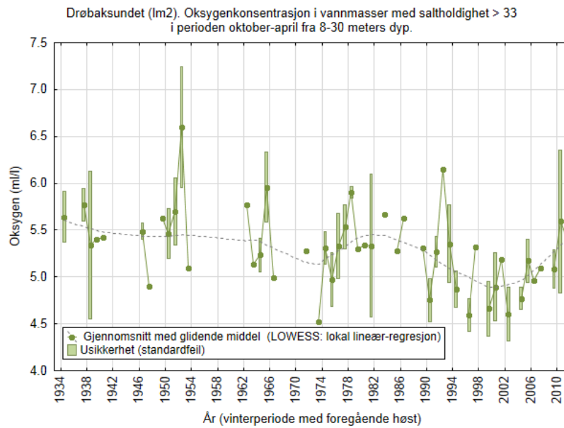
Figur 5. Oksygen (ml/l) i Drøbaksundet (1m2) fra 1933-2011 i vannmasser som kan danne nytt dypvann i Indre Oslofjord. Data fra Braarud og Ruud 1937, Dannevig 1945, Beyer og Føyn 1951, Havforskningsinstituttet (1952-61) og NIVA (1962-2011). Det er først beregnet middelvei for hver dato av observasjoner som oppfyller utvalgsriteriet, deretter er det beregnet enkelt gjennomsnitt uten vektning over datogjennomsnittene innenfor hver vinterperiode fra oktober til april. Årstall gjelder månedene januar-april, men hver vinterperiode omfatter også data fra oktober-desember året før. For perioden oktober 2011 til april 2012 og oktober 2012 til april 2013 var det ikke noe vann som passet inn i kriteriet saltholdighet > 33 ved 8 til 30 meters dyp.
