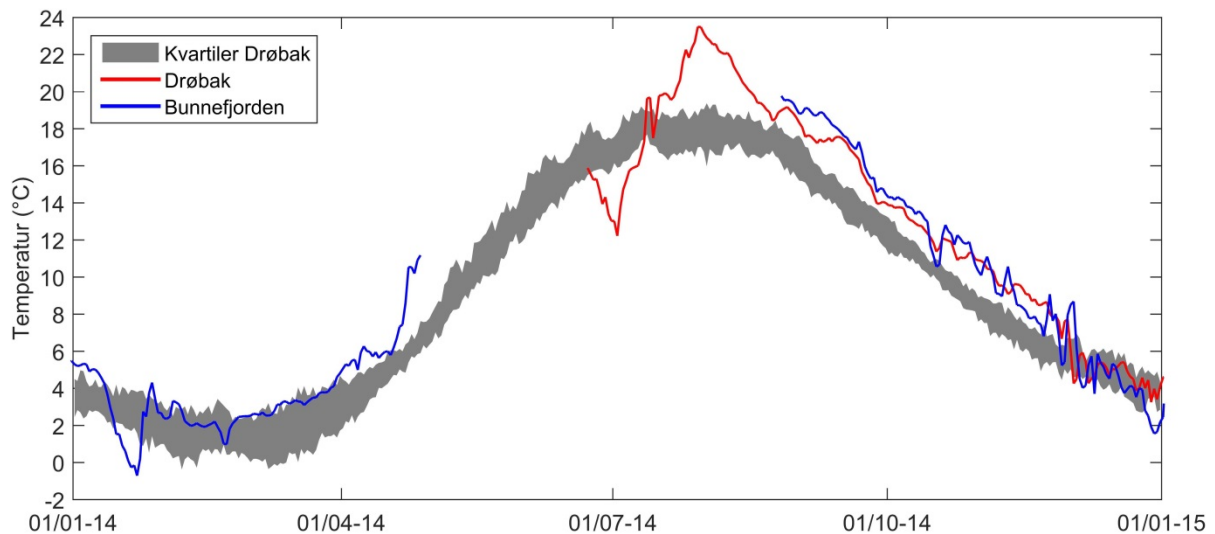
Figur 20. Termometermålinger (døgnmiddel) i 1 m dyp ved Biologisk stasjon i Drøbak og i Bunnefjorden sør for Bekkensten for perioden januar 2012 til desember 2012. I figuren er også daglige observasjoner i 1 m dyp fra Drøbak for perioden 1967-1993 lagt inn (innsamlet av tidligere bestyrer Walvig på Biologisk Stasjon i Drøbak).
