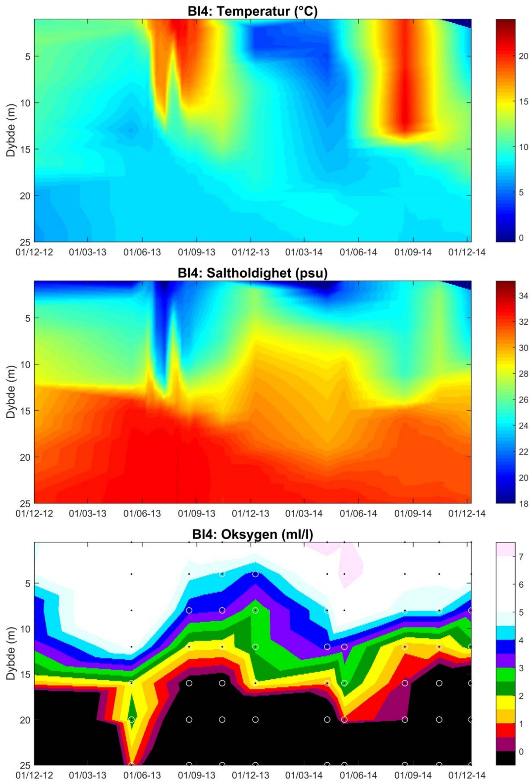
Figur 11. Hydrografisk utvikling i Bærumsbassenget fra desember 2012 til desember 2014. Øverst vises temperatur, i midten saltholdighet og nederst oksygenkonsentrasjonen.
