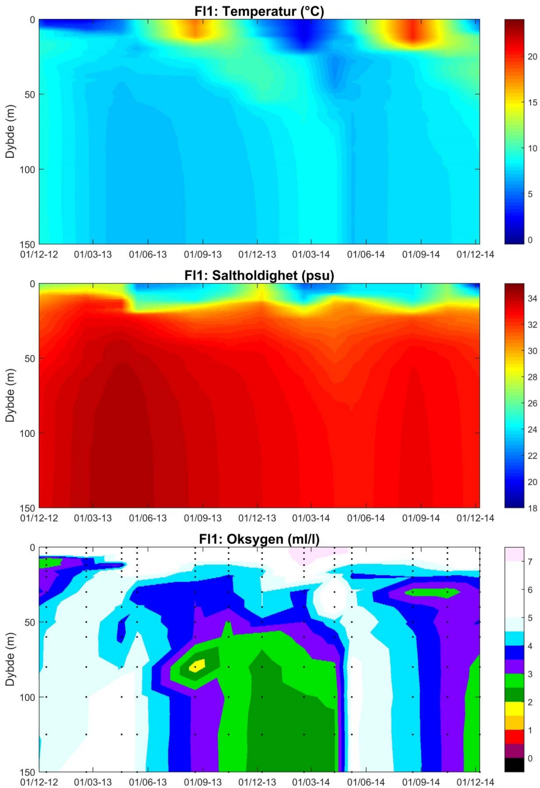
Figur 9. Hydrografisk utvikling ved Søndre Langåra fra desember 2012 til desember 2014. Øverst vises temperatur, i midten saltholdighet og nederst oksygenkonsentrasjonen.
