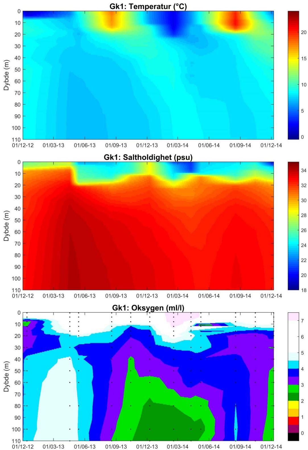
Figur 8. Hydrografisk utvikling i Gråøyrenna vest for Håøya fra desember 2012 til desember 2014. Øverst vises temperatur, i midten saltholdighet og nederst oksygenkonsentrasjonen.
