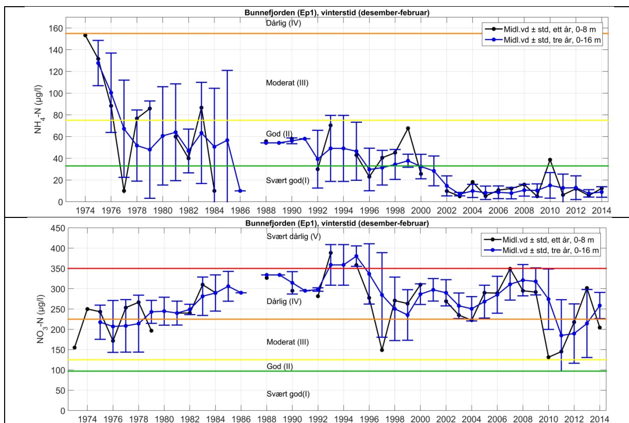
Figur 29. Vinterobservasjoner av \text{NH}_4\text{-N} (øverste panel) og \text{NO}_3\text{-N} + \text{NO}_2\text{-N} (nederste panel) i Bunnefjorden (Ep1). For detaljert forklaring, se i Figur 26
