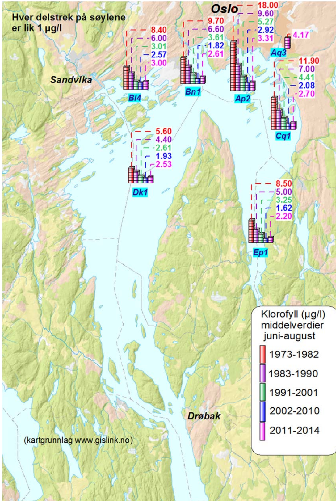
Figur 25. Klorofyll a (µg/l) i 0-2 meters dyp, middelværdier i juni-august fra 1973-82, 1983-90, 1991-2001, 2002-2010 og 2011-2014. Klorofyll a er et indirekte mål på planteplanktonbiomassen.
