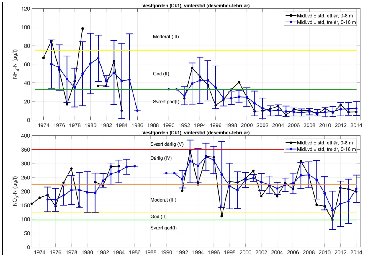
Figur 27. Vinterobservasjoner av NH 4 -N (øverste panel) og NO 3 -N+NO 2 -N (nederste panel) i Vestfjorden (Dk 1). For detaljert forklaring, se i Figur 26 .
