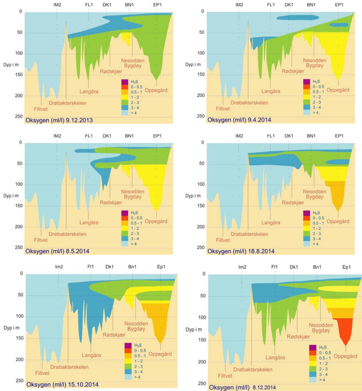
Figur 4. Oksygenvariasjonen i Indre Oslofjord fra desember 2013 til desember 2014.
