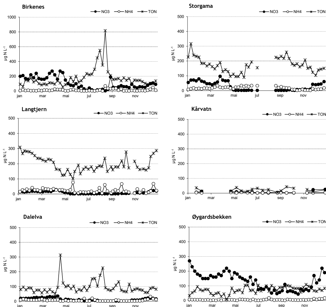
Figur 19. Sesongmessig fluktusjoner i konsentrasjonene av nitrat ( \text{NO}_3 ), ammonium ( \text{NH}_4 ) og totalt organisk nitrogen (TON) ved feltforskningsstasjonene i 2022. \text{NO}_3 ●, \text{NH}_4 ○ og TON *. Enhet: \mu\text{g N L}^{-1} . TON = totalt nitrogen – nitrat – ammonium. NB! Annen skala på y-aksen for Birkenes.
