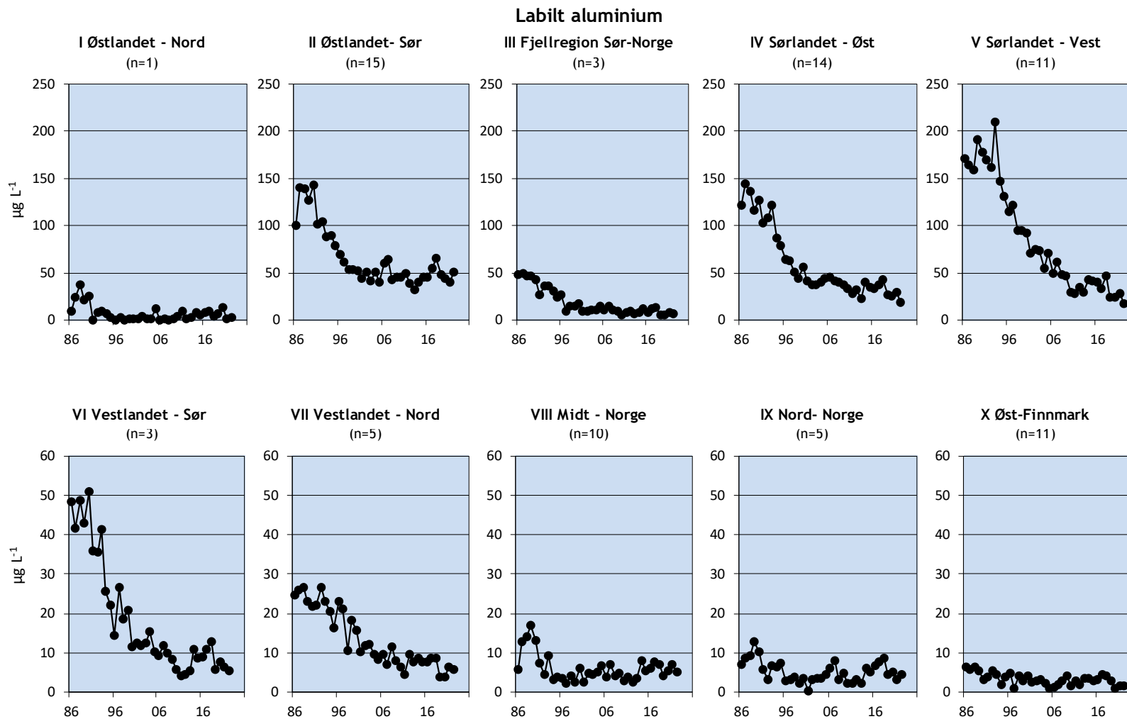
Figur 9. Årlige gjennomsnittskonsentrasjoner av labilt aluminium (LAI) i de forsureningsfølsomme innsjøene for perioden 1986-2022 fra hver av de 10 regionene beskrevet i Vedlegg 1. NB! Ulik skala på y-aksene. Enhet: \mu\text{g L}^{-1} . n angir antall innsjøer i hver region.
