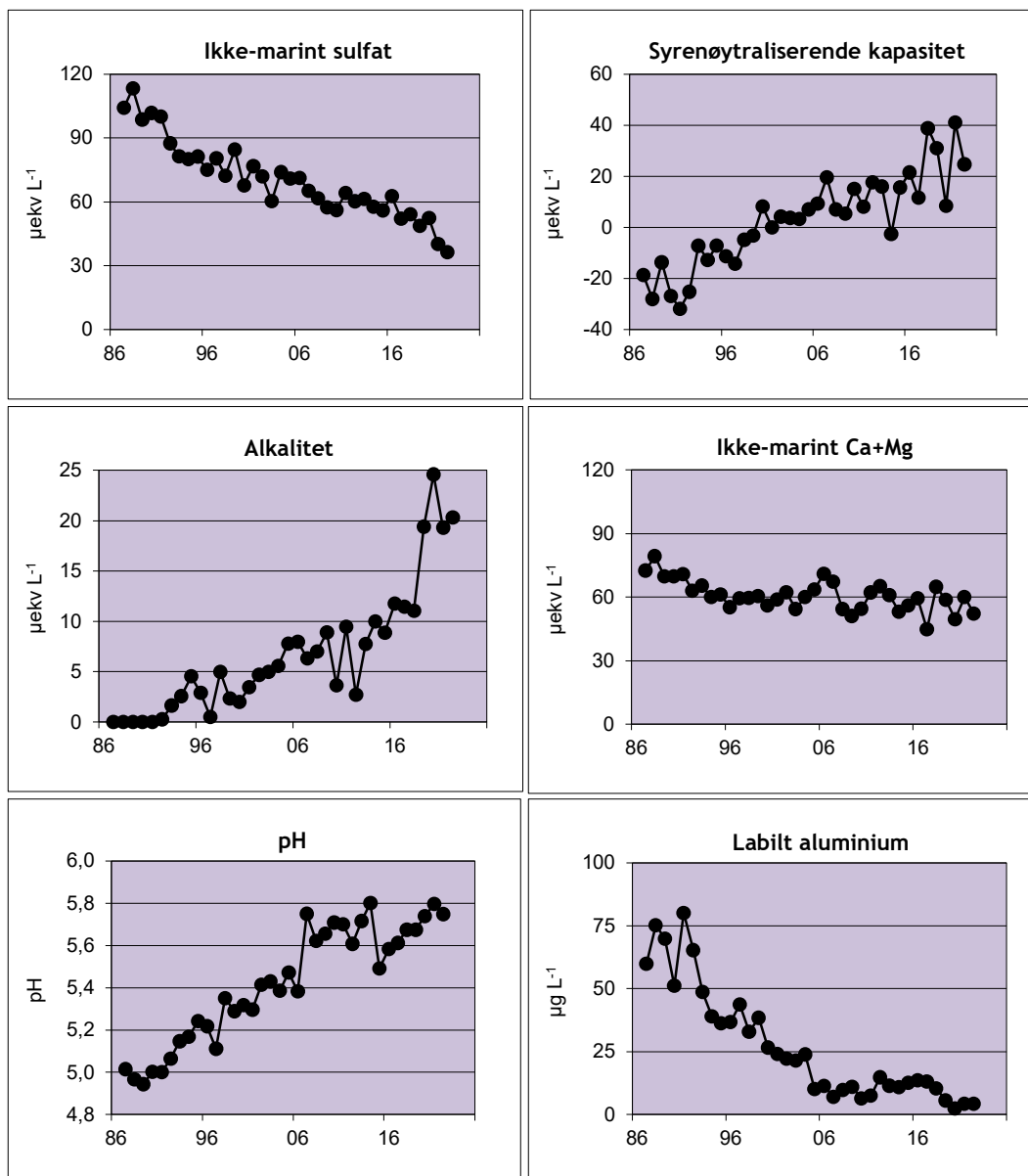
Figur 11. Forsuringsparametere for 6 små innsjøer på Jarfjordfjellet for perioden 1987-2022. Middelerverdier for ikke-marint sulfat ( \text{SO}_4^* ), syrenøytraliserende kapasitet (ANC), alkalitet, ikke-marine toverdige basekationer ( \text{Ca}+\text{Mg} )*, pH (basert på \text{H}^+ -ekvivalenter) og labilt aluminium (LAI).
