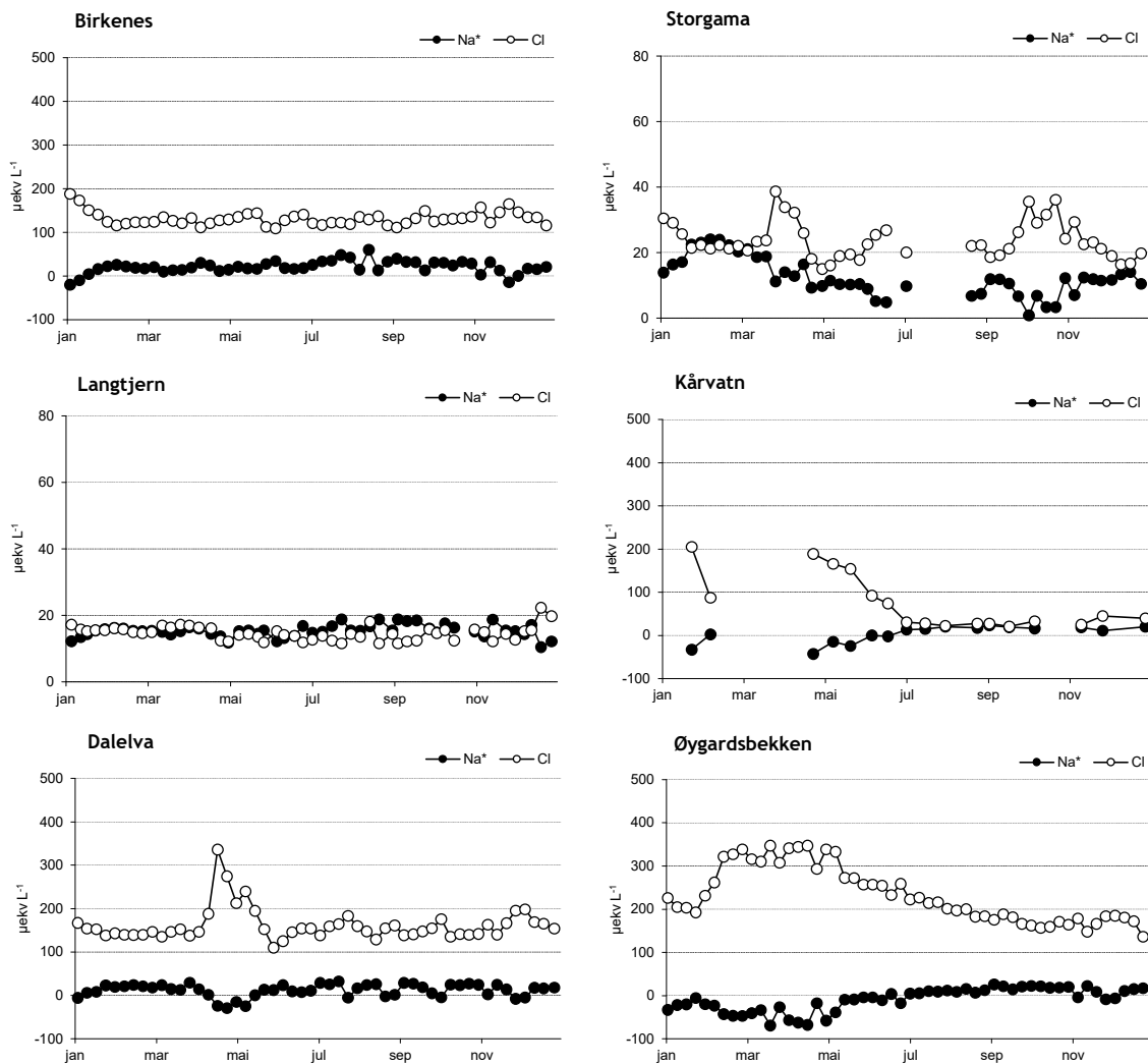
Figur 16. Sesongmessige fluktusjoner i konsentrasjonene av ikke-marint natrium ( \text{Na}^+ ) og klorid ( \text{Cl}^- ) på feltforskningsstasjonene i 2022. \text{Na}^+ ● og \text{Cl}^- ○. Enhet: \mu\text{ekv L}^{-1} . NB! Ulik skala på y-aksene. Negativ \text{Na}^+ tolkes som at natrium holdes tilbake i nedbørfeltet og erstattes av andre kationer i avrenningen.
