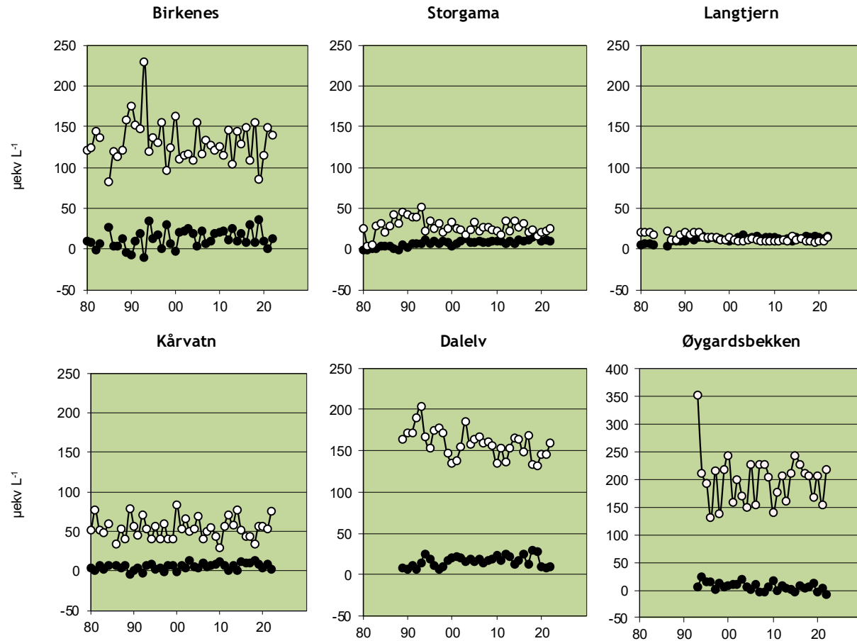
Figur 23. Volumveid konsentrasjoner av klorid (Cl) og ikke-marint natrium ( \text{Na}^* ) ved feltforskningsstasjonene for perioden 1980-2022. \text{Na}^* ● og Cl ○. Enhet: \mu\text{ekv L}^{-1} . NB! Annen skala på y-aksen for Øygardsbekken.
