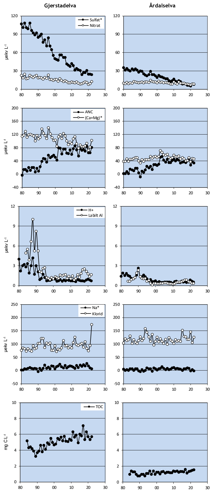
Figur 25. Årsmiddelerverdi av utvalgte parametere for Gjerstadelva og Årdalselva for perioden 1980-2022.
