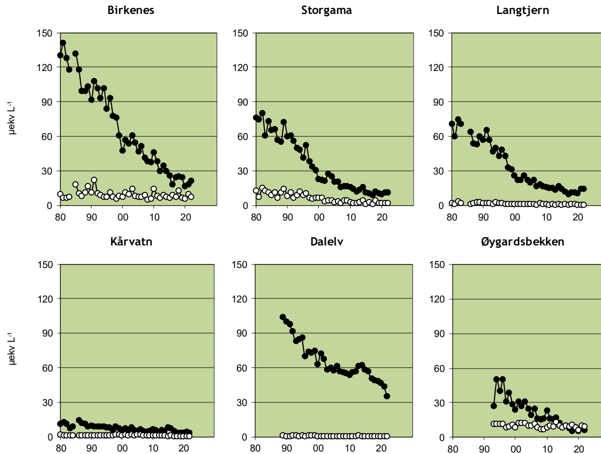
Figur 20. Volumveide konsentrasjoner av nitrat ( \text{NO}_3 ) og ikke-marint sulfat ( \text{SO}_4^* ) ved feltforskningsstasjonene for perioden 1980-2022. \text{SO}_4^* ● og \text{NO}_3 ○. Enhet: \mu\text{ekv L}^{-1} .
