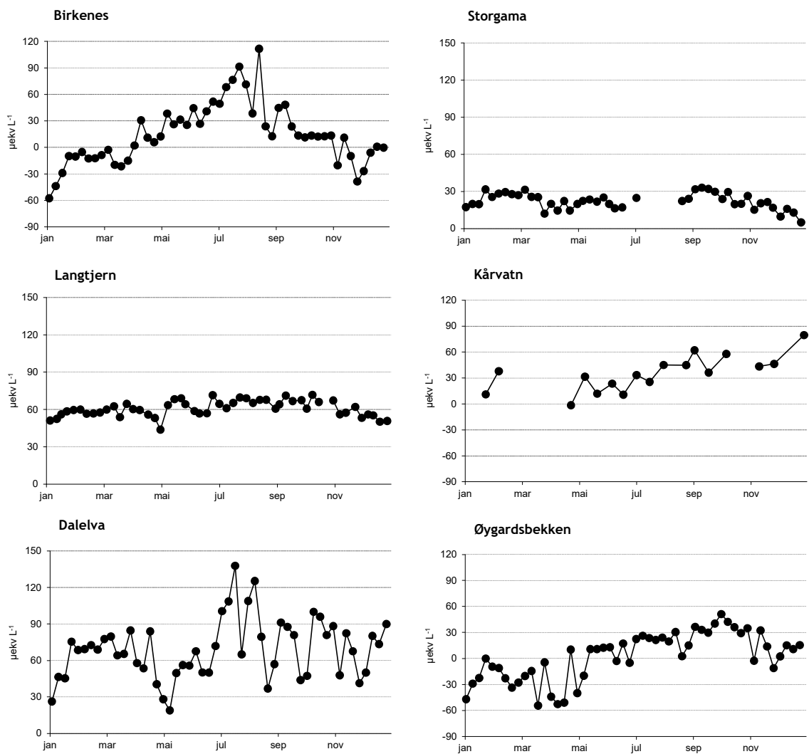
Figur 17. Sesongmessig fluktusjoner i konsentrasjonene av syrenøytraliserende kapasitet (ANC) ved feltforskningsstasjonene i 2022. Enhet: \mu\text{ekv L}^{-1} . NB! Ulik skala på y-aksene.
