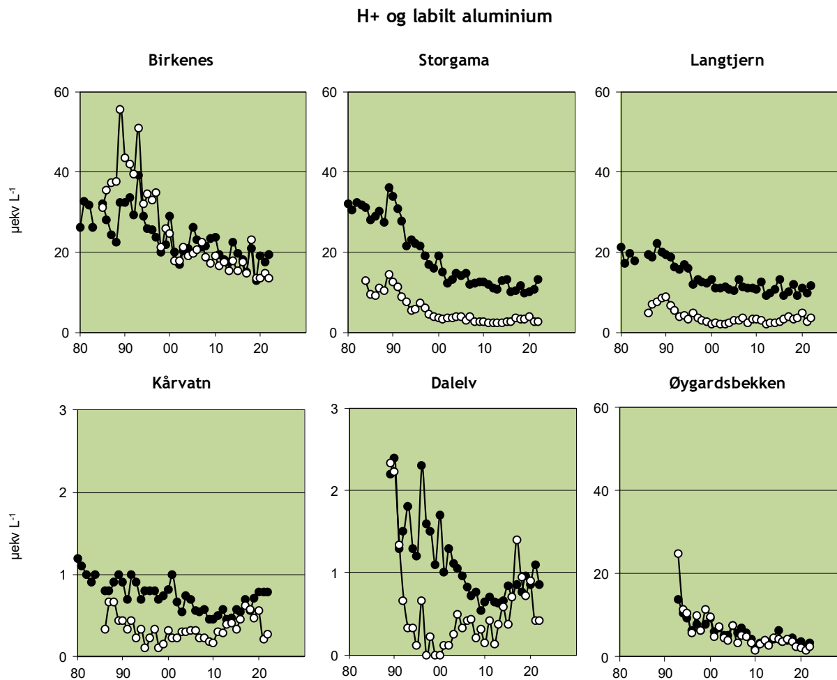
Figur 22. Volumveide konsentrasjoner av hydronium ioner (H + ) og labilt aluminium (LAI) ved feltforskningsstasjonene for perioden 1980-2022. H + ● og labilt Al ○. Enhet: µekv L -1 . NB! Annen inndeling på y-aksen for Kårvatn og Dalelv.
