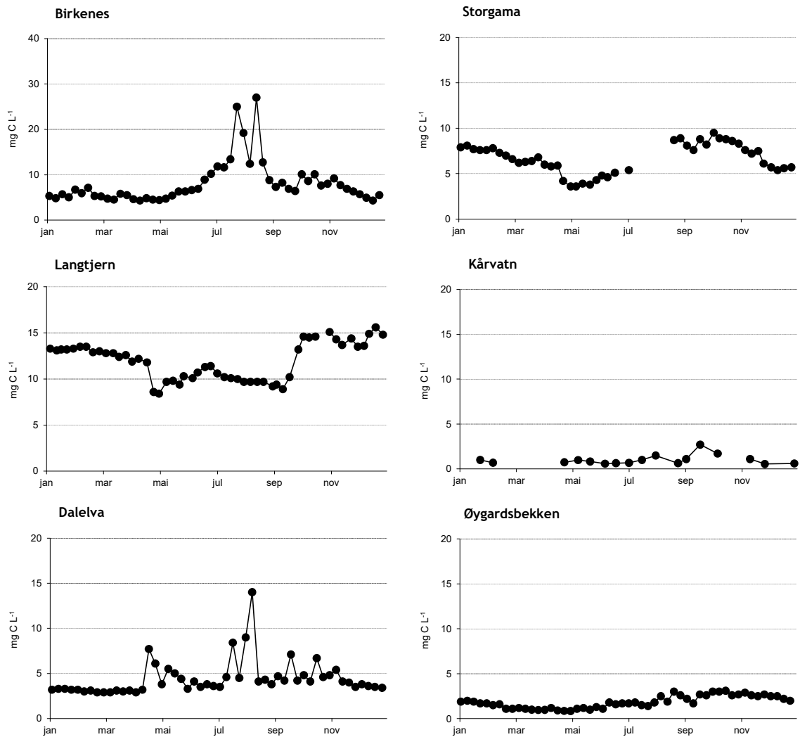
Figur 18. Sesongmessig fluktusjoner i konsentrasjonene av total organisk karbon (TOC) ved feltforskningsstasjonene i 2022. Enhet: mg C L -1 . NB! Annen skala på y-aksen for Birkenes.
