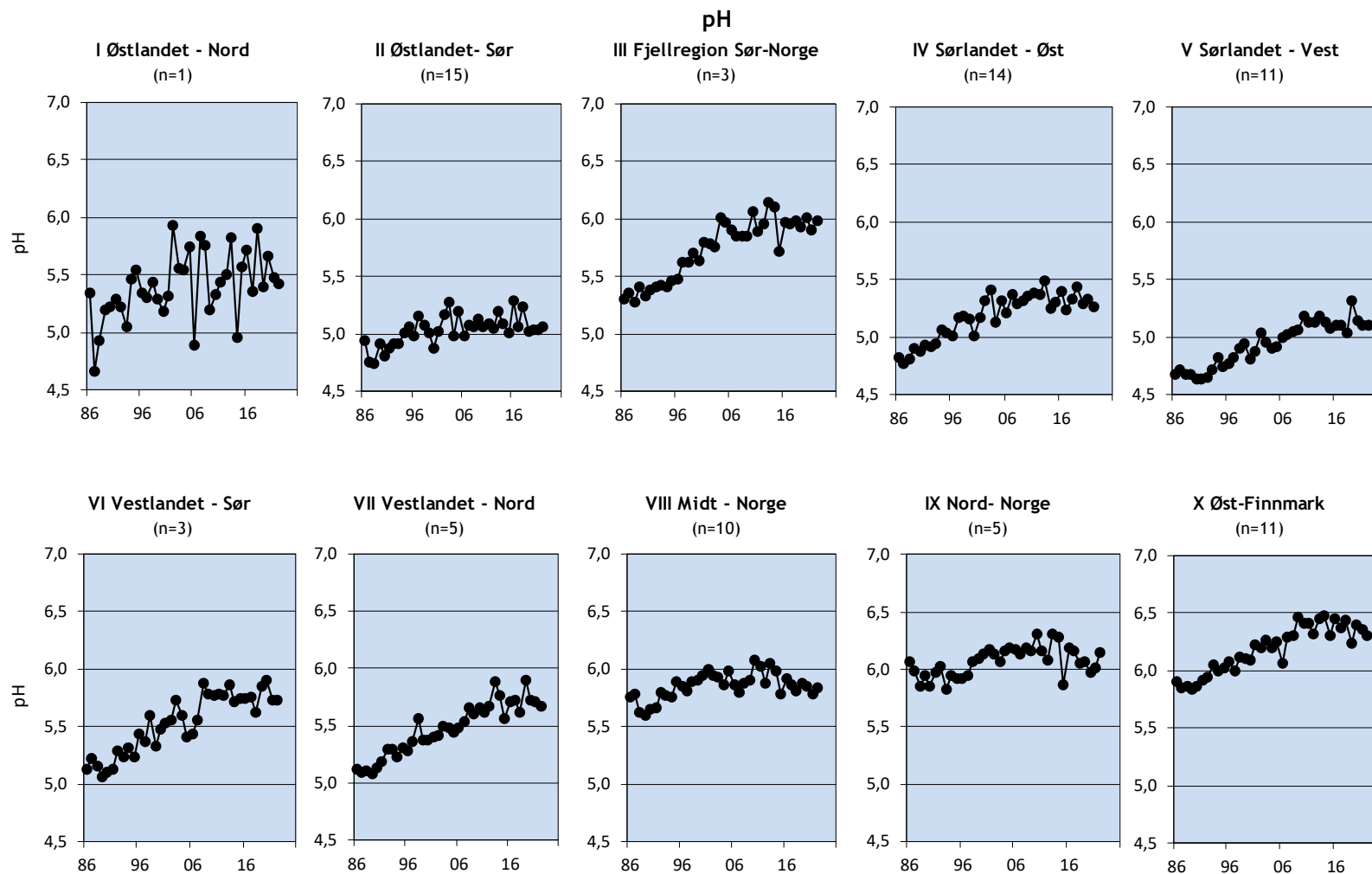
Figur 8. Årlige gjennomsnitt av pH (via H^+ ekv L^{-1} ) i de forsurningsfølsomme innsjøene for perioden 1986-2022 fra hver av de 10 regionene beskrevet i Vedlegg 1. n angir antall innsjøer i hver region.
