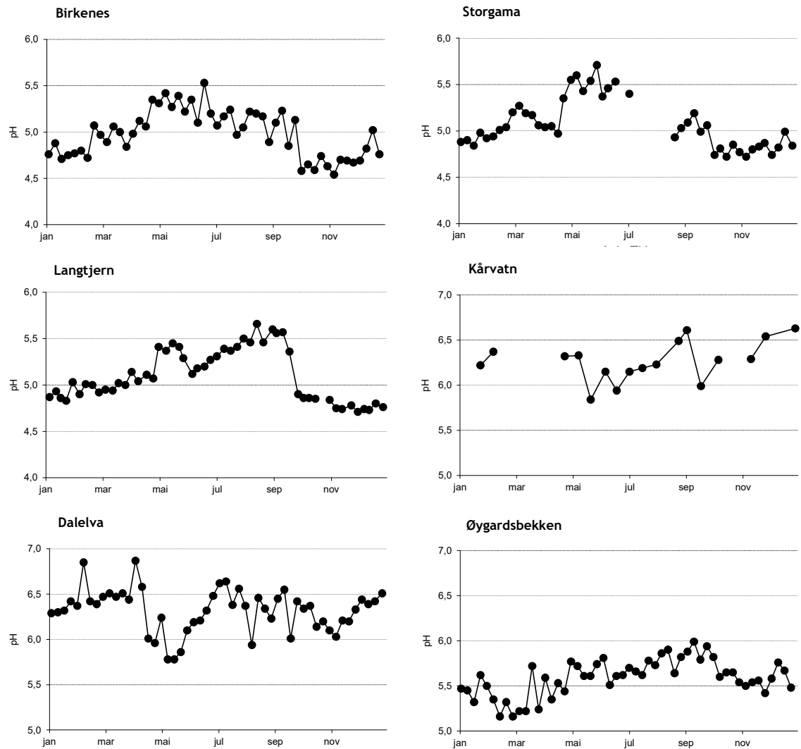
Figur 14. Sesongmessig fluktusjoner i pH ved feltforskningsstasjonene i 2022. NB! Ulik skala på y-aksene.
