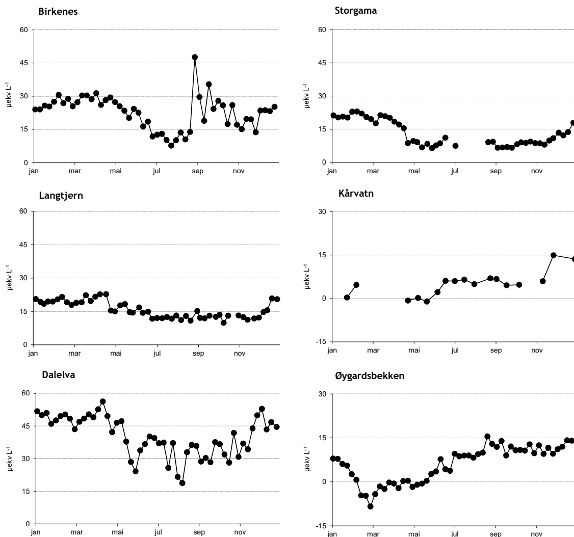
Figur 13. Sesongmessig fluktusjoner i konsentrasjonene av ikke-marint sulfat ( \text{SO}_4^* ) ved feltforskningsstasjonene i 2022. Enhet: \mu\text{ekv L}^{-1} . NB! Ulik skala på y-aksene.
