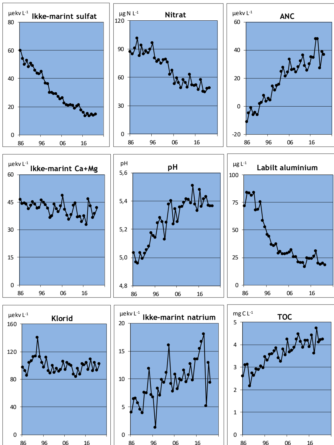
Figur 3. Årlige gjennomsnittskonsentrasjoner fra 1986 til 2022 av et utvalg av parametere i 78 forureningsfølsomme innsjøer fordelt over hele landet.
