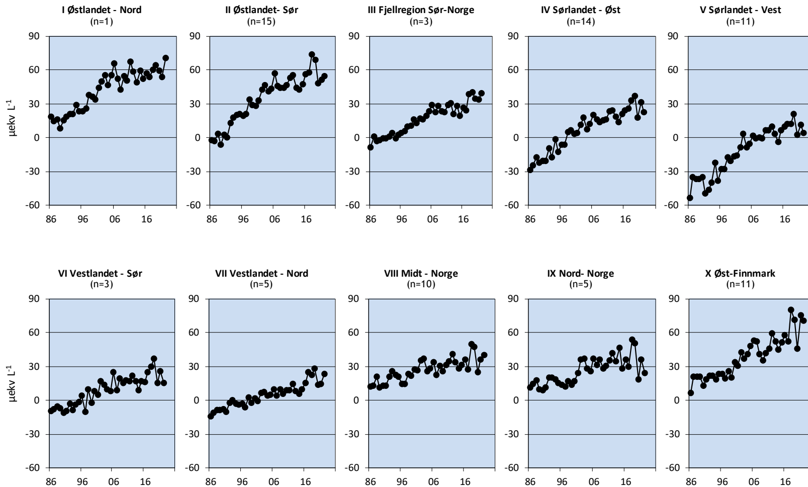
Figur 6. Årlige gjennomsnittsverdier av syrenøytraliserende kapasitet (ANC) i de forsurningsfølsomme innsjøene for perioden 1986-2022 fra hver av de 10 regionene beskrevet i Vedlegg 1. Enhet: \mu\text{ekv L}^{-1} . n angir antall innsjøer i hver region.
