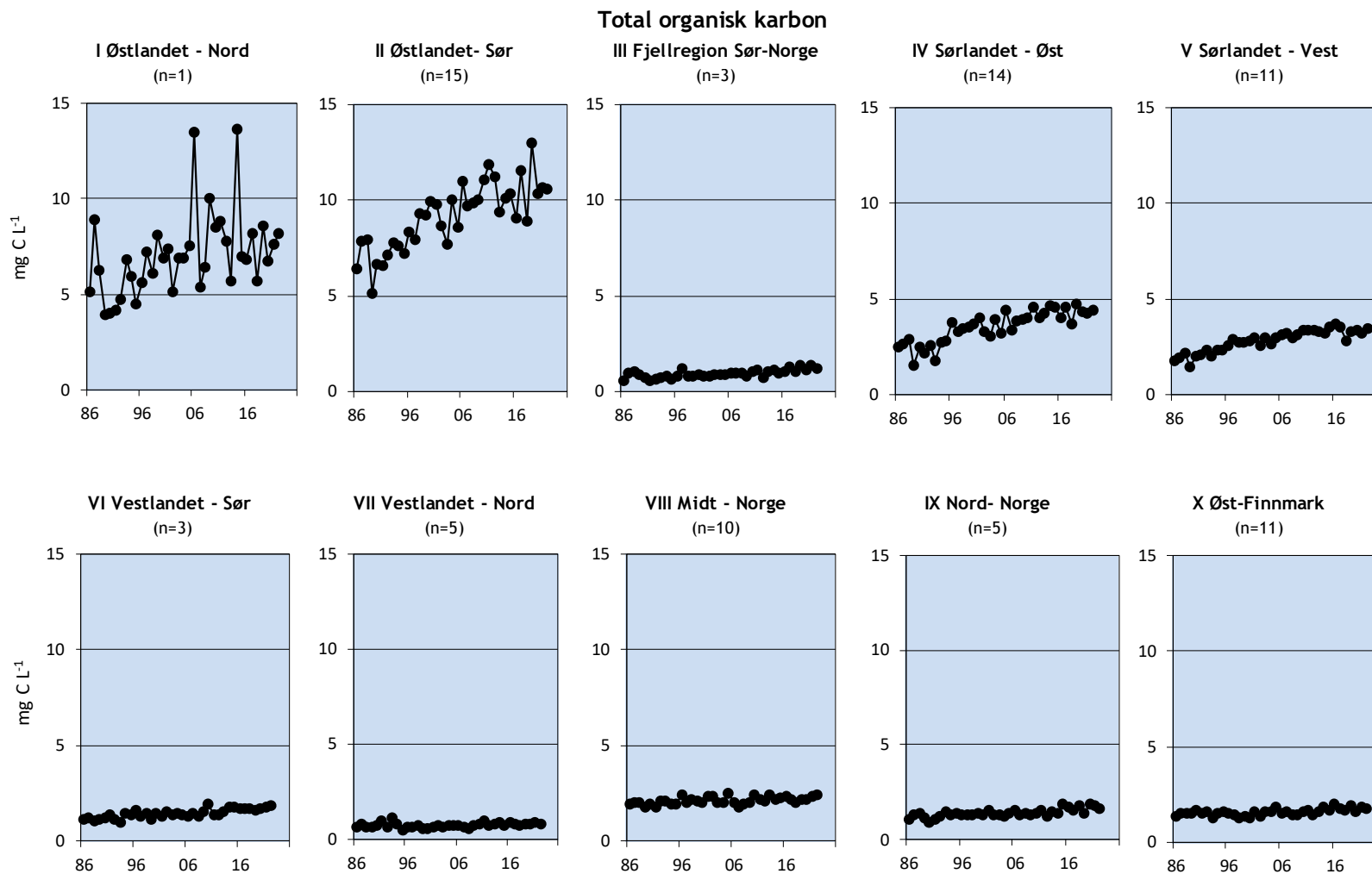
Figur 10. Årlige gjennomsnittskonsentrasjoner av total organisk karbon (TOC) i de forsureningsfølsomme innsjøene for perioden 1986-2022 fra hver av de 10 regionene beskrevet i Vedlegg 1. Enhet: mg C L -1 . n angir antall innsjøer i hver region.
